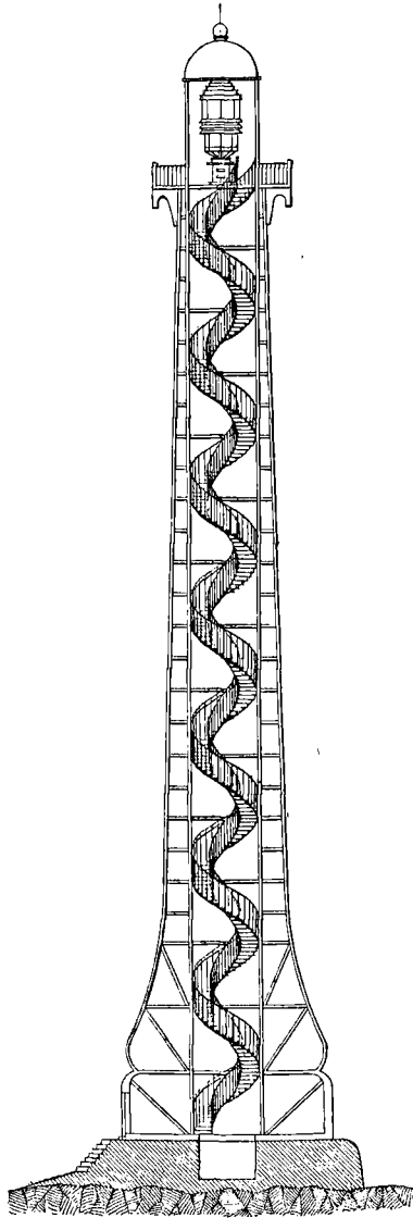
Phare métallique des Roches-Douvres (au nord de la Bretagne). Symétrie hélicoïde parfaite.
