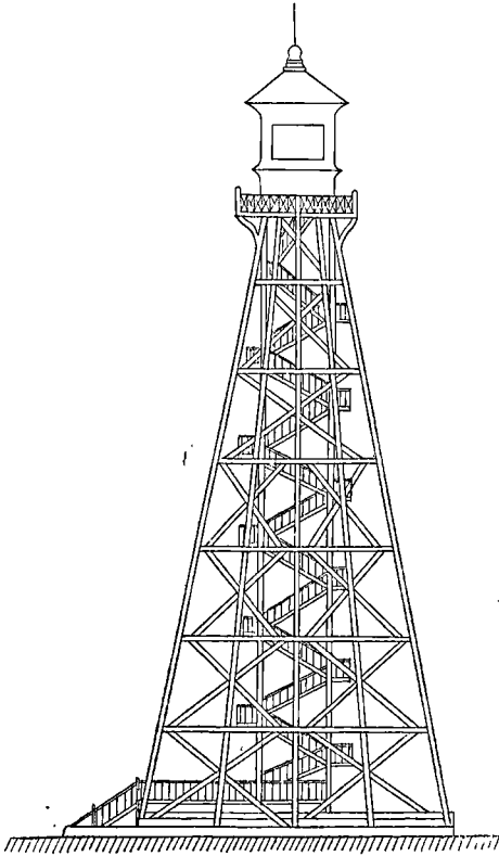
Phare en charpente de Pontailac (près de l'embouchure de la Gironde). Disposition hélicoïde de l'escalier, non isotrope autour de l'axe vertical. Paliers et rampes alternants.
