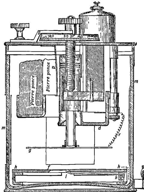
Électromètre portatif, forme actuelle : \frac{2}{3} de la grandeur.
