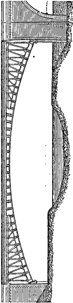
Pont avec un seul système de diagonales symétriques.
