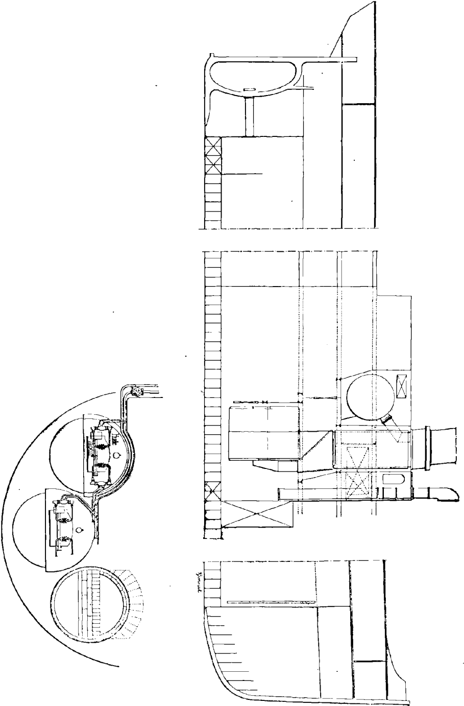
Fig. 55. — Coupe d'un bateau-réservoir, système Fortescue Plannery et Boyd.
