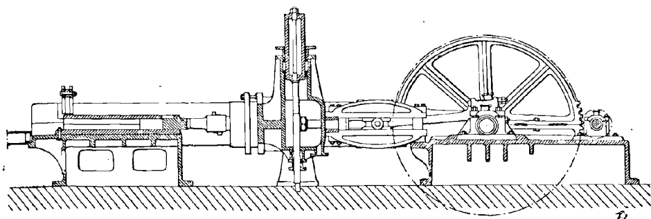
FIG. 136. — Presse Bourriez.
