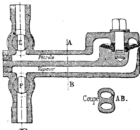
FIG. 73. — Brûleur Artenef.
