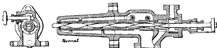
FIG. 114. — Appareil Kermode.
