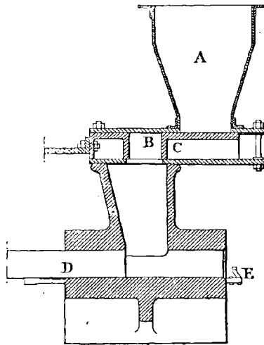
FIG. 134. — Presse de la Compagnie Paris-Lyon-Méditerranée.
