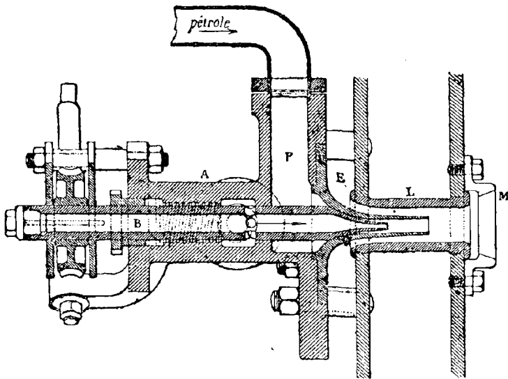
FIG. 65. — Autre appareil Urquardt.
