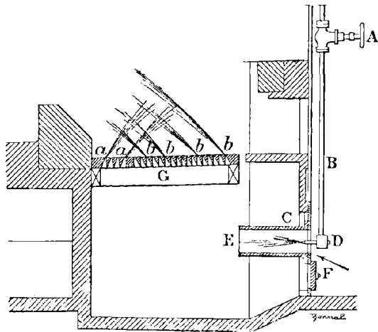
FIG. 42. — Grille Poillon.
