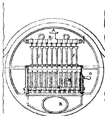
FIG. 79. — Foyer à pétrole des Forges et Chantiers de la Méditerranée.
