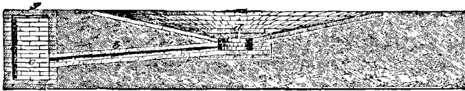
FIG. 132. — Aire en maçonnerie pour meule verticale.
