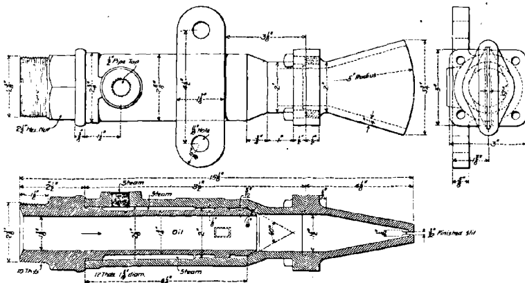
FIG. 94, 95, 96. — Brûleur Lundholm.
