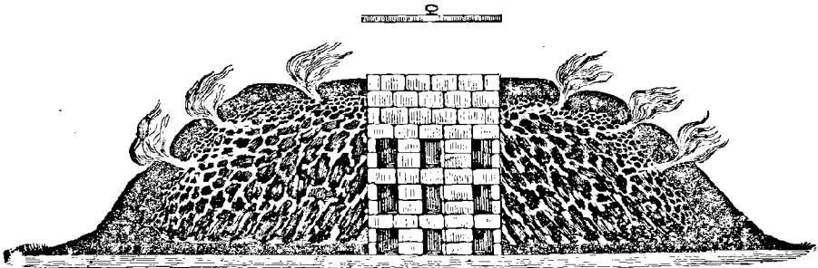
FIG. 160. — Meule pour la carbonisation de la houille.
