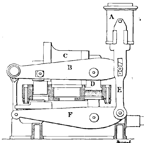
FIG. 149. — Presse Biérix.
