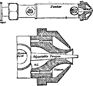
FIG. 57. — Injecteur à pétrole de l'Hydroleum Fuel Co.
