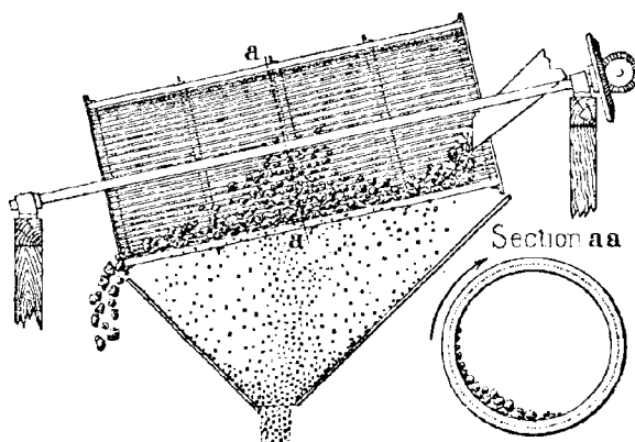
FIG. 11. — Trommel simple à axe incliné.
