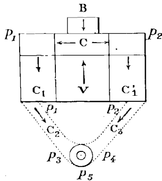
FIG. 129. — Schéma d'une installation faite à la Réunion pour brûler la bagasse.
