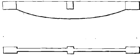
FIG. 123. — Barreaux de grille pour sciure de bois.
