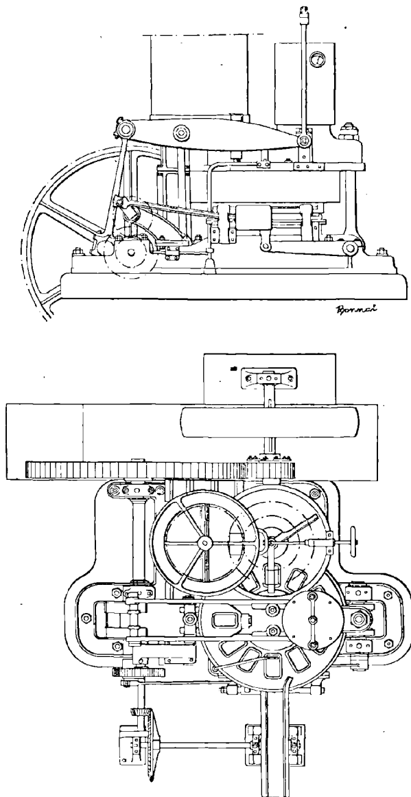
FIG. 131 et 132. — Presse Crozet.
