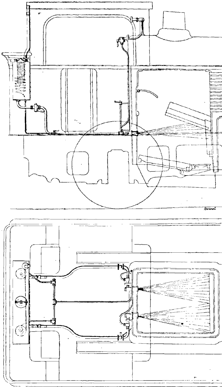
FIG. 84. — Application à une locomotive d'un appareil Vétillard Scherdin.
