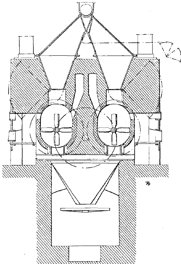
FIG. 139. — Four Marsais.
