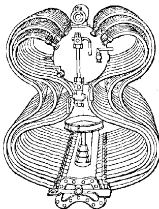
FIG. 418. — Chaudière au pétrole lampant.
