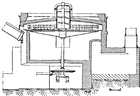
FIG. 140. — Four Biérix.
