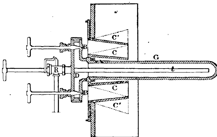
FIG. 419. — Brûleur Rosier.
