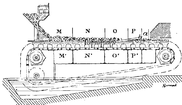
FIG. 38. — Chargeur Coxe.
