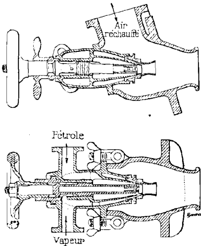
FIG. 100 et 101. — Pulvérisateur double d'Allest.
