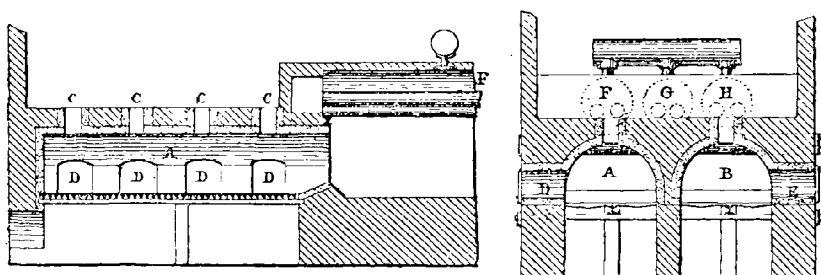
FIG. 121 et 122. — Foyer Hoyt pour l'emploi de la tourbe.
