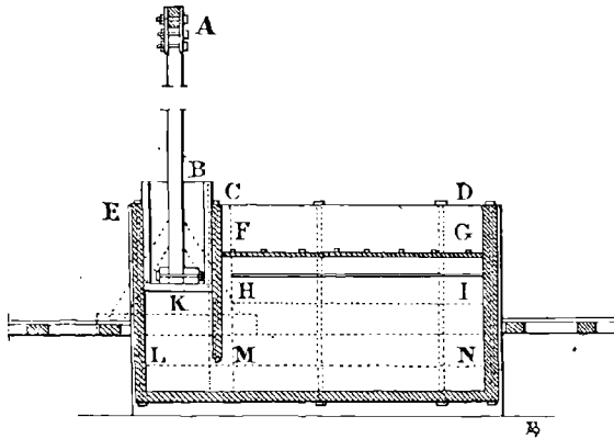
FIG. 28. — Laveur Lacretelle.
