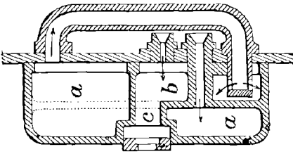
FIG. 81. — Boîte de mélange de l'appareil Santenard.
