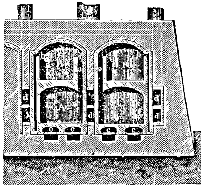
FIG. 171. — Four à coke système Fromont.
