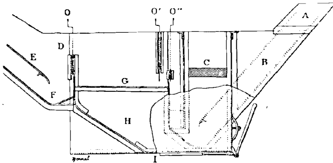
FIG. 30. — Laveur Bérard.
