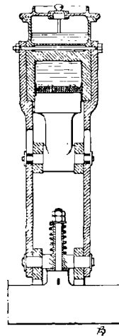
FIG. 145. — Appareil de moulage de la presse Dupuy.
