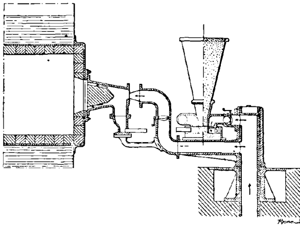
FIG. 47. — Appareil Friedeberg.
