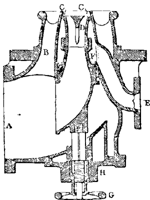
FIG. 111. — Pulvérisateur d'Allest à air soufflé.
