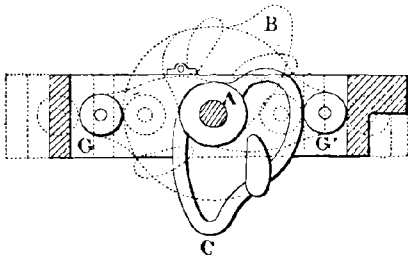
Fig. 144. — Détail de la came de commande dans la presse Durand et Marais.
