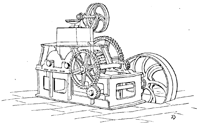
FIG. 157. — Presse Zimmermann-Hanrez.
