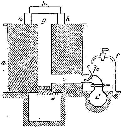
FIG. 62. — Foyer à pétrole pour forge.
