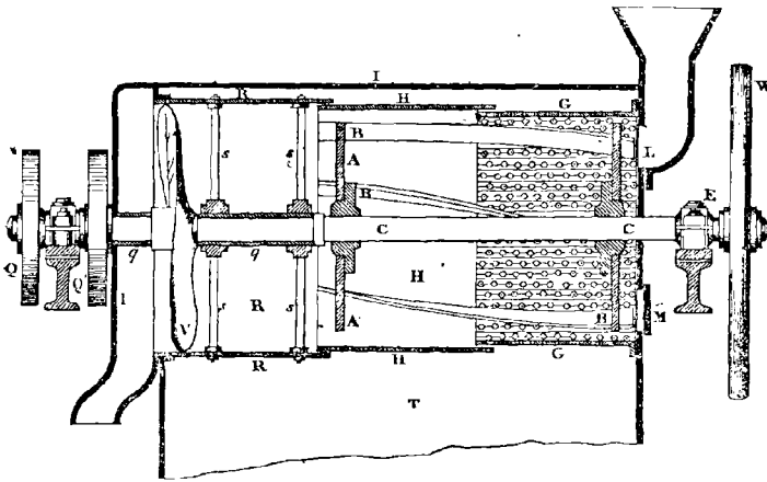
FIG. 22. — Broyeur-épurateur Sottiaux.
