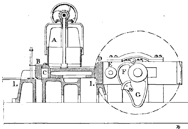
FIG. 143. — Presse Durand et Marais.
