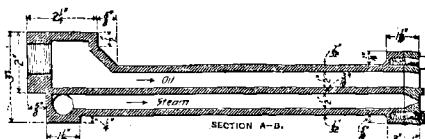
FIG. 89. — Brûleur Booth.
