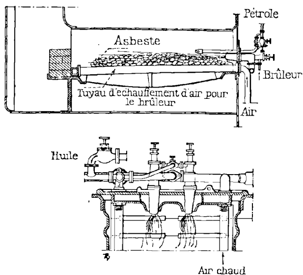
FIG. 115 et 116. — Application d'un appareil Kermode à un foyer.
