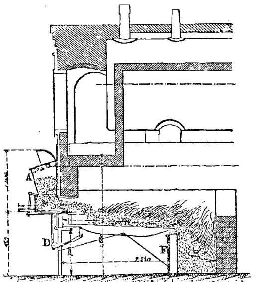
FIG. 39. — Appareil Proctor.
