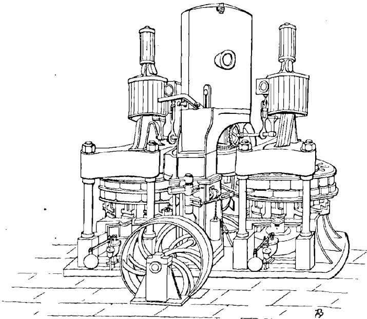
FIG. 146. — Presse Mazeline.
