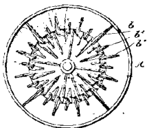
FIG. 52. — Broyeur pour le foyer de l'Ideal Fuel Feeder Co.
