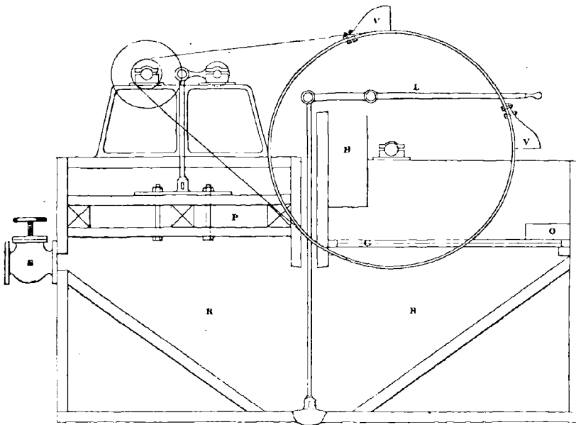
FIG. 32. — Laveur Lührig-Coppéc.
