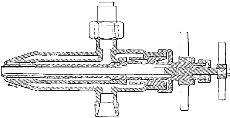
Fig. 110. — Brûleur Rusden et Eeles.
