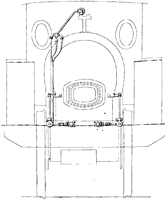
FIG. 83. — Application à un foyer de locomotive d'un appareil Vétillard Scherding.
