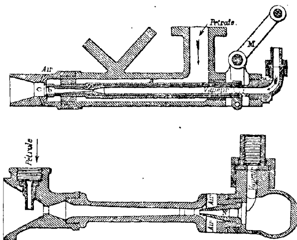
FIG. 104 et 105. — Pulvérisateur Kœrting.
