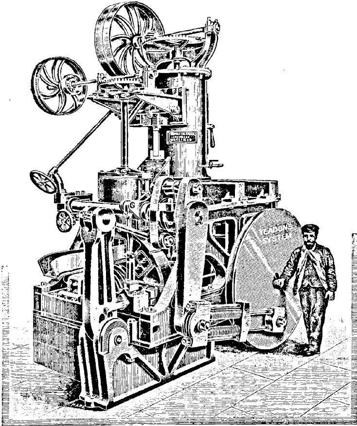
FIG. 148. — Presse Yeadon.
