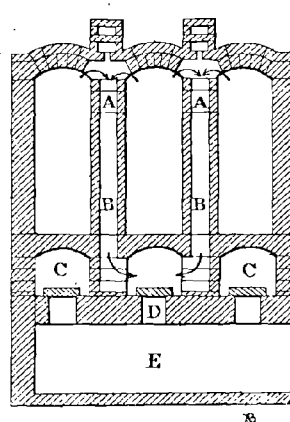
FIG. 172. — Four à coke système Coppée.
