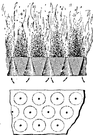
FIG. 43. — Grille Kudlicz.
