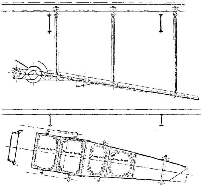
FIG. 6. — Table à secousse (Élévation et plan).
