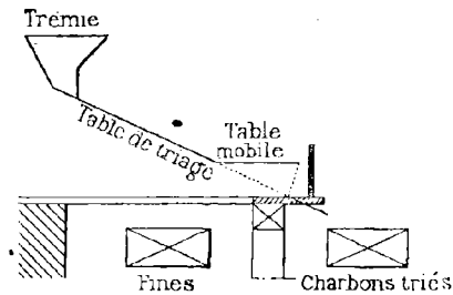
FIG. 17. — Triage sur table mobile.
