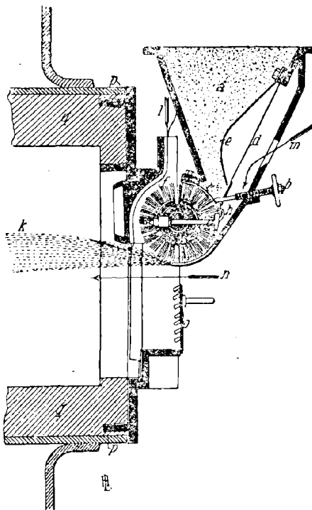
FIG. 48. — Appareil Schwarzkopf.
