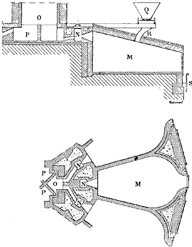
FIG. 163 et 166. -- Four à ruche Eaton.
