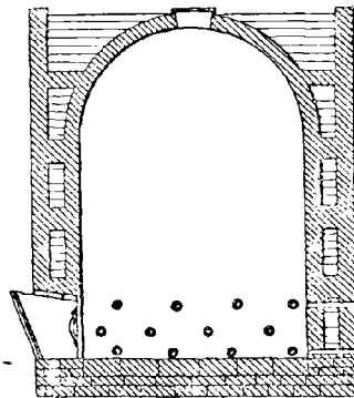
FIG. 123. — Four d'Oberndorf.
