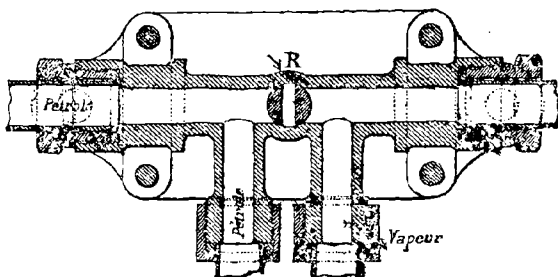
FIG. 74. — Brûleur Artenef.
