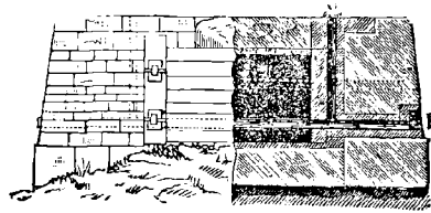
FIG. 161. — Four Schaumburg. (Coupe transversale.)
