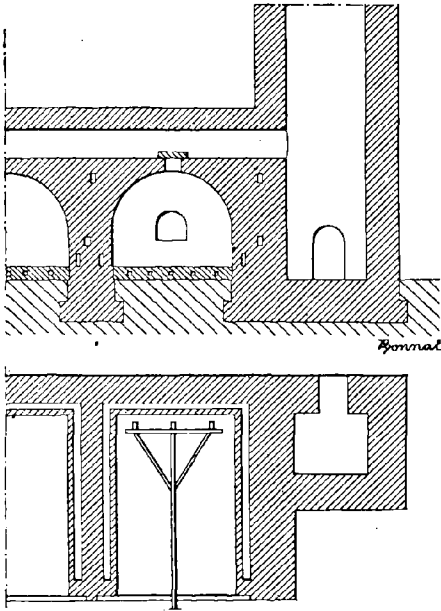
FIG. 167 et 168. — Fours à coke Gibson.
