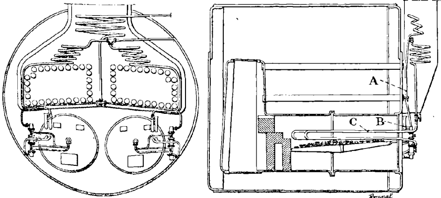
FIG. 107. — Disposition du brûleur Orde sur un foyer.
