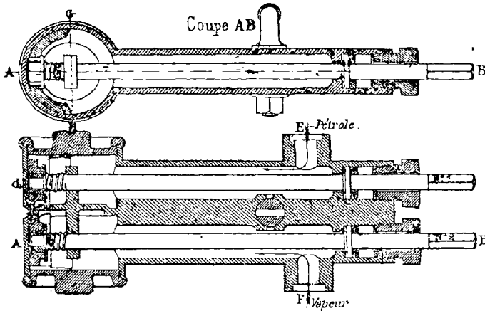
Fig. 76. — Appareil Lenz.
