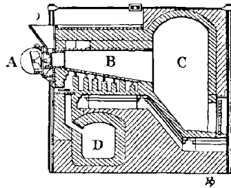
FIG. 182. — Four à coke système Lürmann.
