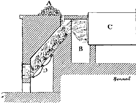
FIG. 127. — Foyer à bagasse système Fryer.
