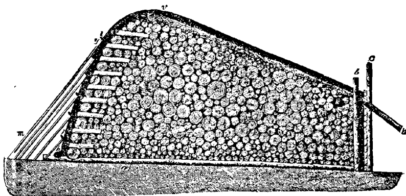
FIG. 131. — Meule horizontale pour la carbonisation du bois.
