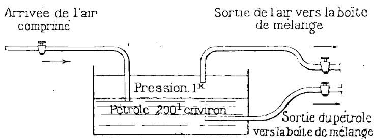
FIG. 80. — Appareil Santenard.
