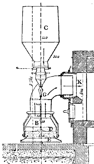
FIG. 46. — Appareil Wegener.
