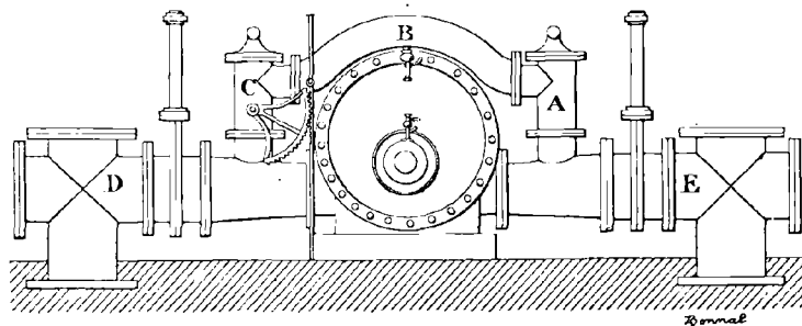
FIG. 184. — Extracteur Beale.
