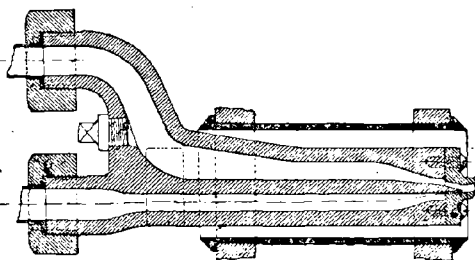
FIG. 72. — Pulvérisateur Fvardofski.
