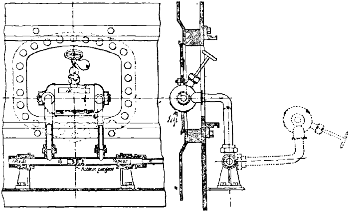
FIG. 69. — Disposition d'ensemble du foyer Karapetof.
