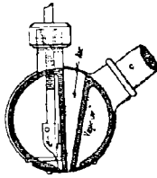
FIG. 67 et 68. — Brûleur Karapetof.
