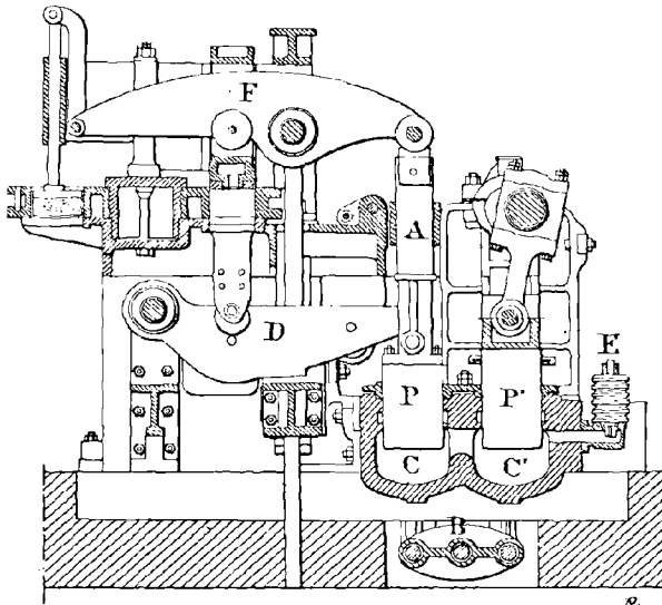
FIG. 133. — Presse Roux-Veillon.
