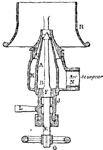
FIG. 98. — Pulvérisateur d'Allest.
