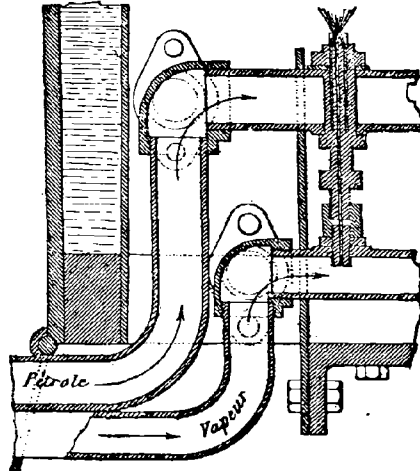
FIG. 64. — Appareil Urqhardt.
