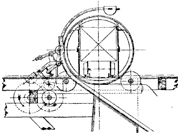
FIG. 3. — Appareil verseur circulaire.
