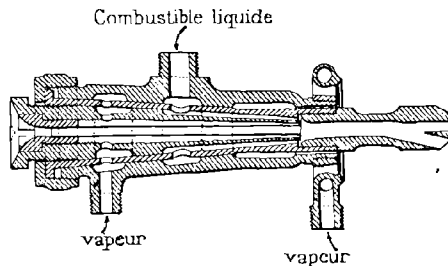
FIG. 86. — Injecteur Holden.
