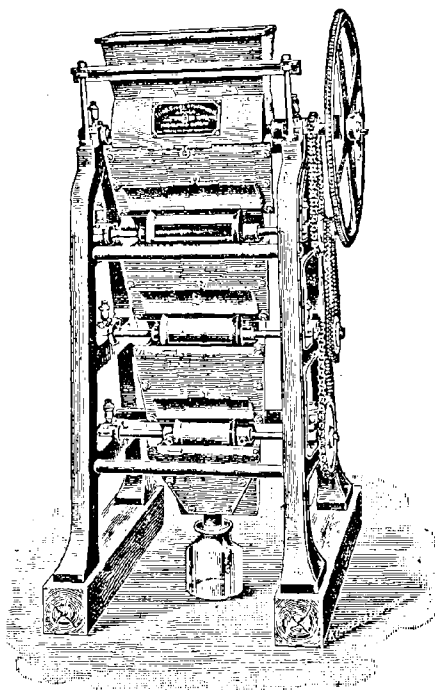
FIG. 1. — Appareil de prise d'essai mécanique des échantillons d'analyse.
