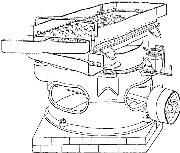
FIG. 8. — Crible Coxe.
