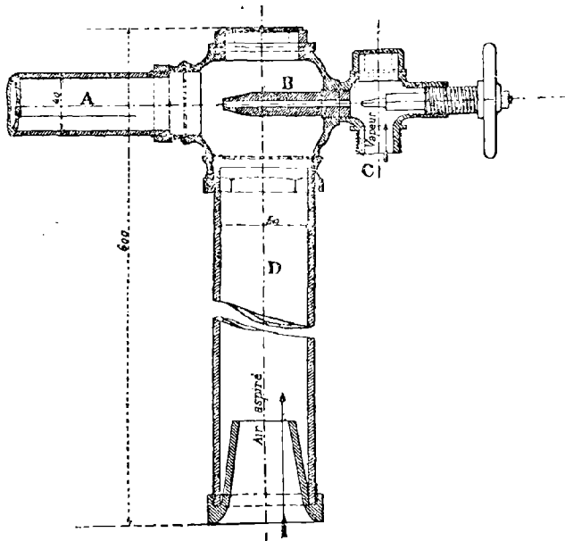
FIG. 41. — Appareil Orvis.
