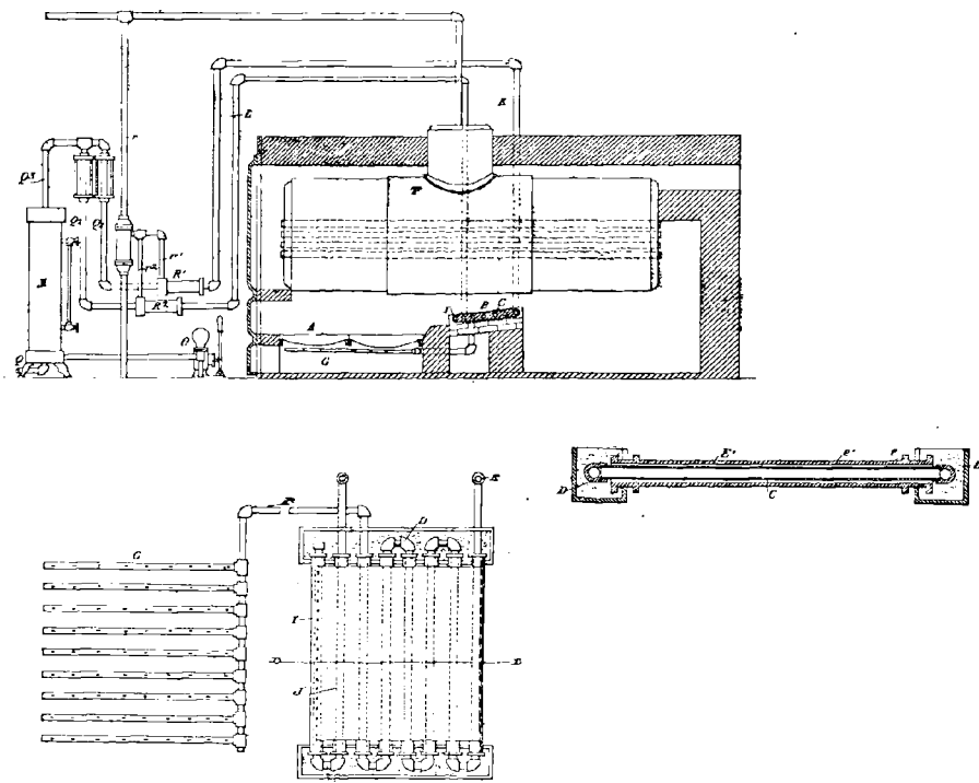
FIG. 59, 60, 61. — Foyer au pétrole de l'Economy Manufacturing Co.
