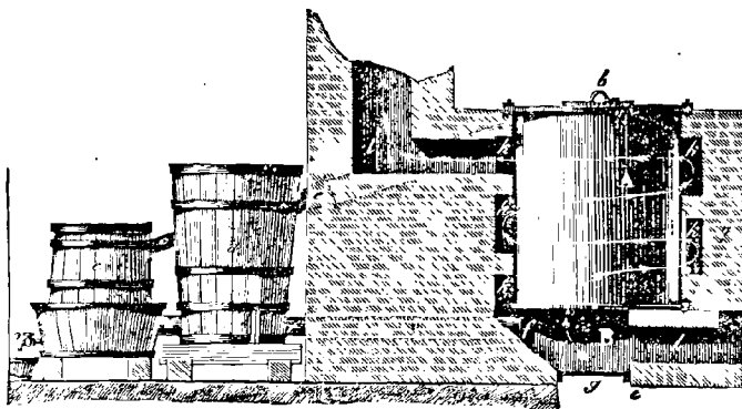
FIG. 135. — Four de carbonisation avec récupération des sous-produits.
