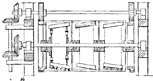
FIG. 13. — Trommel avec brosses de nettoyage des surfaces.
