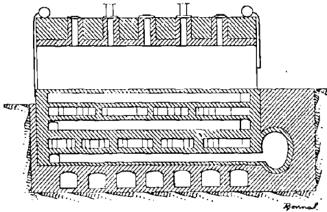
FIG. 181. — Four système Festner-Hoffmann.
