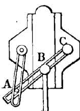
FIG. 27. — Coulisse différentielle d'un bac à piston.
