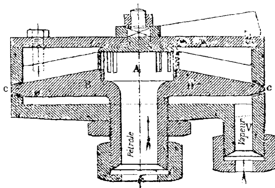
FIG. 70. — Brûleur Brandt.
