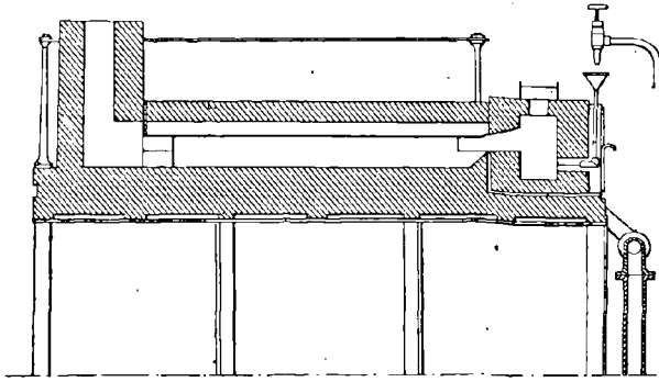
Fig. 63. — Foyer de forge à résidus de pétrole.
