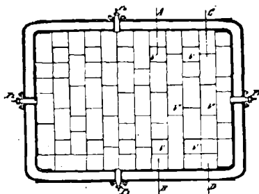
FIG. 71. — Sote du foyer Fvardofski.
