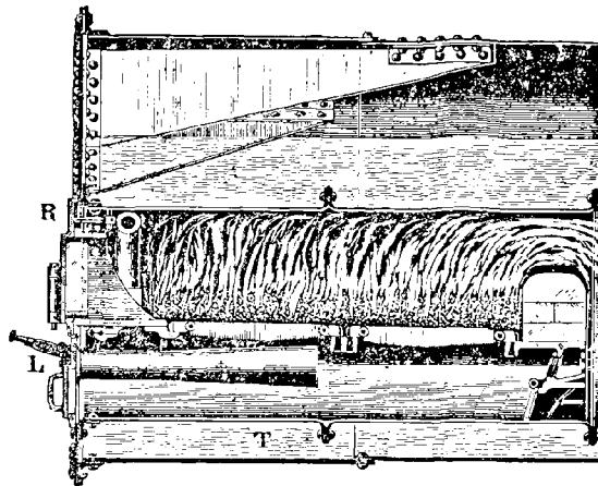
FIG. 45. — Foyer Meldrum.
