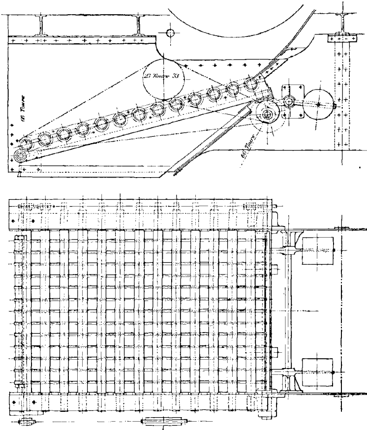
FIG. 5. — Grille mobile des mines de Béthune.
