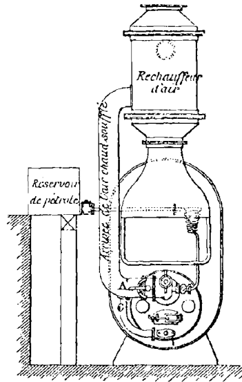
FIG. 112. — Installation d'un pulvérisateur à air soufflé système d'Allest.
