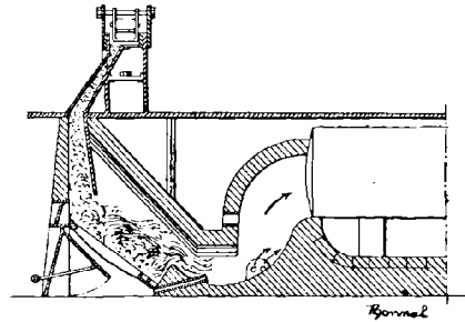
FIG. 128. — Foyer à bagasse système Price Abell.
