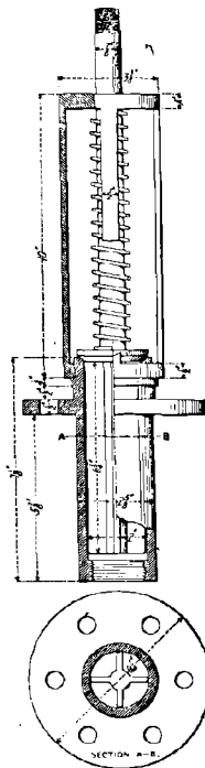
FIG. 90. — Sonpape de sûreté Booth.
