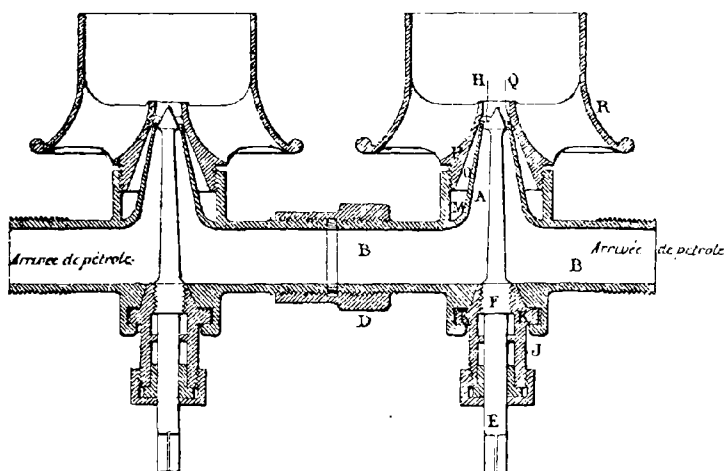
FIG. 99. — Pulvérisateurs d'Allest accouplés.
