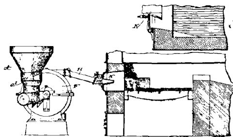
FIG. 53. — Foyer de l'Ideal Fuel Feeder Co.
