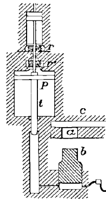
FIG. 147. — Pot de presse de la machine Mazeline.
