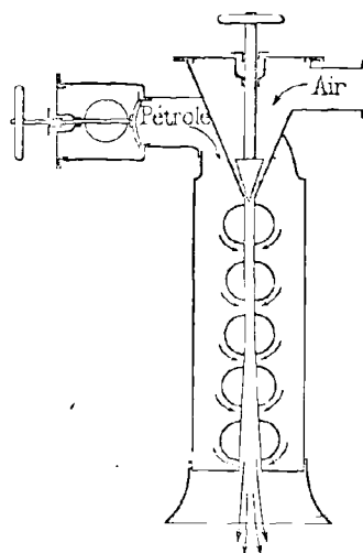
FIG. 113. — Pulvérisateur Fontaine.
