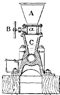
FIG. 153. — Machine à agglomérer de la Compagnie P.-L.-M.
