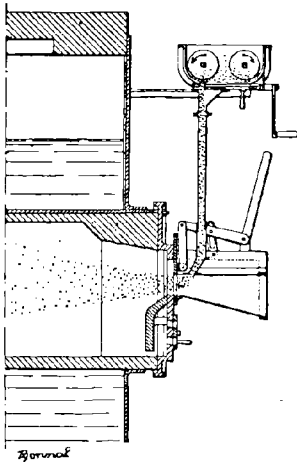
FIG. 49. — Appareil Rühl.
