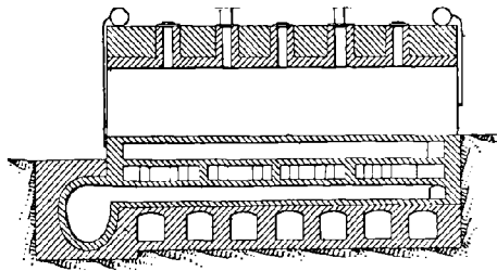
FIG. 180. — Four à coke système Festner-Hoffmann.
