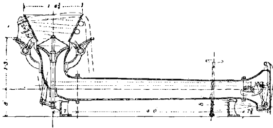
FIG. 83. — Brûleur à pétrole Clarkson.
