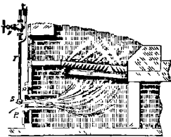
Disposition du foyer extérieur.
