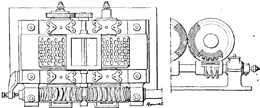
FIG. 158 et 159. — Presse Fouquemberg.
