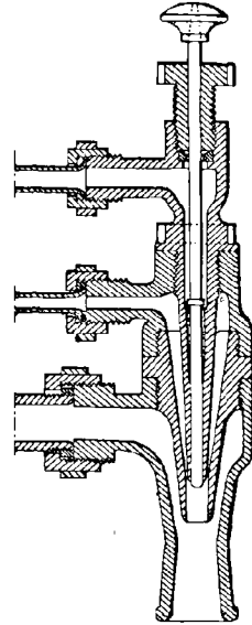
FIG. 106. — Brûleur Orde.
