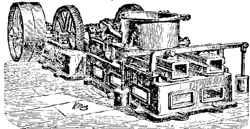
PRESSE A BRIQUETTES
