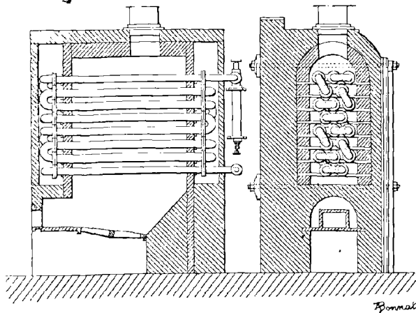
FIG. 138. — Surchauffeur de vapeur.
