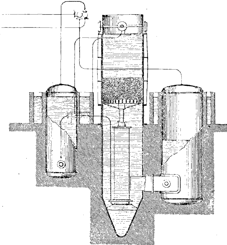
FIG. 29. — Laveur Evrard.
