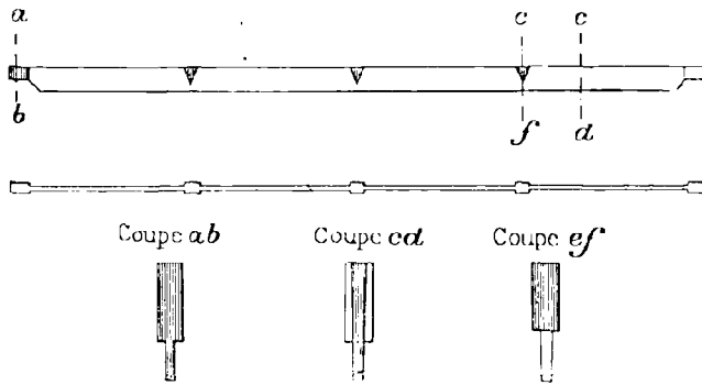
FIG. 31. — Grille du laveur Guilhaumat.
