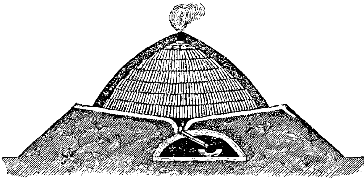
FIG. 133. — Meule russe avec trou à goudron.
