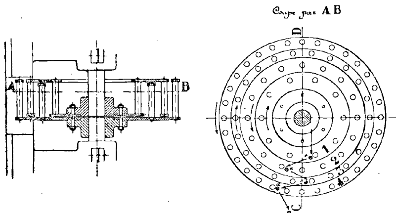
Fig. 136 et 137. — Broyeur Carr.
