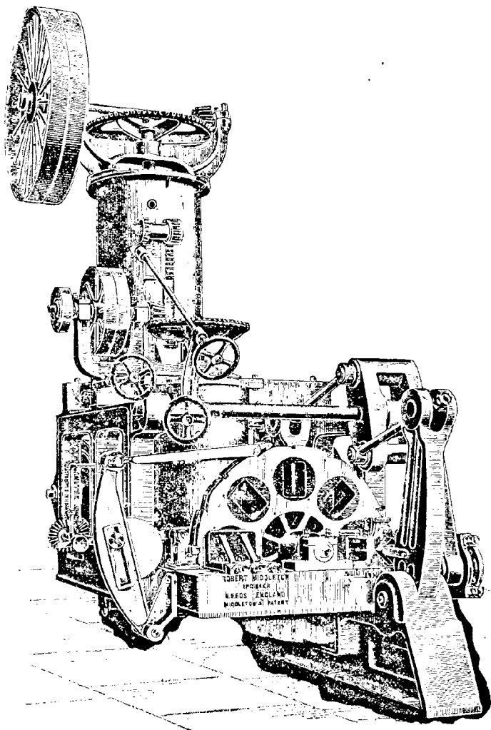
FIG. 142. — Presse Middleton.
