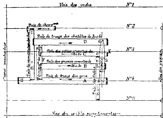
FIG. 23. — Schéma du criblage du puits Mars aux Houillères de Saint-Étienne.
