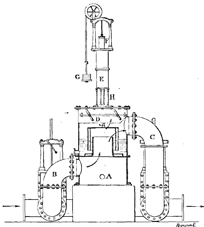
FIG. 185. — Appareil Pelouze et Audouin.
