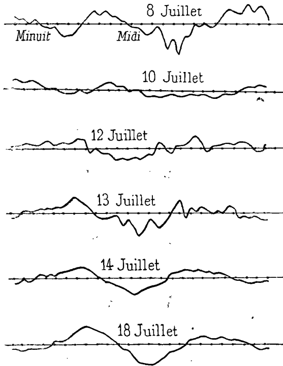
Courbes de courant tellurique fournies par un câble d'environ 1.600 milles, orienté sensiblement de l'est à l'ouest, les deux bouts du câble étant à la terre.
