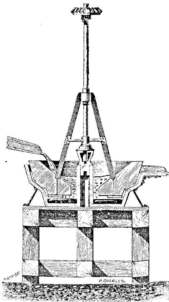
FIG. 49. — Moulin tyrolien.
