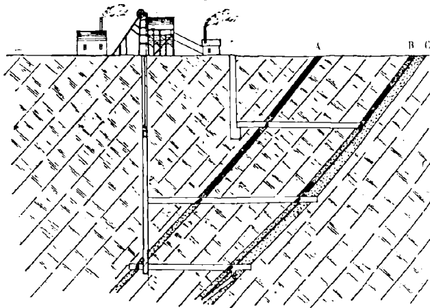
FIG. 17. — Coupe de la mine de Crown-Reef.
