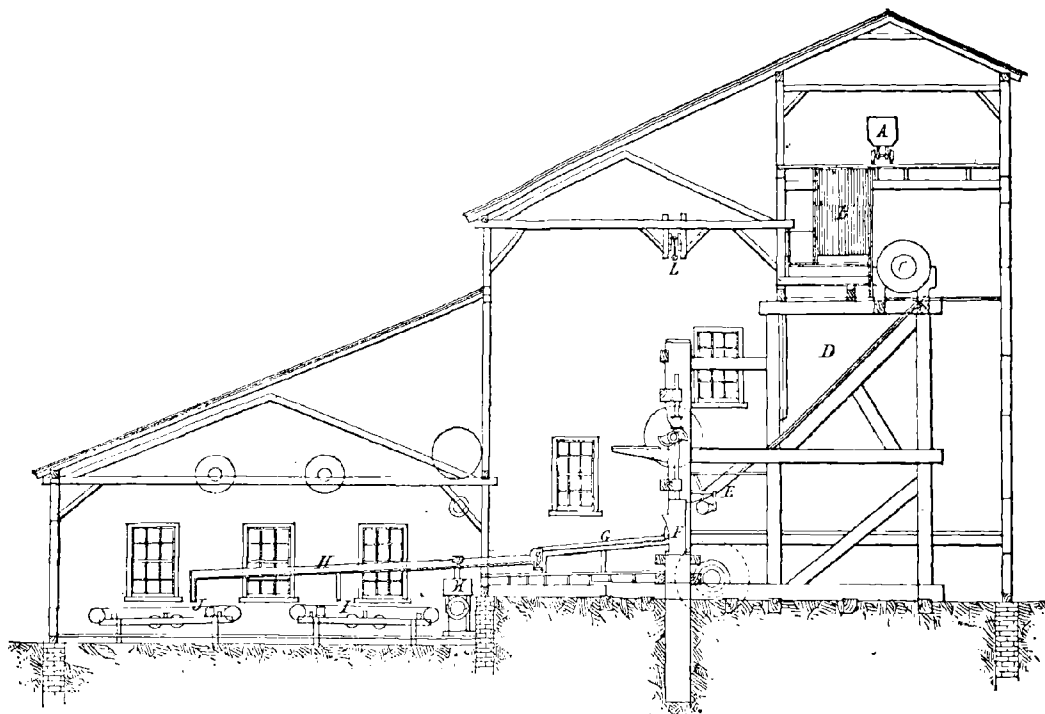
Fig. 48. — Installation d'un moulin à bocard au Witwatersrand.
