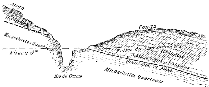
FIG. 11. — Coupe du filon de Passagem (suivant l'inclinaison du gîte) 1 .
