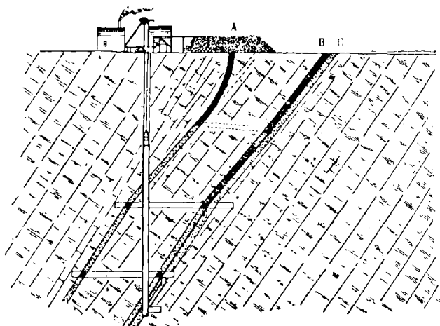
Coupe par le puits 2.
