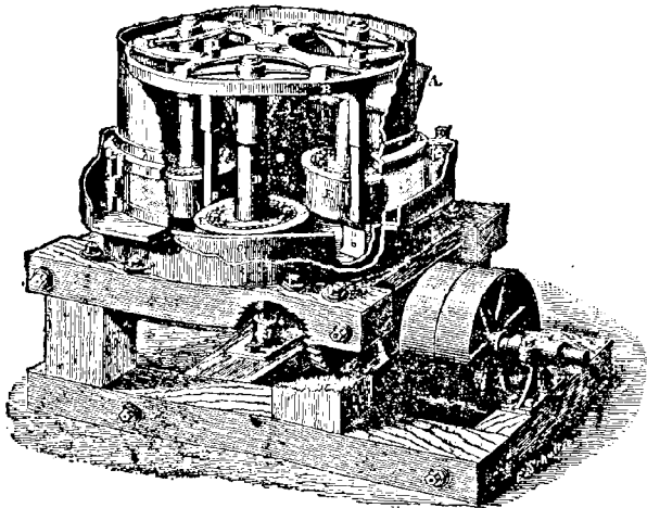
FIG. 38. — Moulin Huntington.
