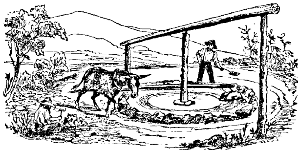
FIG. 37. — Arrastra.
