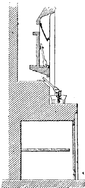
FIG. 67. — Coupe de l'appareil pour les essais d'or.
