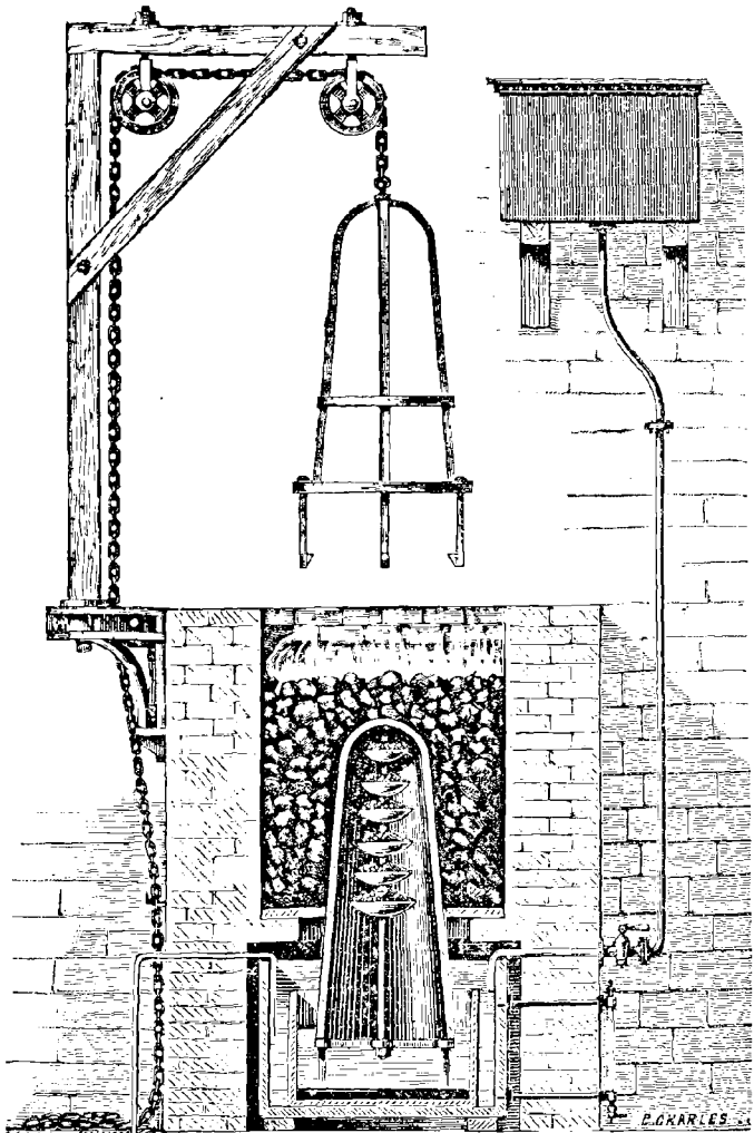
FIG. 55. — Cloche pour la distillation de l'amalgame.
