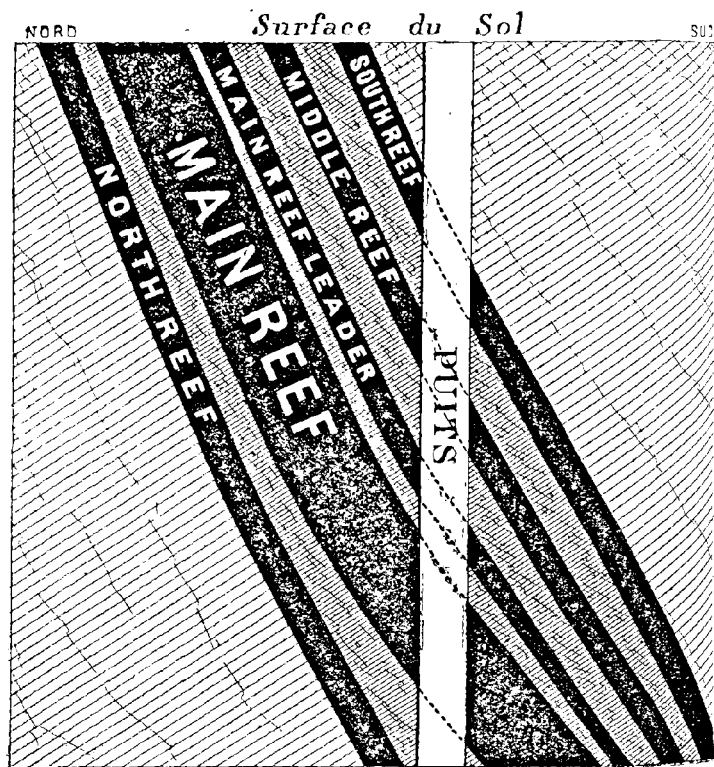
FIG. 14. Coupe théorique du Main-Reef.
