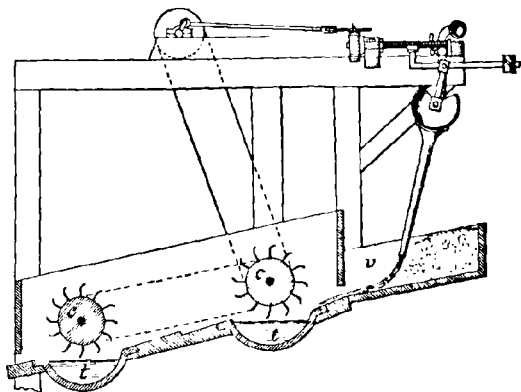
Fig. 53. — Amalgamateur Atwood.
