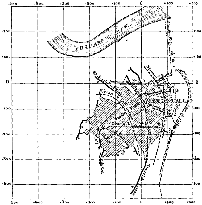
FIG. 4. — Plan horizontal de la mine de Callao en juillet 1887 (d'après de Launay).
