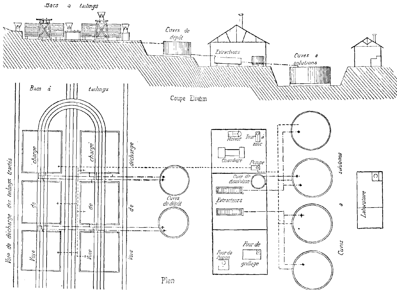
FIG. 62. — Élévation et plan schématiques d'une usine de cyanuration de Witwatersrand.
