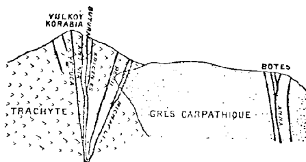
FIG. 9. — Coupe verticale Est-Ouest des filons de Vulkoy (Transylvanie).
