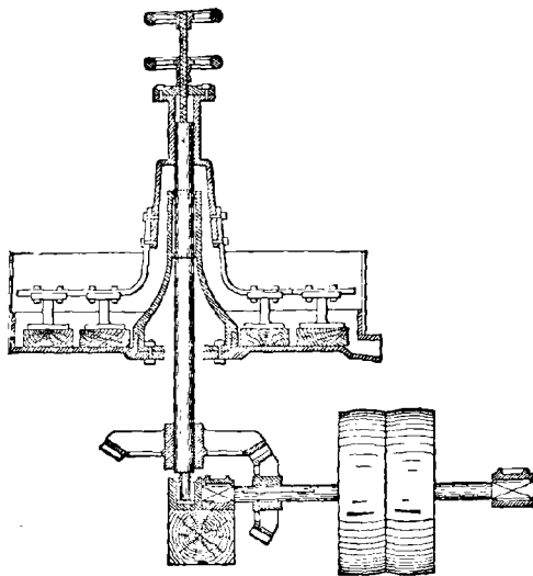
Fig. 51. — Knox-pan 1 .
