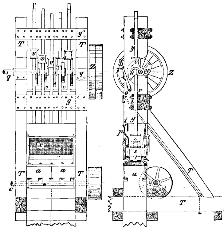
FIG. 45. — Bocard californien.
