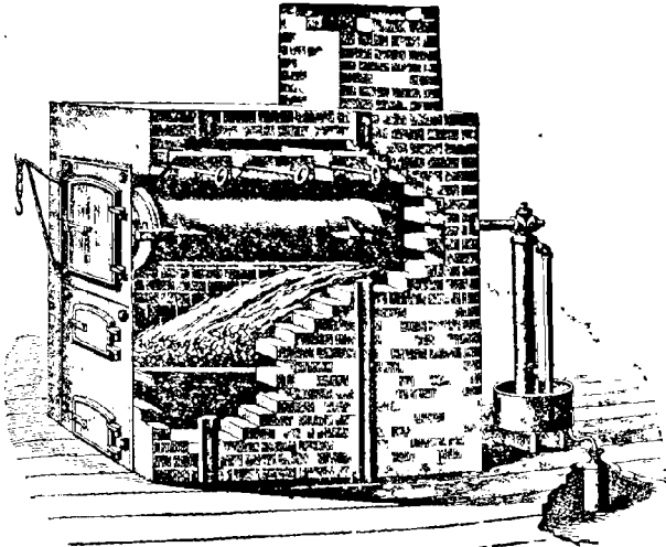
FIG. 54. — Distillation de l'amalgame 1 .
