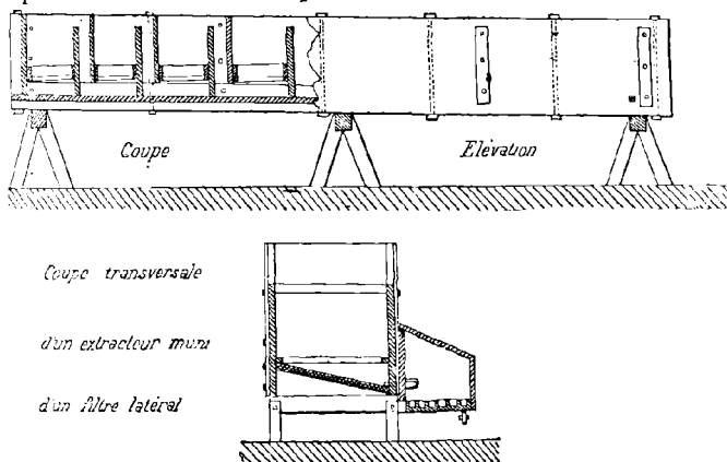
FIG. 61. — Récipient pour la précipitation de l'or 1 .
