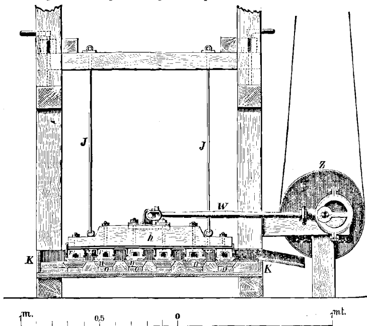
FIG. 52. — Eureka-Rubber.
