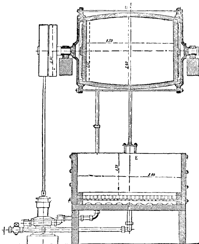
FIG. 58. — Appareil de chloruration de la mine de Passagem (Brésil) 1 .
