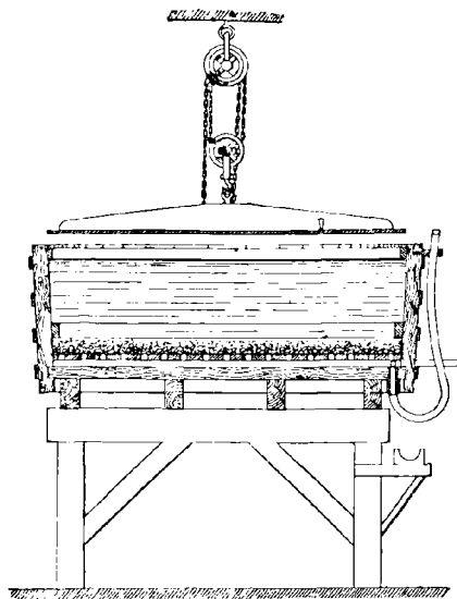
FIG. 56. — Cuve fixe 1.
