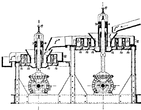
FIG. 50. — Amalgamateur Laszlo.
