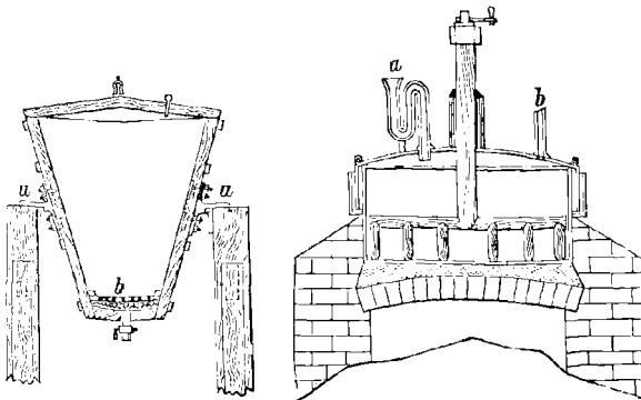
FIG. 57. — Cuve suspendue.
