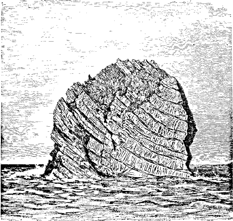
FIG. 6. — L'îlot du milieu (Rhyolites).
