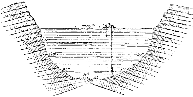
Fig. 4. — Coupe du cratère du nord-ouest au sud-est.
