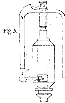
Echelle de 0 me 08 pour 1 metre.
