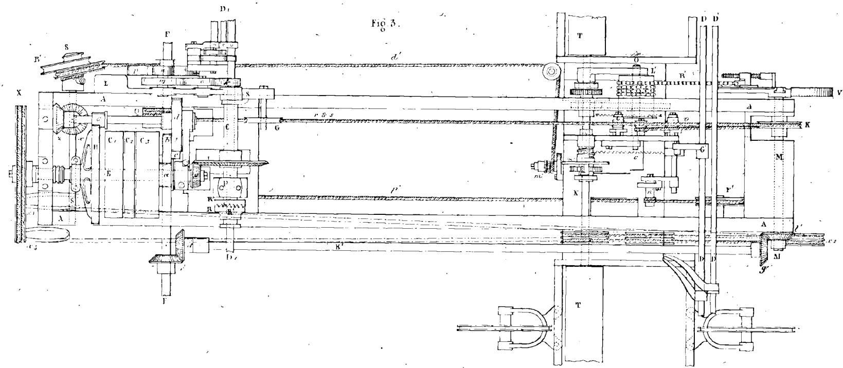
Echelle des figures 1, 2 et 3 0 m obli pour 1 mètre. la figure 4 est à une échelle double.
