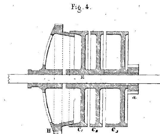
Echelle des figures 1, 2 et 3 0 m obli pour 1 mètre. la figure 4 est à une échelle double.
