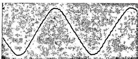
FIG. 8. — Courant d'une machine Gramme tétrapolaire. — Circuit non inductif. — La machine fournit d'autre part un courant continu : on reconnaît le passage des touches du collecteur sous les balais (période \frac{1}{60} ).
