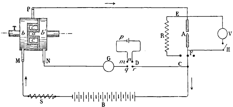
FIG. 1. — Disposition des appareils : T, commutateur tournant ; M et P, balais principaux ; N, balai du galvanomètre ; B, batterie d'accumulateurs (70 volts alimentant l'arc) ; S, résistance de stabilité sans induction ; G, galvanomètre ; p , élément d'accumulateur ; D, commutateur inverseur ; C, interrupteur à deux directions ; A, arc électrique ; E et F, bornes de la lampe ; R, résistance sans induction pouvant être substituée à l'arc ; V, voltmètre ; H, clef du voltmètre.
