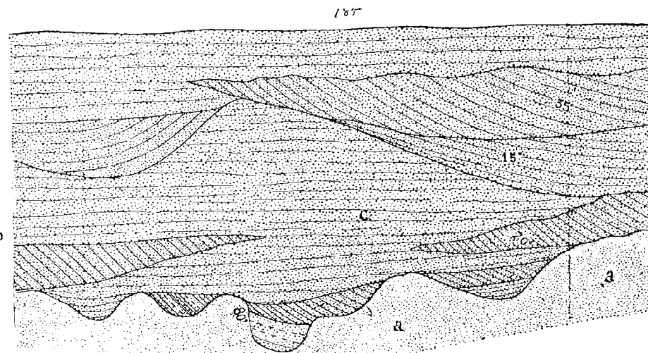
Fig. 183. Coupe des sables du bassin Freycinet à Dunkerque.
