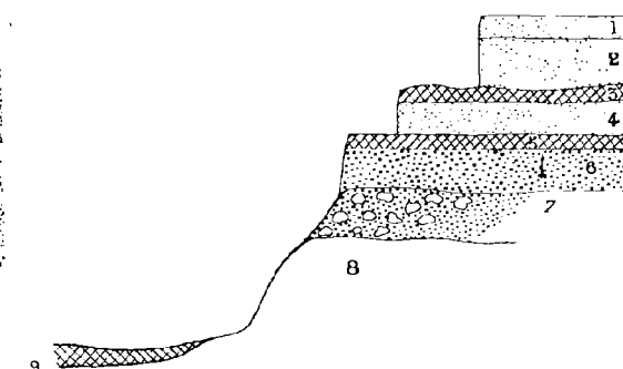
Fig. 183. Coupe de l'holocène à Wissant.
