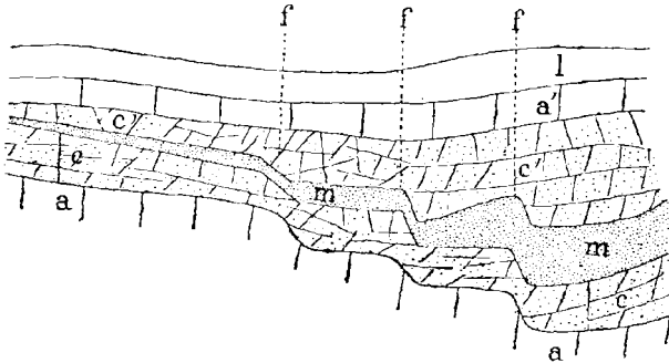
Fig. 2. — Coupe de la carrière Vaiteau à Crécy.
