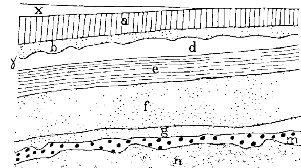
Fig. 166. Coupe du pleistocène Grimmeures
