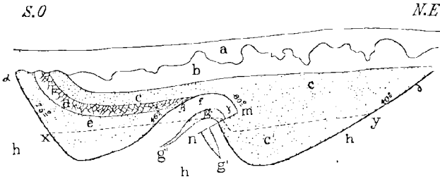
Fig. 3. — Coupe du chantier Patin à Marcheville.
