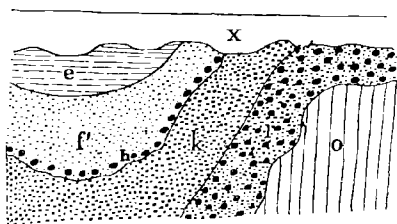
Fig. 158. Coupe du pleistocène à Moulin-Quignon près d'Abbeville.
