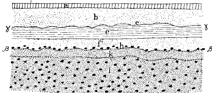
Fig. 160. Coupe du pleistocène à Angreau.
