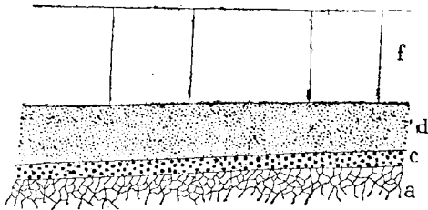
Fig. 14. — Coupe prise à l'entrée du souterrain de la carrière de Curlu
