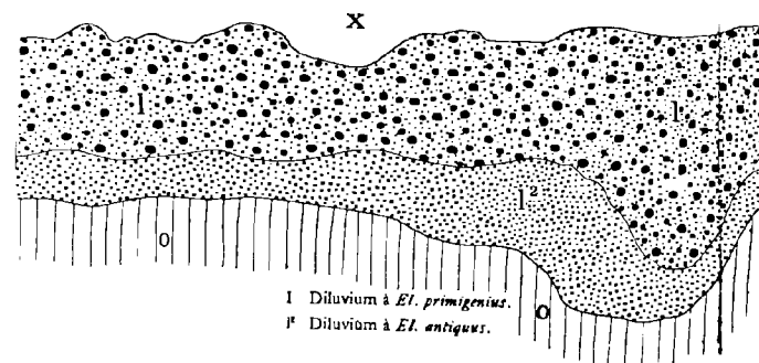
Fig. 175 Coupe du diluvium à Abbeville.
