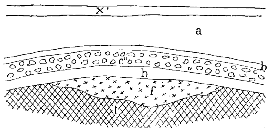
Fig. 180. Coupe d'une tourbière à Aveluy, d'après M. Debray.
