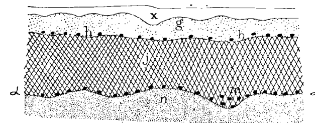
Fig. 175. Coupe des dépôts de la grotte d'Hydroquent, par M. Hamy.
