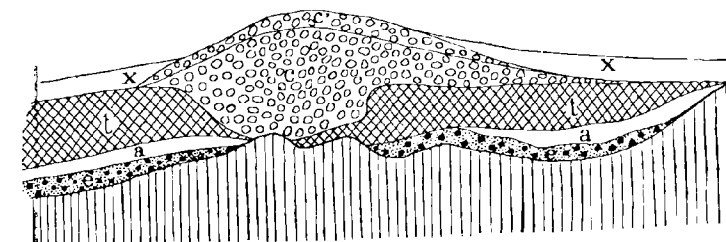
Fig. 184. Coupe d'une tourbière à Ardres.
