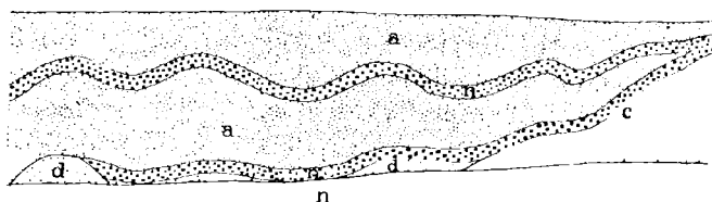
Fig. 4. — Coupe du sable phosphaté à l'exploitation Dancieux, près du chemin de Préel en 1900
