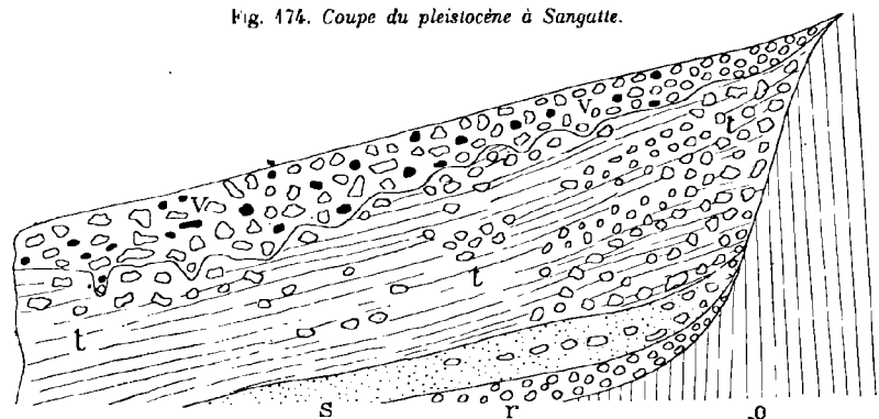
Fig. 174. Coupe du pleistocène à Sangatte.
