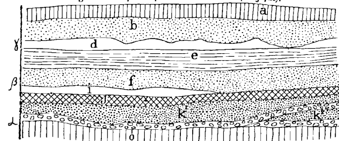
Fig. 165. Coupe du pleistocène à Fontaine-au-Bois.
