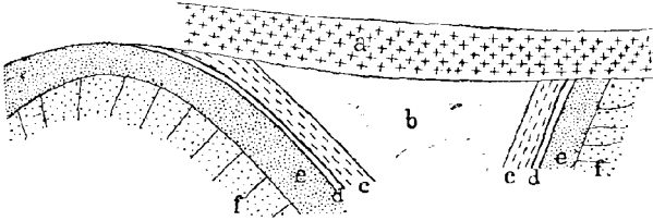
Fig. 1. — Coupe d'une poche de sable phosphaté, à Beauval.
