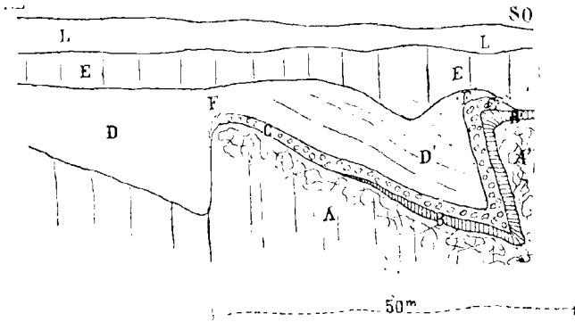
Fig. 1. — Coupe d'une carrière de craie phosphatée à Étaves.
