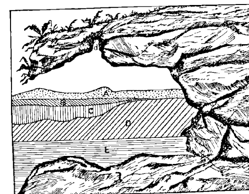
Fig. 171. Coupe du pleistocène au Mont des Calz.
