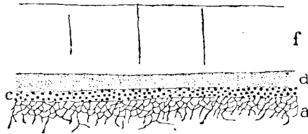
Fig. 12. — Coupe prise à l'entrée de l'exploitation de phosphate de chaux de Mont St-Quentin
