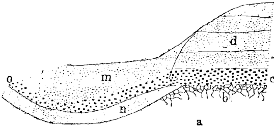
Fig. 7 — Coupe d'une poche dans le chantier Rouzé, à Haravesne.
