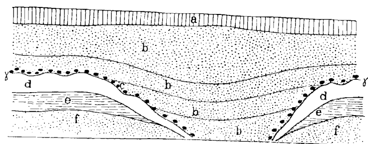
Fig. 164. Coupe du pleistocène à Hébemont-sur-Oise.
