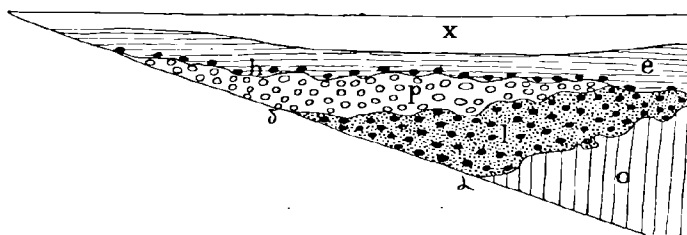
Fig. 167. Coupe du pleistocène à Haumont.
