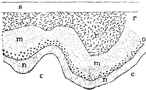
Fig. 6. — Coupe d'une poche dans le chantier Rouzé, à Haravesne
