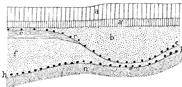
Fig. 173. Coupe du pleistocène à Menhecourt près Abbeville, par M. Prestwich
