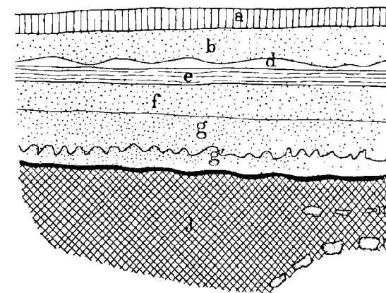
Fig. 165. Coupe du pleistocène à Fontaine-au-Bois.
