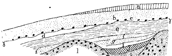
Fig. 162. Coupe du pleistocène au Cateau.
