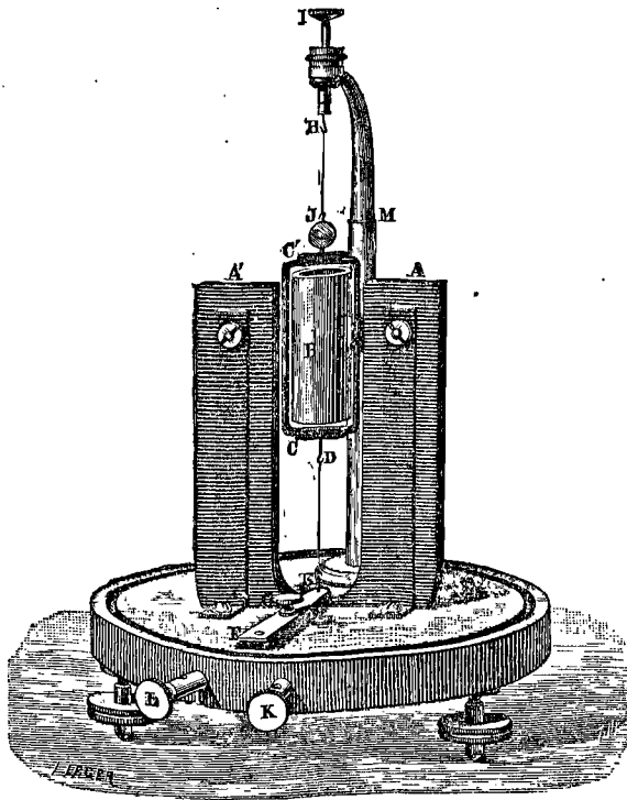
Fig. 177. — Galvanomètre Deprez et d'Arsonval. ( Lumière électrique. )
