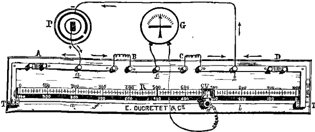
Fig. 200. — Pont de Wheatstone à rhéocorde. (Ducretet.)
