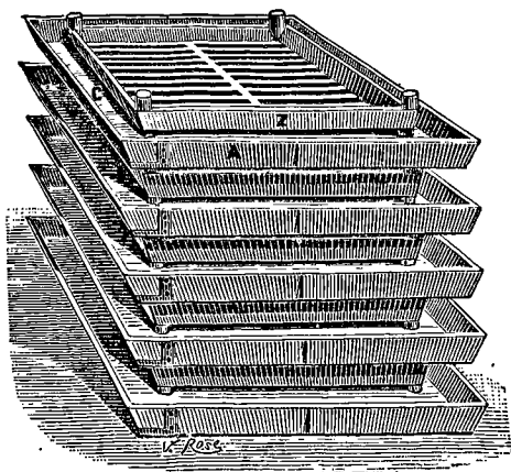
Fig. 234. — Pile de Sir William Thomson. ( La Lumière électrique. )
