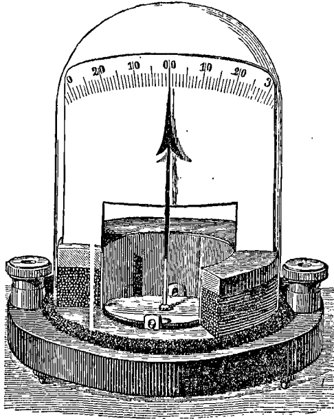
Fig. 181. — Galvanomètre Bréguot. (Ducretet.)
