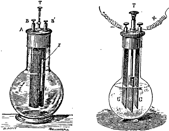
Fig. 233 et fig. 237. — Éléments Grenet.
