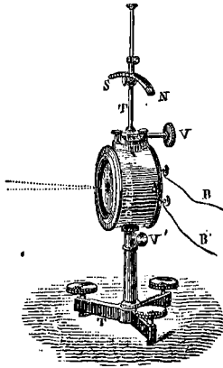
Fig. 174. — Galvanomètre Thomson. (Ducretet.)
