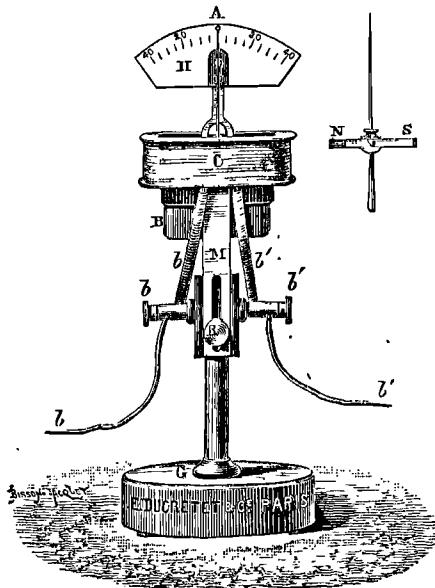
Fig. 180. — Galvanomètre de démonstration. (Ducretet.)
