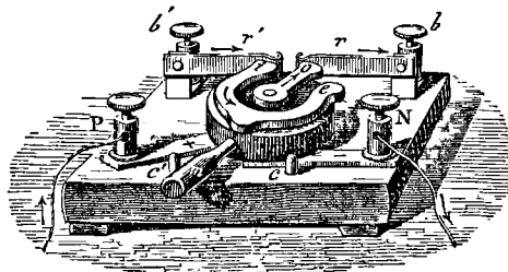
Fig. 162. — Commutateur de Bortin. (Ducretet.)
