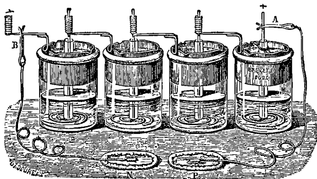
Fig. 232. — Pile Callaud.
