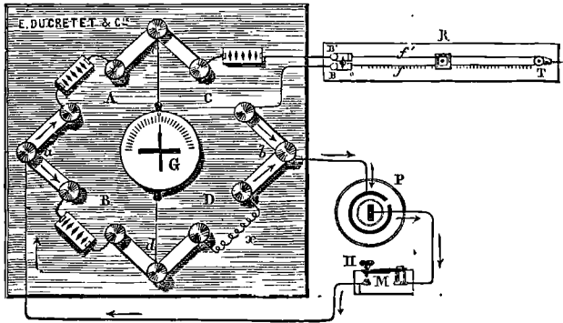
Fig. 199. — Pont de Wheatstone. (Ducretet.)
