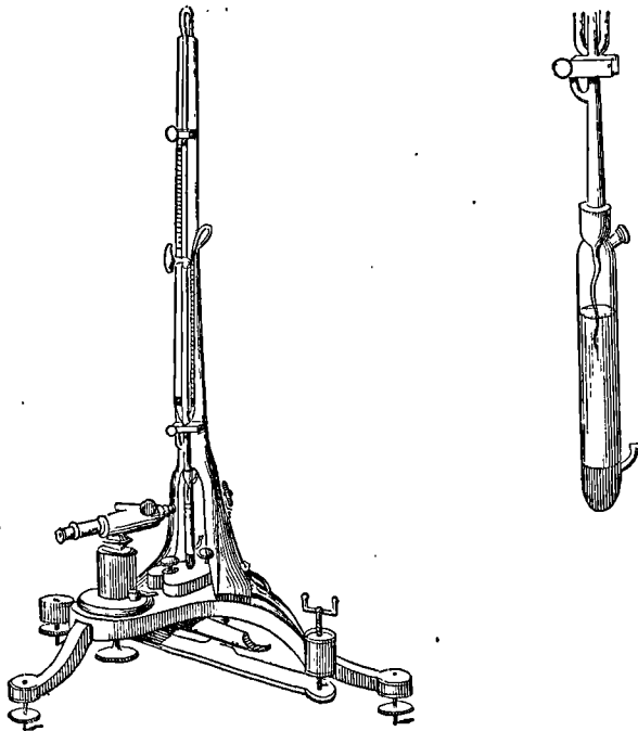
Fig. 193. — Electromètre capillaire Lipmann.
