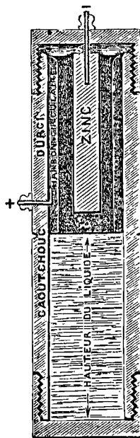
Fig. 229. — Pile hermétique, modèle Trouvé.
