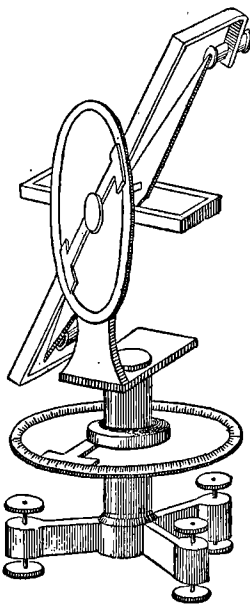
Fig. 149. — Boussole d'inclinaison.
