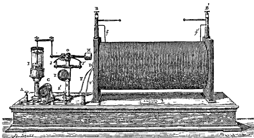
Fig. 248. — Bobine de Ruhmkorff avec interrupteur simple à mercure. (Gaiffé.)
