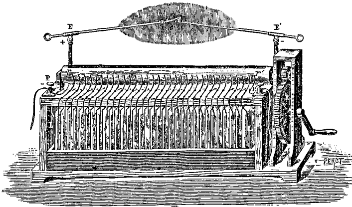
Fig. 213. — Machine rhéostatique. (Planté.)
