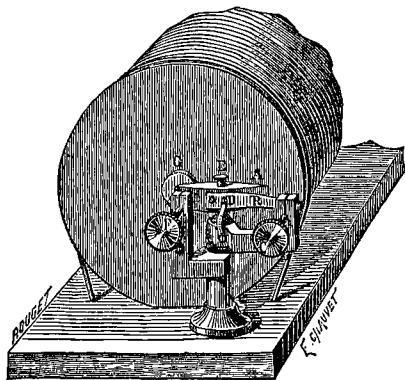
Fig. 245. — Interrupteur Marcel Deprez. (Carpentier.)
