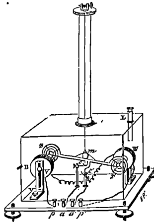
Fig. 184. — Balance de Lallemand. (Ducretet.)
