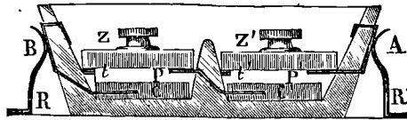
Fig. 227. — Pile à sulfate de mercure. (Gaiffe.)
