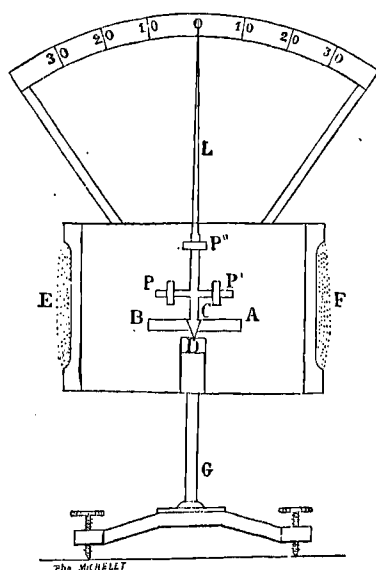
Fig. 170. — Galvanomètre de Bourbouzo. (Ducretet.)
