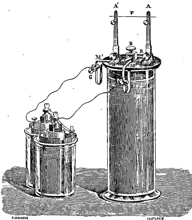
Fig. 240. — Élément secondaire Planté, en charge.
