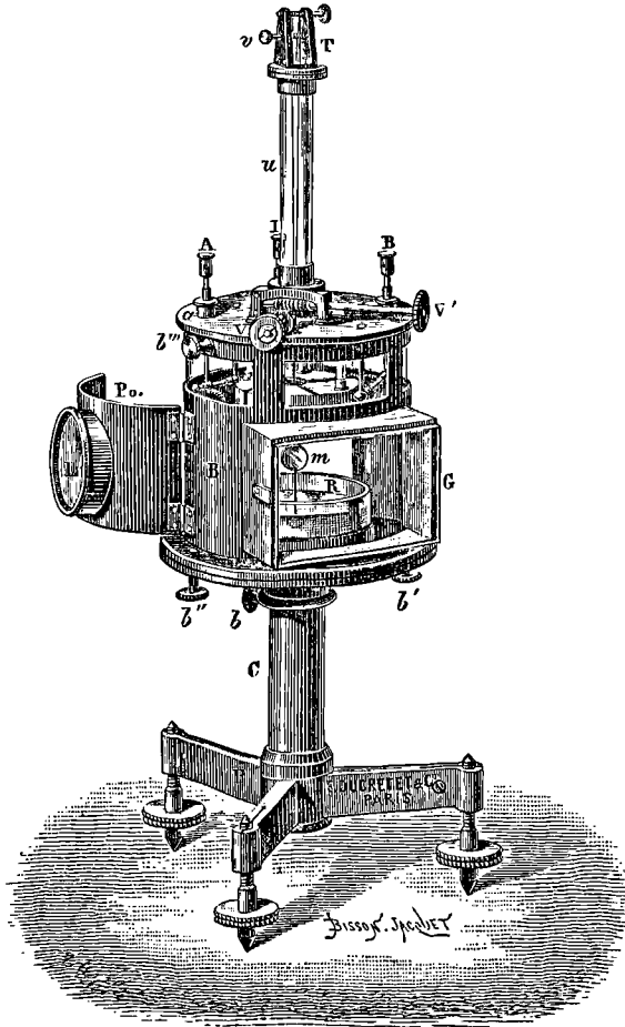
Fig. 191. — Électromètre. (Ducretet.)
