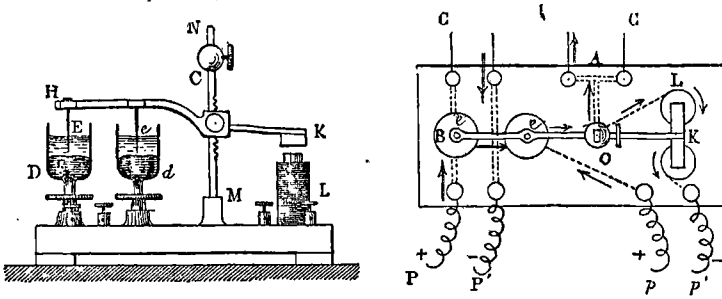
Fig. 247. — Interrupteur Foucault.
