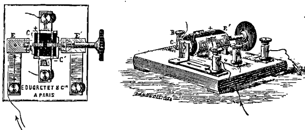
Fig. 160 et 161. — Commutateur Ruhmkorff. (Ducet.)
