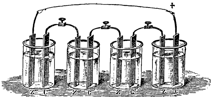
Fig. 216. — Pile à couronne de tasses.
