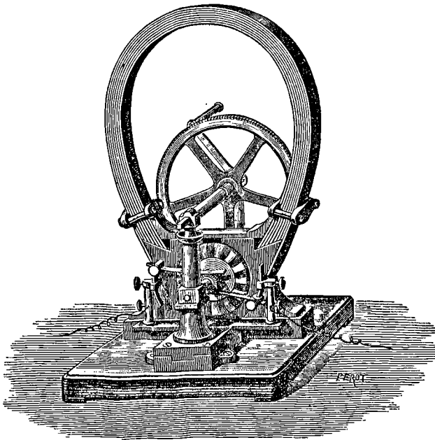
Fig. 252. — Machine Gramme. (Bréguet.)
