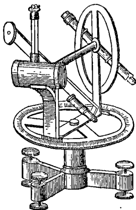
Fig. 143. — Théodolite-boussole.
