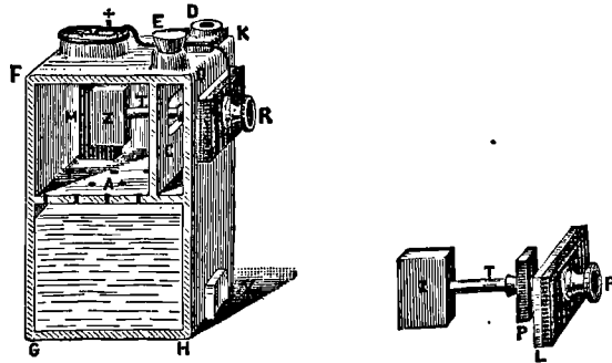
Fig. 239. — Pile Fauché.
