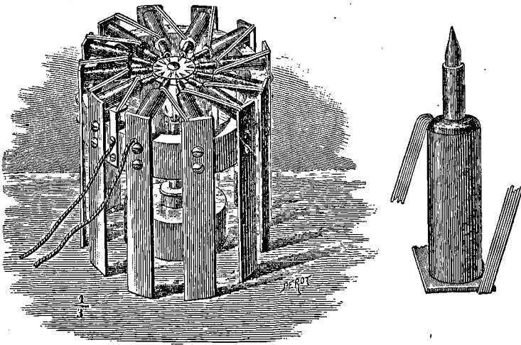
Fig. 242. — Pile thermo-électrique de Noé. (Dréquet.)
