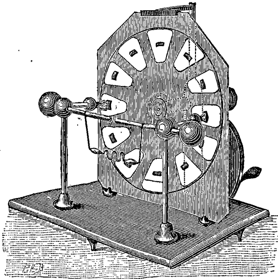
Fig. 210. — Machine Toepler. ( La Lumière électrique. )
