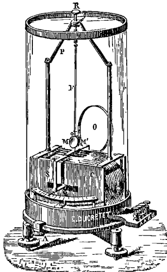
Fig. 167. — Galvanomètre différentiel. (Ducretet.)
