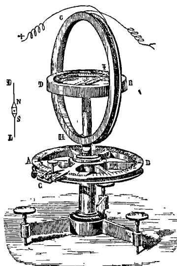
Fig. 160. — Boussole des tangentes. (Ducretet.)
