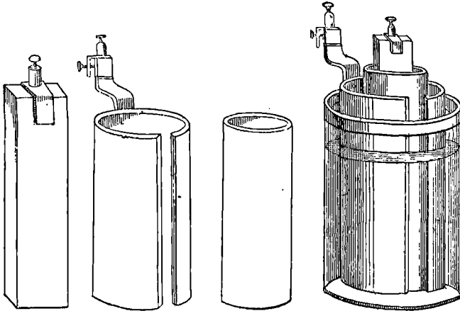
Fig. 235. — Élément de Bunsen.
