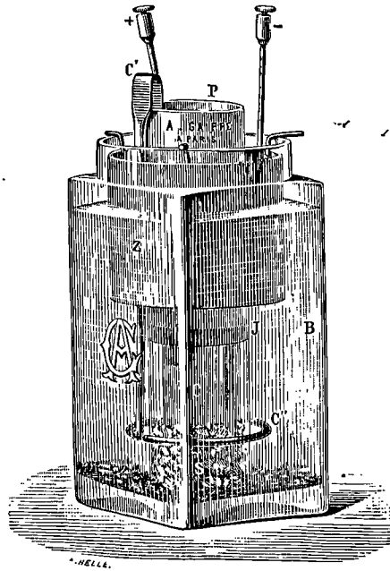
Fig. 231. — Élément de Gaiffe au sulfate de cuivre. (Gaiffe.)
