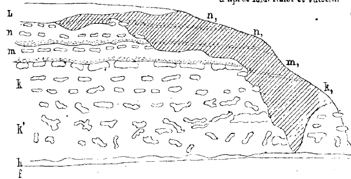
Fig. 151. — Coupe de la colline de Wemmet.
