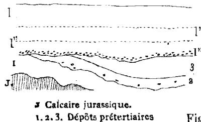
Fig. 126. Coupe d'une tranchée à Neuve-Maison.
