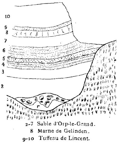
Fig. 134. Coupe d'une sablière à Owillers.
