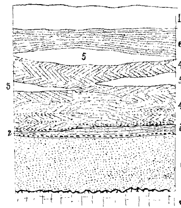
Fig. 141. Coupe de la sablière d'Erquelines. d'après M. Rutot.
