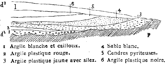
Fig. 139. Coupe d'une sablière à Offies.
