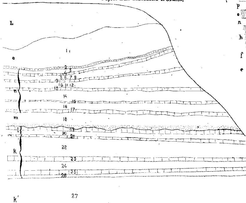
Fig. 147. — Coupe de la carrière du M t des Récollets.
