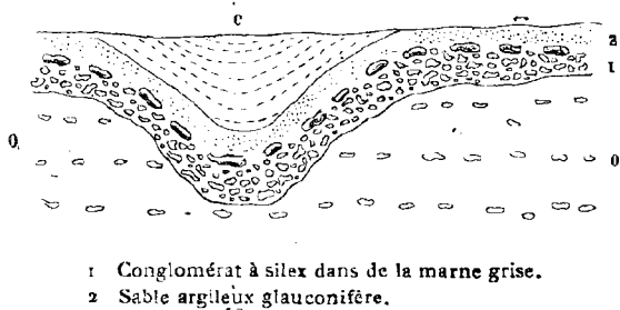
Fig. 124. Coupe du conglomérat à silex, à Briastre.
