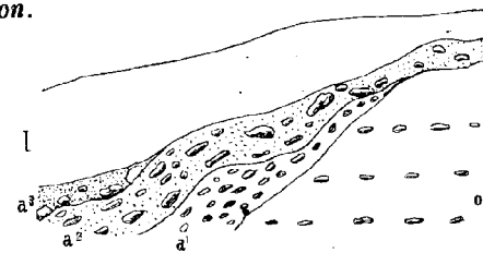
Fig. 128. Coupe d'une tranchée à Neuville.
