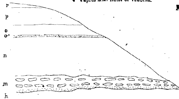
Fig. 151. — Coupe de la colline de Wemmet.
