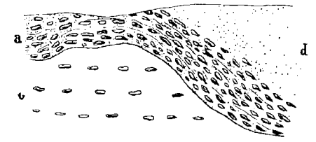
Fig. 131. Coupe d'une sablière à Ostricourt.
