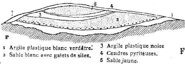
Fig. 142. Coupe du landenien à Viesly.
