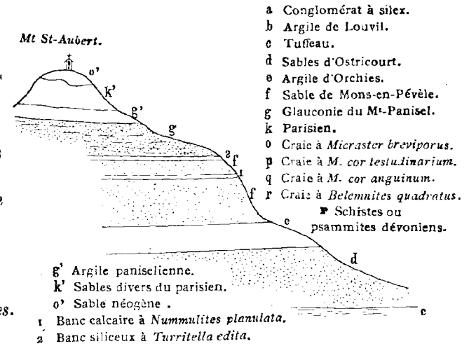
Fig. 144. Coupe théorique du Mont de la Trinité. d'après MM. Ortlieb et Chellonneix.
