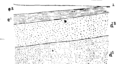
Fig. 131. Coupe d'une sablière à Ostricourt.
