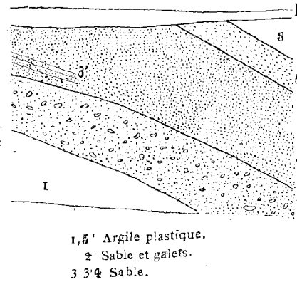
Fig. 141. Coupe de la sablière d'Erquelines. d'après M. Rutot.
