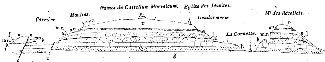
Fig. 148. — Coupe des M ts Cassel et des Récollets.
