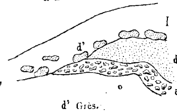
Fig. 133. Coupe des carrières de grès à Beaurain.
