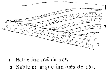
Fig. 136. Coupe d'une sablière à Bertaimont.
