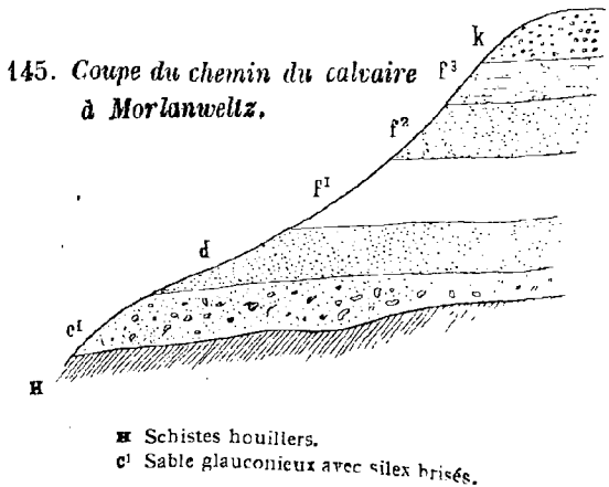
Fig. 143. Coupe théorique de la colline de Mons-en-Pévèle. d'après MM. Ortlieb et Chellonneix.
