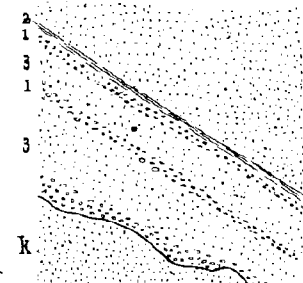
Fig. 156. — Coupe dans les sables de Diest au M t de Boëschepe.
