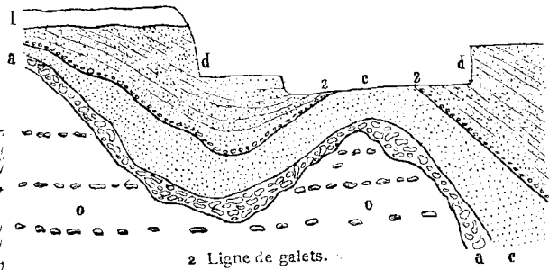
Fig. 137. Coupe d'une sablière à Beugnies.
