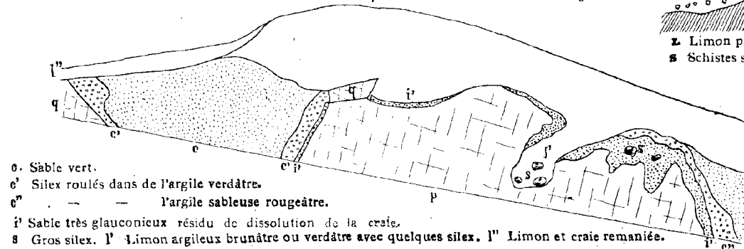
Fig. 128. Coupe d'une tranchée à Neuville.
