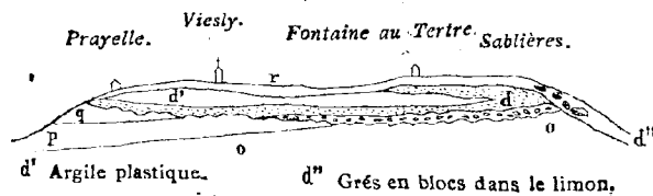
Fig. 142. Coupe du landenien à Viesly.
