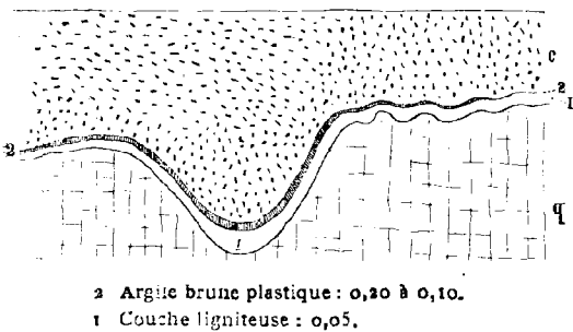
Fig. 124. Coupe du conglomérat à silex, à Briastre.
