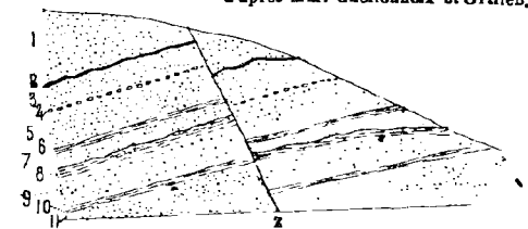
— Coupe du chemin de la Hotte-en-bas au M t Noir. d'après MM. Chellonneix et Ortlieb.
