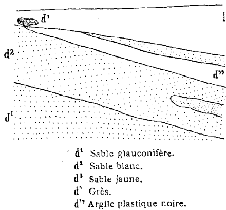
Fig. 136. Coupe d'une sablière à Bertaimont.
