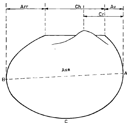
FIG. 4 c — Valve d'ASMUSSIIDAE
