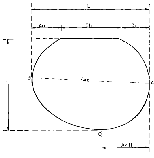
FIG. 4 a — Valve de LIOESTHERIIDAE cycladiforme
