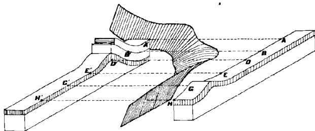
FIG. 2. - Interprétation schématisique du décrochement. Les deux blocs diagrammes représentent les deux panneaux séparés par le décrochement, le panneau occidental à gauche et le panneau oriental à droite. Les plis longitudinaux et transversaux qui les affectent ne sont pas figurés. Une même lettre (par exemple A et A') désignent deux points en regard l'un de l'autre, de part et d'autre du décrochement.
