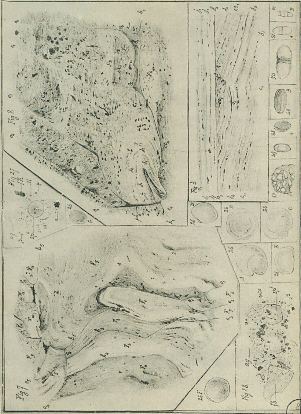
SECTIONS HORIZONTALES ET SPORES DU BROWN OILSHALE DE LA RÉGION DE BROXBURN. ORGANITES DU SCHISTE BITUMEUX DU BOIS D'ASSON.
