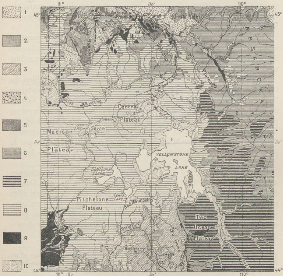
FIG. 262. — Carte géologique du Yellowstone National Park, d'après Arn. Hague, J. P. Idings et W. H. Weed ( U. S. Geol. Survey, Atlas to accompany Monograph XXXII, part 2, pl. XVII, Washington, 1904 ).
