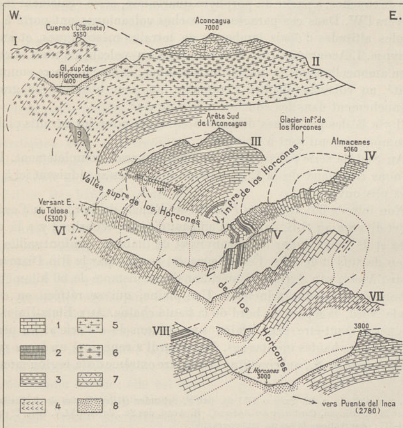
FIG. 298. — Coupes échelonnées de Puente del Inca à l'Aconcagua (Andes Argentines), d'après W. Schiller ( Neues Jahrb. für Mineralogie , Beilage-Bd. XXIV, 1907, pl. XLVI).
