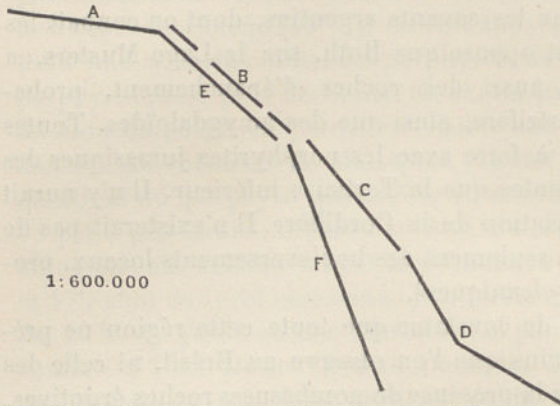
FIG. 302. — Lignes directrices de la Sierra de la Ventana, d'après R. Hauthal.
