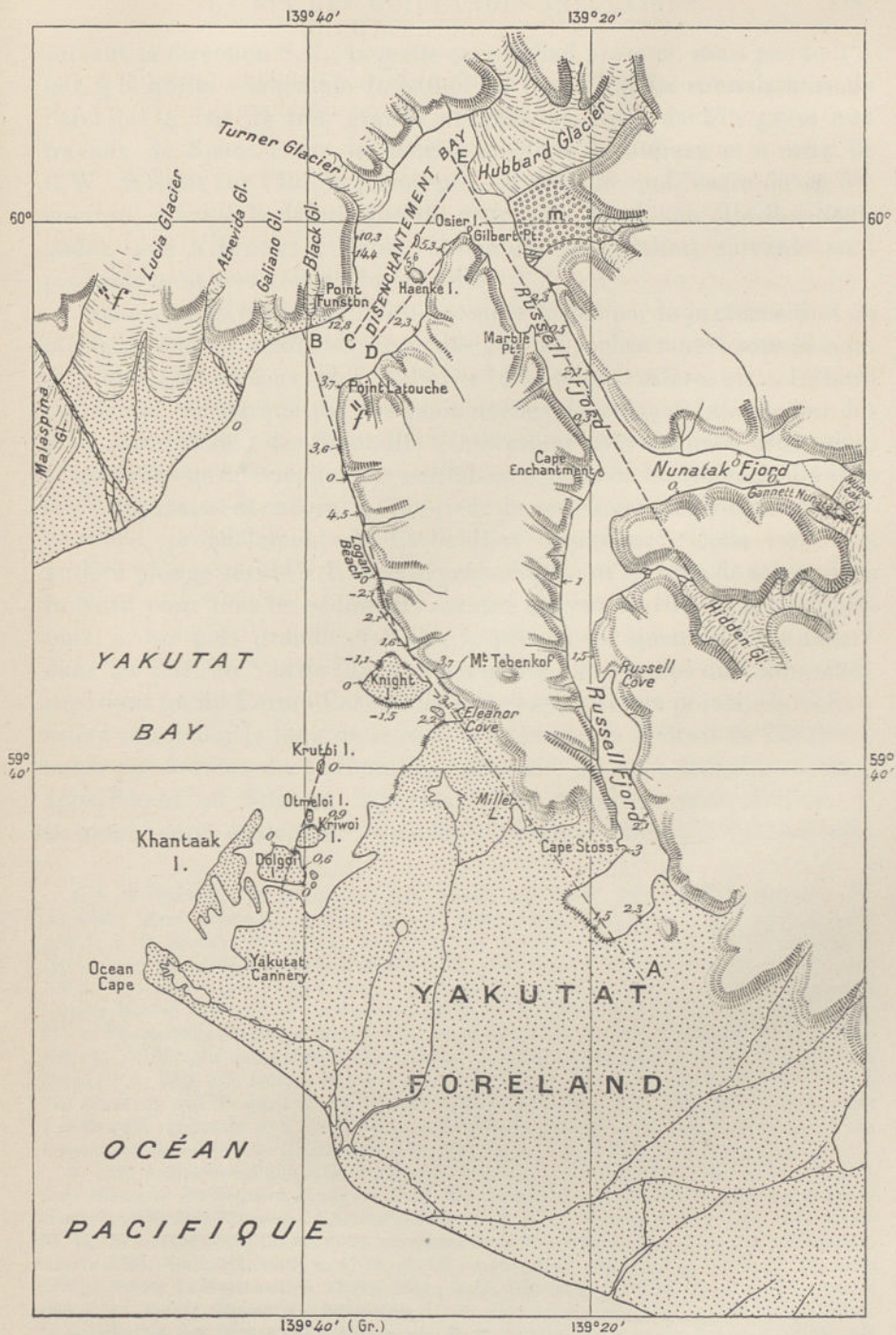
FIG. 269. — Failles récentes de la Baie de Yakutat (Alaska), d'après Ralph S. Tarr et Lawrence Martin ( Bull. Geol. Soc. of America , XVII, 1903, p. 54, pl. 23).
