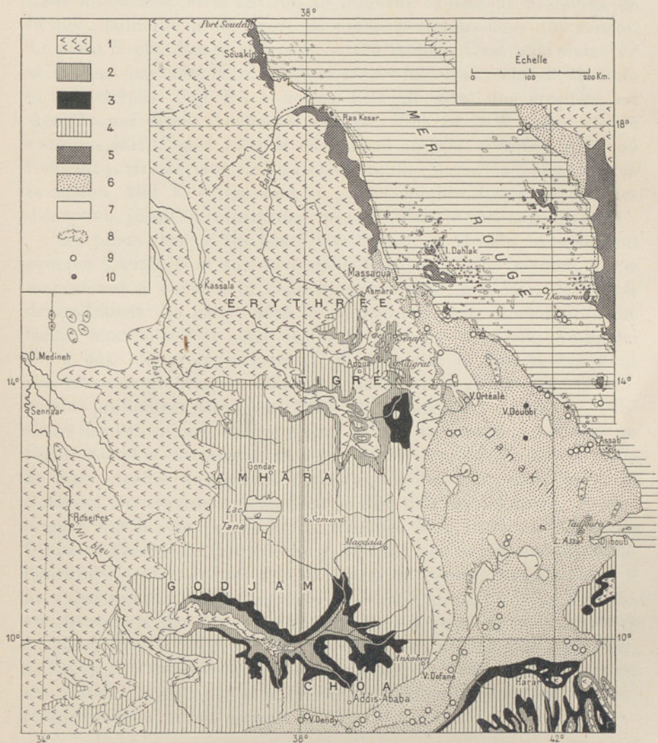
FIG. 222. — Carte géologique de l'Abyssinie, d'après G. Dainelli et O. Marinelli (in : A. Ghisleri, Atlante d'Africa . In-4°, Bergamo, 1909, p. 31-32).
