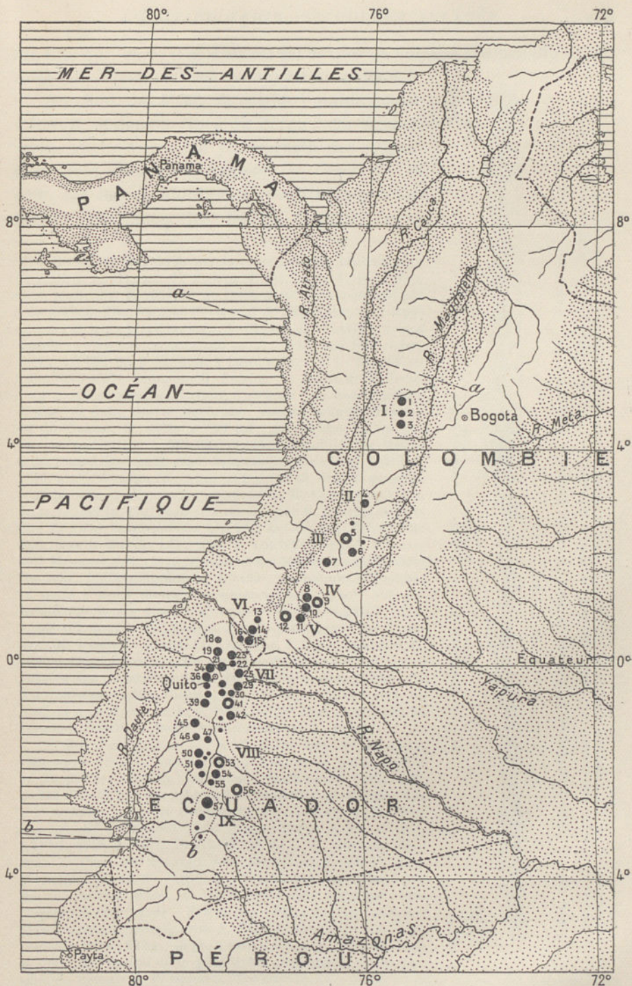
FIG. 294. — Distribution des principaux centres volcaniques dans les Andes de la Colombie et de l'Équateur, d'après A. Stübel ( Petermanns Mitteil. , XLVIII, 1902, pl. I).
