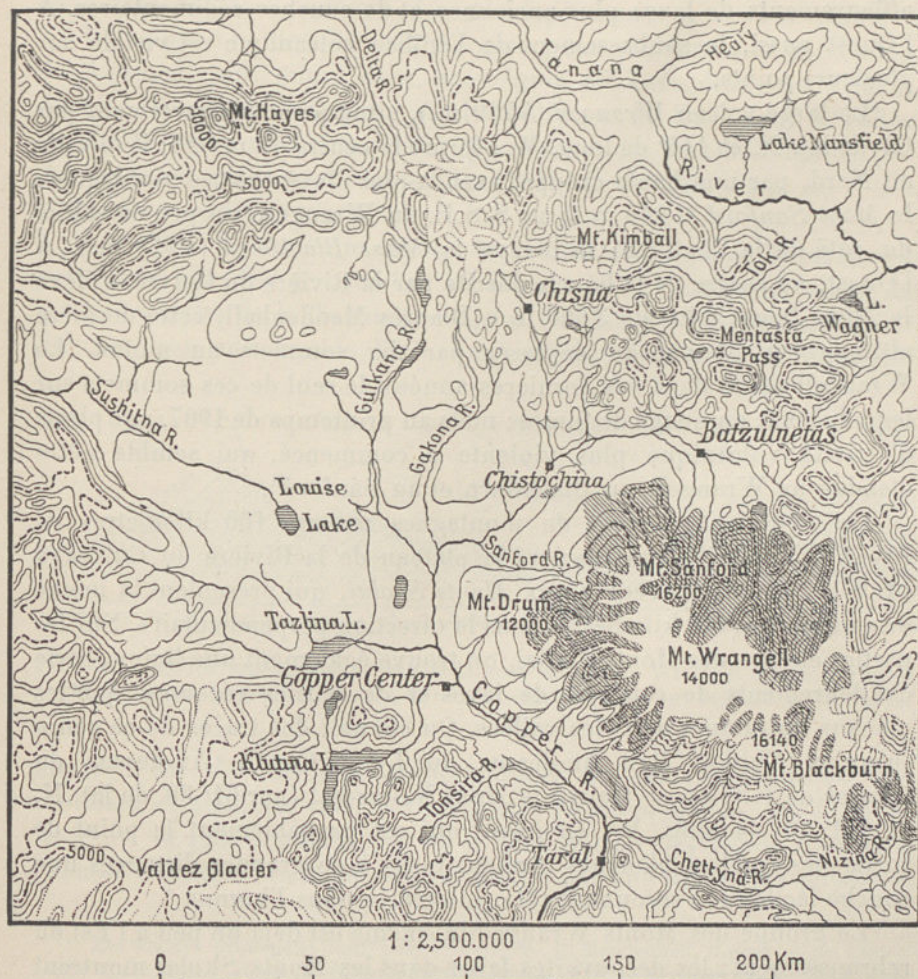
FIG. 267. — Le Plateau de la Rivière du Cuivre, d'après la carte de R. U. Goode (in A. H. Brooks, The Geography and Geology of Alaska ; U. S. Geol. Survey, Prof. Paper 43, pl. XXXIV, 1906). Indications géologiques d'après Mendenhall, Schrader et Spencer. Hauteurs en pieds anglais.
