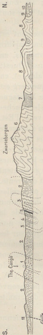
FIG. 227. — Chaînes du Cap. Coupe du faisceau des Zwartebergen à l'Est du village de Prince Albert, d'après A. W. Rogers et A. L. Du Toit ( An Introduction to the Geology of Cape Colony , 2 e ed. In-8 o , London, 1909, p. 40, fig. 4).
