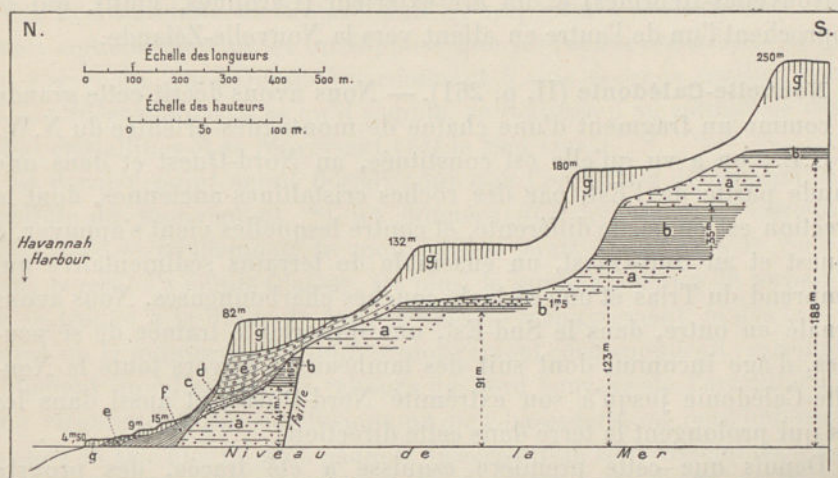
FIG. 236. — Terrasses coralliennes d'Efate (Nouvelles-Hébrides). Coupe de Steep Gully, Havannah Harbour, d'après D. Mawson ( Proc. Linnæan Soc. New South Wales , XXX, 1905, pl. XXIV).
