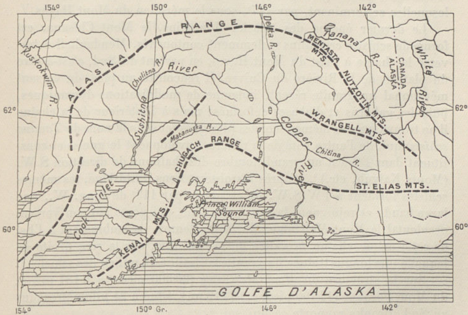
Fig. 249. — Directrices orographiques de l'Alaska Central, d'après W. C. Mendenhall (U. S. Geol. Survey, Professional Paper n° 41, 1905, p. 80, fig. 7).
