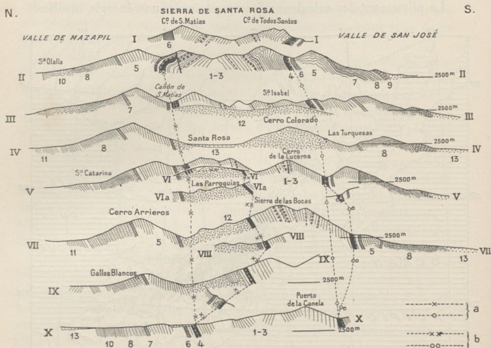
FIG. 283. — Coupes à travers la Sierra de Santa Rosa (Mexique), d'après C. Burckhardt ( Guide des Excursions du X e Congrès Géologique International, Mexico, 1906, n o XXVI ).
