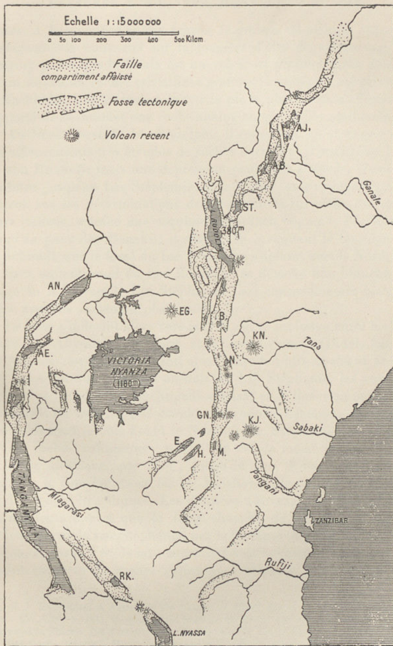
FIG. 221. — Les fossés de l'Afrique Orientale, d'après Emm. de Martonne ( Traité de Géographie Physique . In-8°, Paris, 1909, p. 487, fig. 219).
