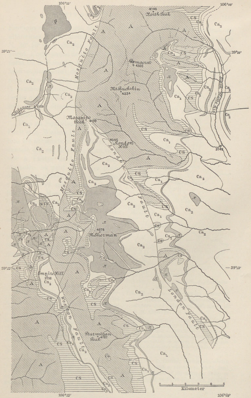
FIG. 257. — Les Montagnes Rocheuses à l'Est de Leadville (Colorado), d'après S. F. Emmons (U. S. Geol. Survey, Monograph XII, Atlas, 1883, feuilles VI et VII).
