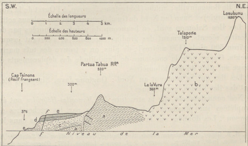
FIG. 235. — Coupe prise au Sud-Ouest d'Espiritu-Santo (Nouvelles-Hébrides), d'après D. Mawson ( Proc. Linnean Soc. New South Wales , XXX, 1905, pl. XXV).
