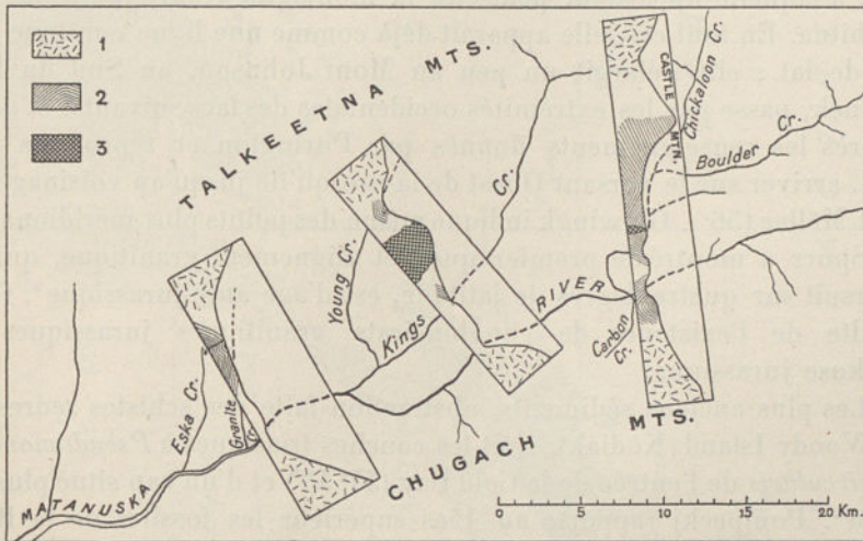
FIG. 251. — Trois coupes à travers la dépression tertiaire de la Matanuska, d'après G. C. Martin ( U. S. Geol. Survey, Bull. n° 289, 1906, p. 16, fig. 2 ).
