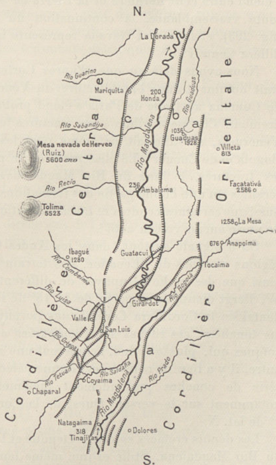
FIG. 293. — Réseau de cassures de la vallée du Magdalena (Colombie), d'après H. Stille ( Festschrift zum siebenzigsten Geburtstag von Adolf v. Koenen gewidmet von seinen Schülern . In-8°, Stuttgart, 1907, pl. 10, fig. 1).
