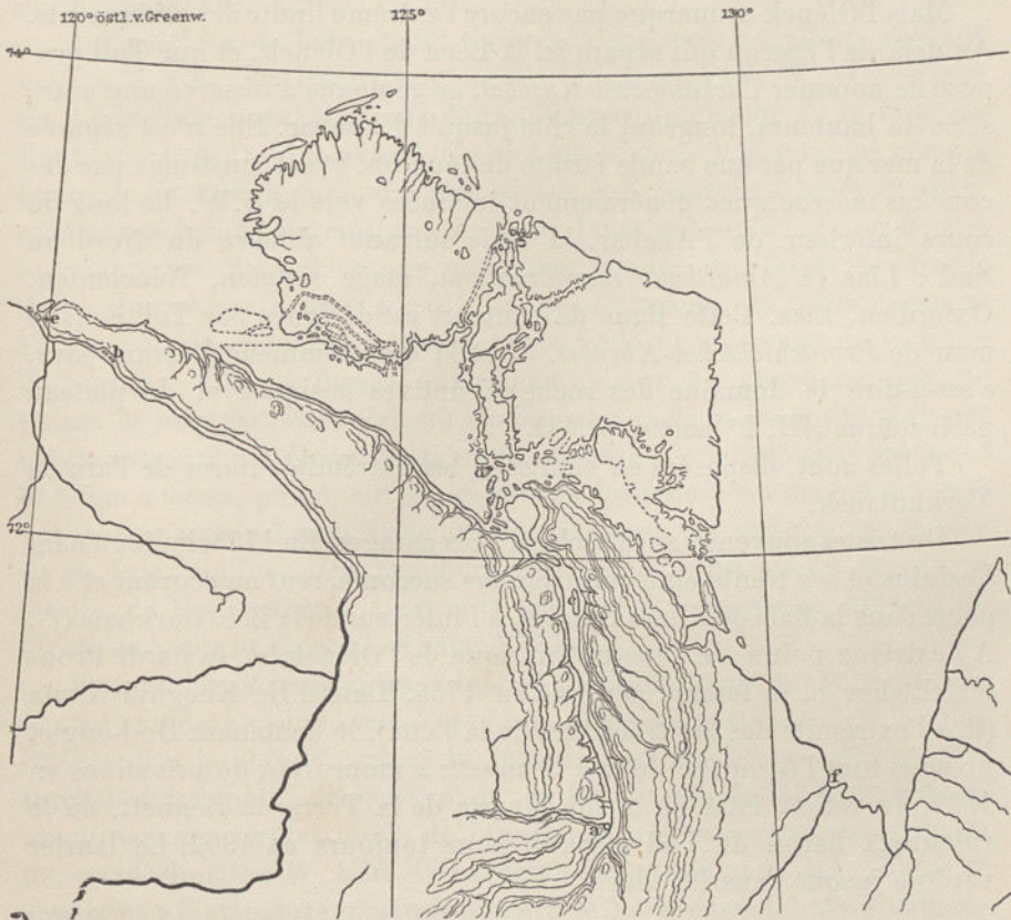
FIG. 241. — Le Delta de la Léna, d'après A. Eigner ( Beobachtungen der Russischen Polarstation an der Lenamündung, II. Theil. Expedition der Kaiserl. Geographischen Gesellschaft. In-4°, St.-Petersburg, 1886 ).
