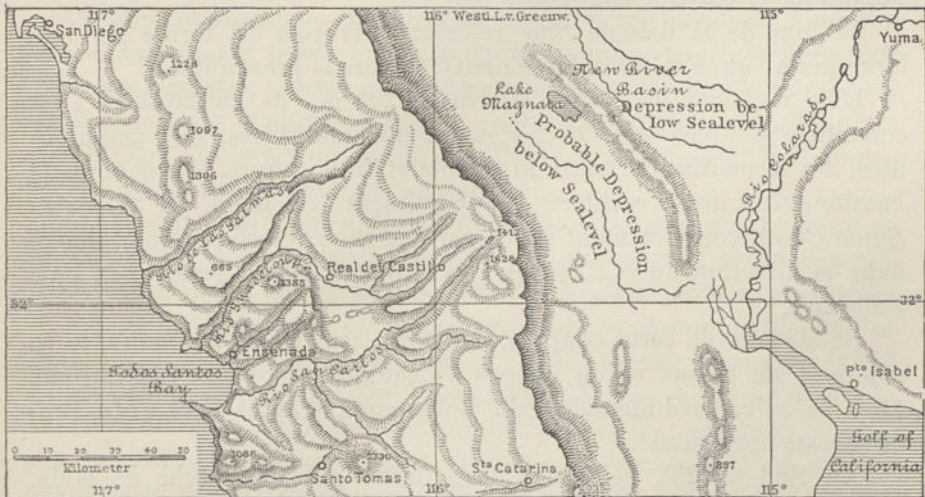
FIG. 279. — L'embouchure du Colorado, d'après W. Lindgren.
