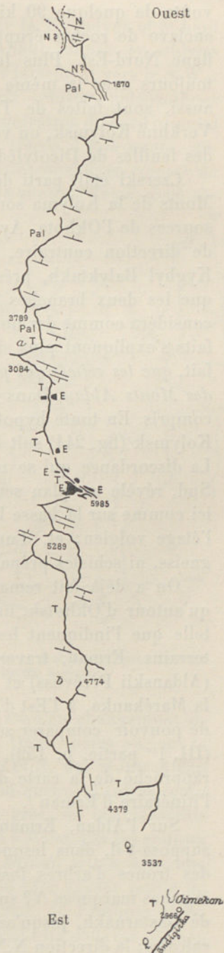
FIG. 243. — Les montagnes de Verkhoïansk entre l'Aldan et l'Indighirka. — Itinéraire se développant de l'Ouest à l'Est, d'après Czarski.
