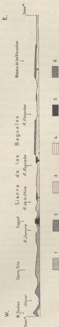
FIG. 304. — Andes de Patagonie. Coupe du Mont Stokes à la branche Nord du Rio Coyle, d'après R. Hauthal (Bertche der Naturforsch. Gesellsch. zu Freiburg i. Br., XV, 1905, pl. I, 1907).
