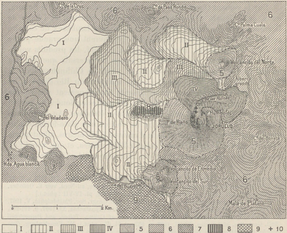
FIG. 281. — Éruptions successives du Jorullo, d'après E. Ordoñez ( Guide des Excursions du X e Congrès Géologique International, Mexico, 1906, n° XI ; carte reprod. Scottish Geogr. Magazine, XXIII, 1907, p. 336 ).
