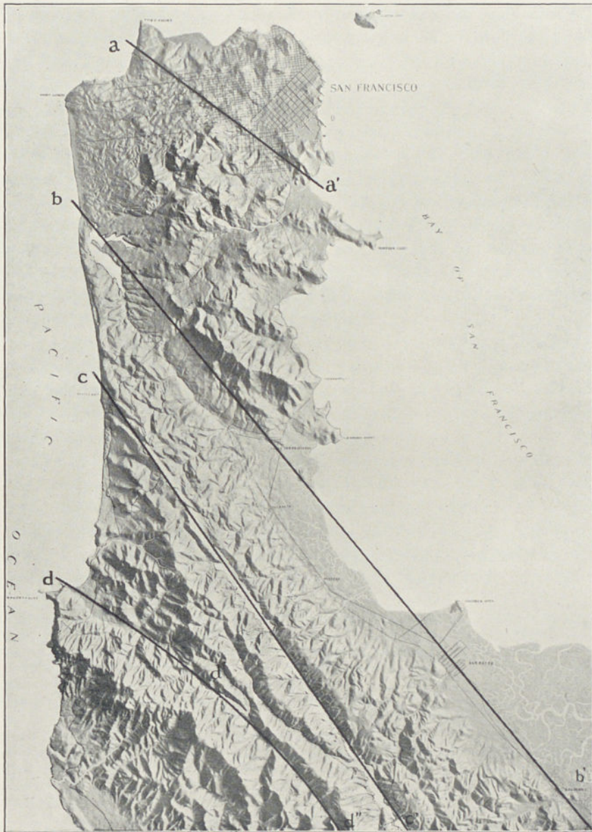
LA PRESQU'ÎLE DE SAN FRANCISCO, d'après un relief modelé par A. C. LAWSON
