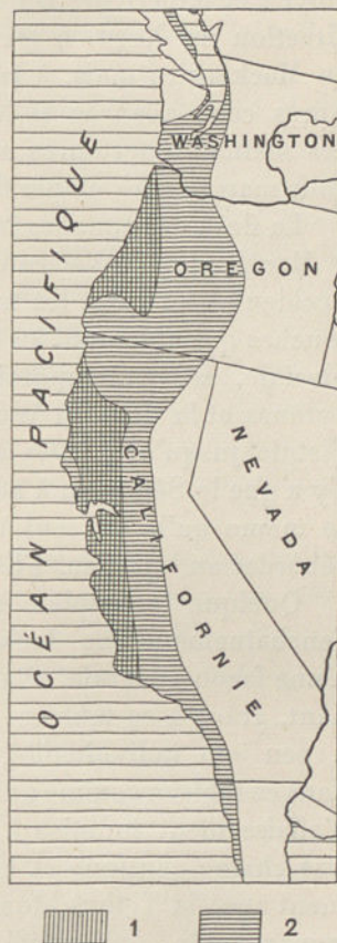
FIG. 287. — Extension des mers crétacées le long du Littoral Pacifique des États-Unis, d'après J. S. Diller et T. W. Stanton (Bull. Geol. Soc. of America, V, 1894, p. 454, fig. 1).
