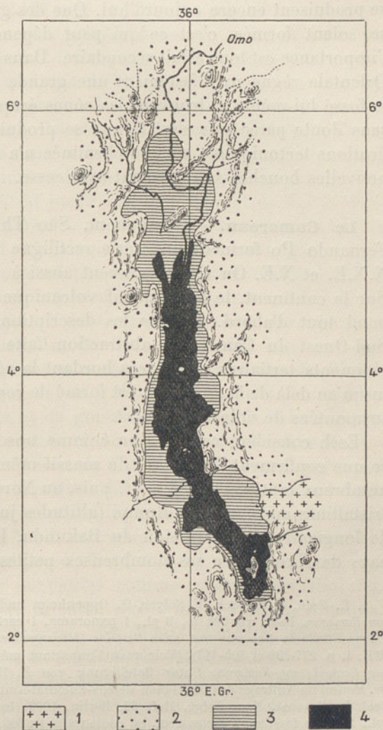
FIG. 224. — Ancienne extension du Lac Rodolphe, d'après M. Sacchi, G. De Angelis d'Ossat et F. Millosevich ( Seconda Spedizione Bottego. Studio geologico . In-8°, Roma, 1900, p. 205, fig. 25).
