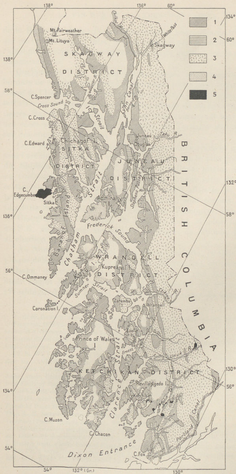
FIG. 270. — Géologie de la Côte Sud-Est de l'Alaska (Archipel Alexandre), d'après C. W. Wright (U. S. Geol. Survey, Bull. n° 345, 1908, pl. II). 1. Terrains paléozoïques (calcaires, phyllades et roches éruptives intercalées); 2. Terrains mésozoïques (granites, schistes ardoisiers, conglomérats, andésites et tufs); 3. Roches intrusives de la Chaîne Côtière (granite, granodiorite et diorite); 4. Terrains tertiaires (grès, conglomérats et laves rhyolitiques); 5. Laves et tufs basaltiques récents. — Échelle de 1 : 3 500 000 environ.
