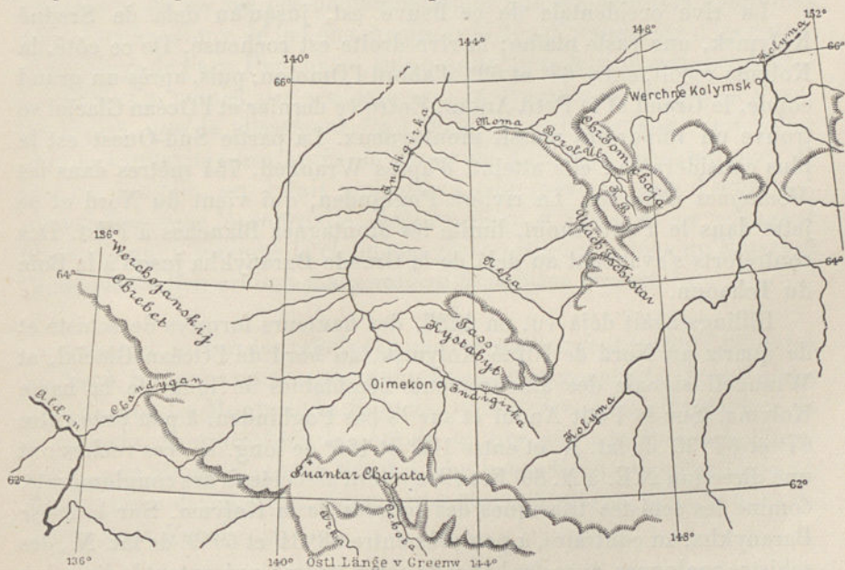
FIG. 244. — Esquisse du cours supérieur de l'Indighirka et de la Kolyma, d'après Czernski. K. B. = Kygyl-Balyktach. — Échelle de 1 : 7 500 000 environ.
