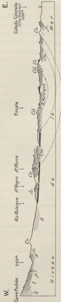
FIG. 299. — Andes Argentines. Coupe de la vallée du Rio Malargué, d'après C. Burckhardt ( Profils géologiques transversaux de la Cordillère. Anales del Museo de La Plata, Sección Geol. y Mineralog., II. In-F., 1900, pl. XXX, fig. 1 ).
