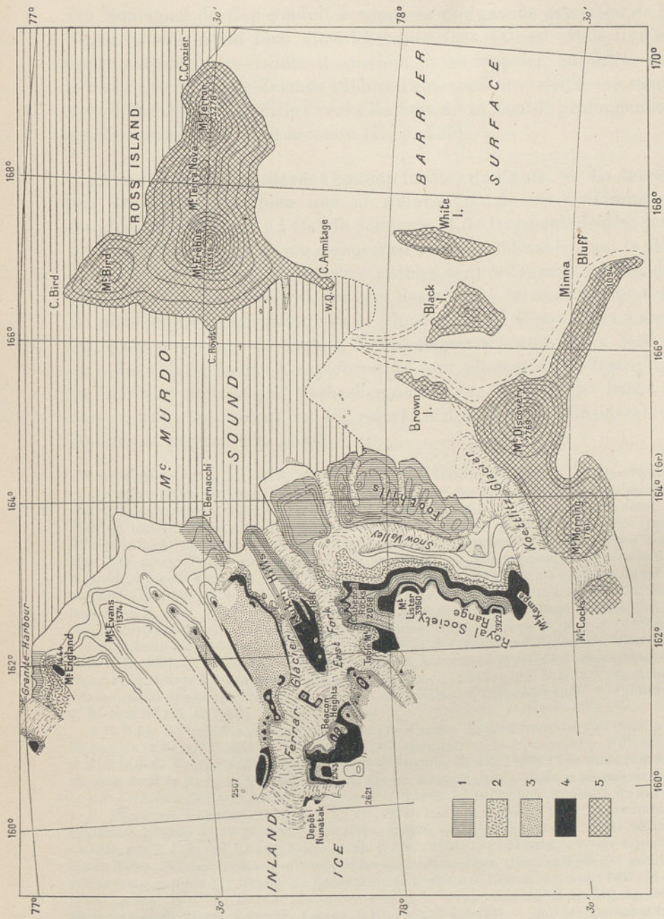
Fig. 230. — Carte géologique d'une partie de la Terre Victoria, d'après H. T. Ferrar ( National Antarctic Expedition, 1901-1904. Natural History, Vol. I. Geology. In-4°, London, 1907, carte à la fin du vol. ).
