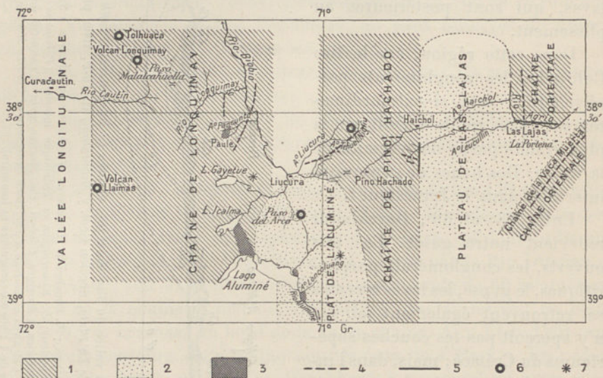
FIG. 300. — Esquisse tectonique de la région comprise entre Las Lajas (République Argentine) et Curacaútin (Chili), d'après C. Burckhardt ( Anales del Museo de La Plata, Sección Geol. y Mineralog. , III, 1900, pl. I).
