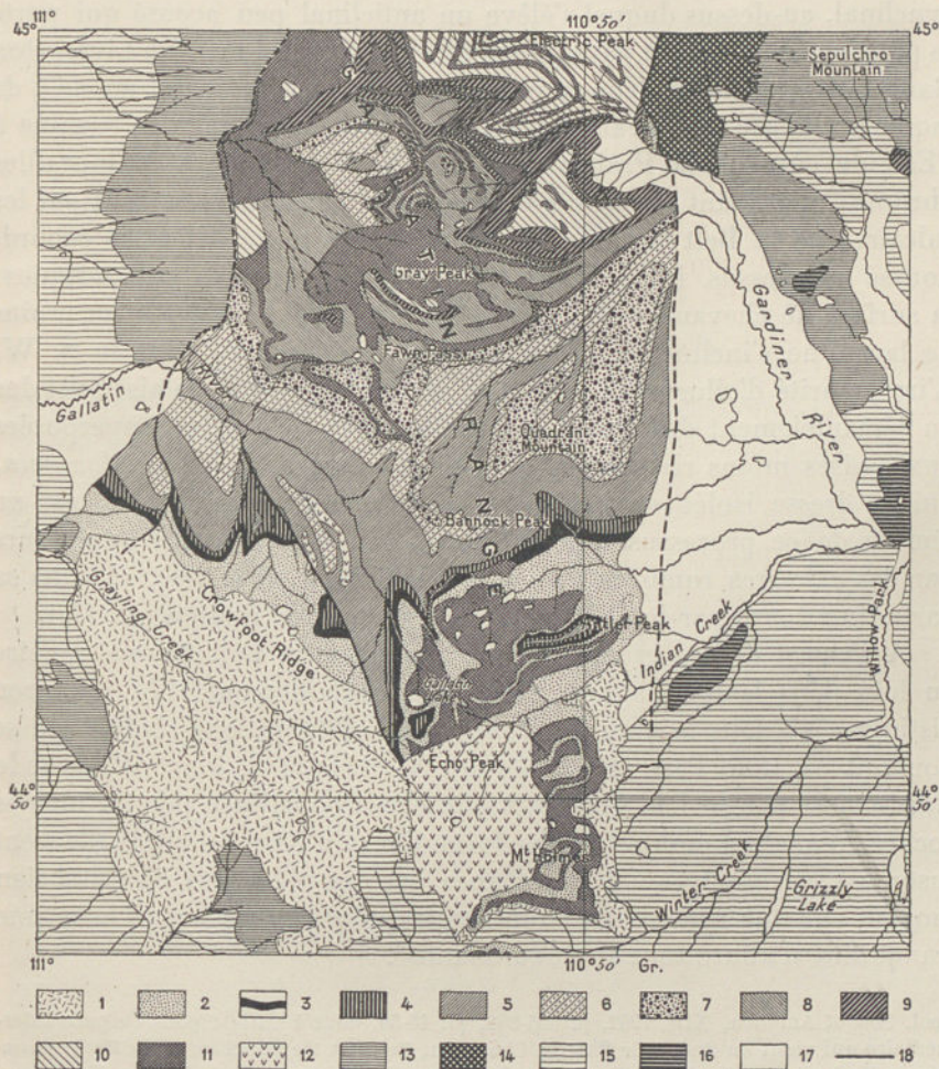
FIG. 263. — Carte géologique du Gallatin Range (Yellowstone National Park), d'après J. P. Iddings et W. H. Weed ( U. S. Geol. Survey, Monograph XXXII, pt. 2, 1899, pl. X ).
