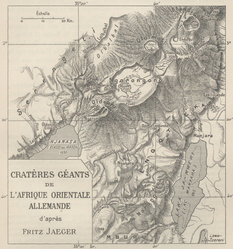
FIG. 220. — Cratères géants de l'Afrique Orientale Allemande, d'après Fr. Jaeger (Mitteil. aus den Deutschen Schutzgebieten, Ergänzungsheft N° 2, carte I, 1911). Échelle de 1 : 900 000.
