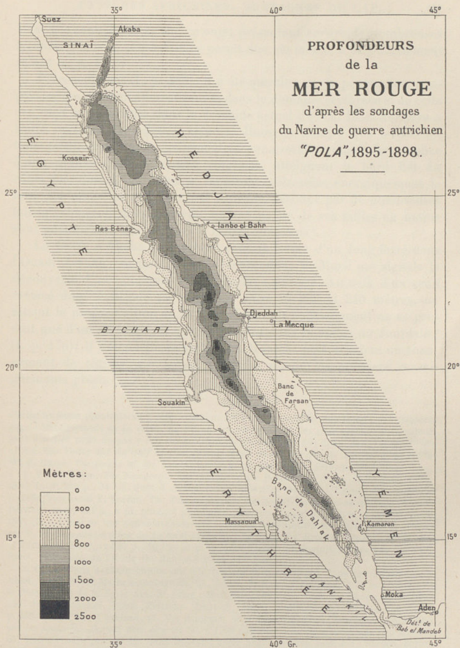
FIG. 223. — Carte bathymétrique de la Mer Rouge, d'après les sondages du navire autrichien « Pola », 1895-1898 ( Denkschriften der Kaiserl. Akademie der Wissenschaften Wien, Mathem.-Naturwiss. Cl. , LXV, 1898, p. 422, et LXIX, 1901, p. 398).
