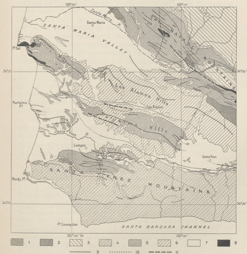
FIG. 278. — Croquis tectonique d'une partie des Chaînes tertiaires du Sud de la Californie, d'après R. Arnold et R. Anderson ( U. S. Geol. Survey, Bulletin 317, 1907, pl. 1 ).
