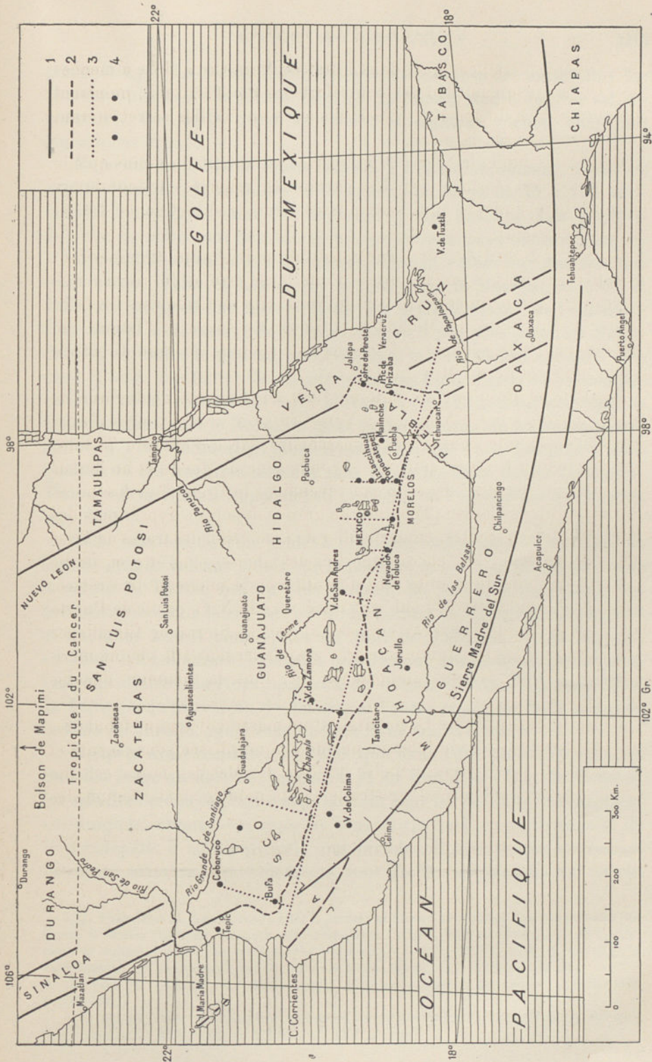
FIG. 286. — Traits généraux de l'orographie du Mexique Central, d'après J. Felix et H. Lenk (Zeitschr. Deutsch. Geol. Gesellschaft., XLIV, 1892, pl. XIX).
