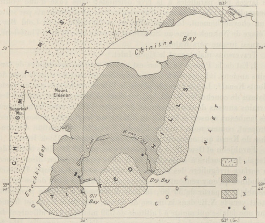
FIG. 253. — La Région pétrolifère du Cook Inlet (Alaska), d'après G. C. Martin (U. S. Geol. Survey, Bull. n° 250, 1905, pl. IV).
