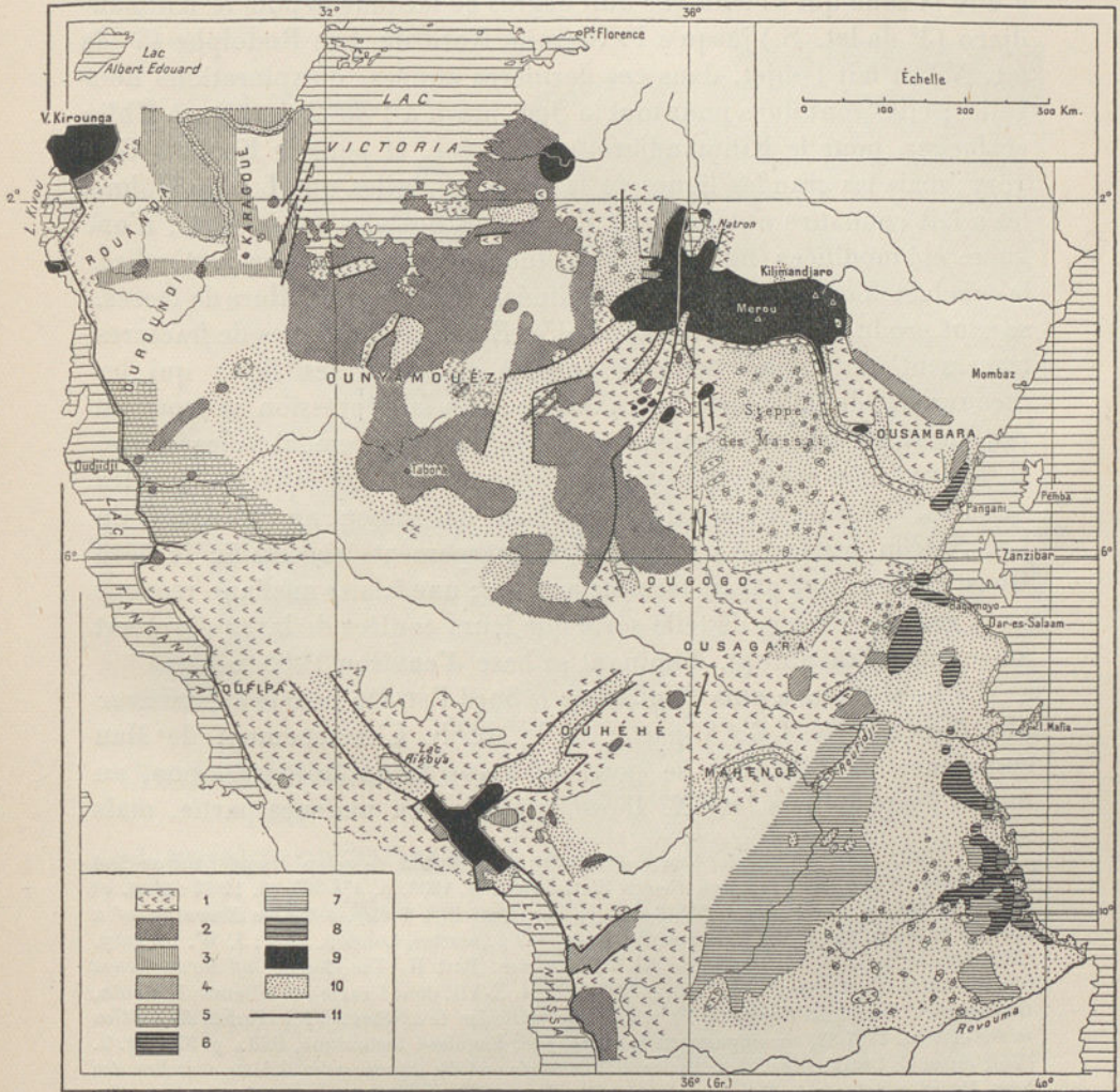
FIG. 219. — Carte géologique de l'Afrique Orientale Allemande, d'après Curt Gagel (in H. Meyer, Das Deutsche Kolonialreich , I. Bd. In-8°, Leipzig-Wien, 1909, p. 416).
