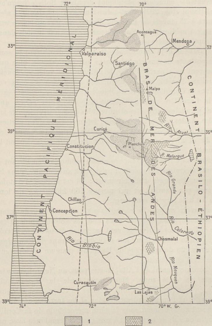
FIG. 297. — Distribution des dépôts jurassiques supérieurs dans les Cordillères Chilo-Argentines, d'après C. Burckhardt ( Beiträge zur Kenntnis der Jura- und Kreideformation der Cordillere ; Palaeontographica , L, 1903, p. 1; Geol. Rundschau , II, 1911, p. 496, fig. 3).
