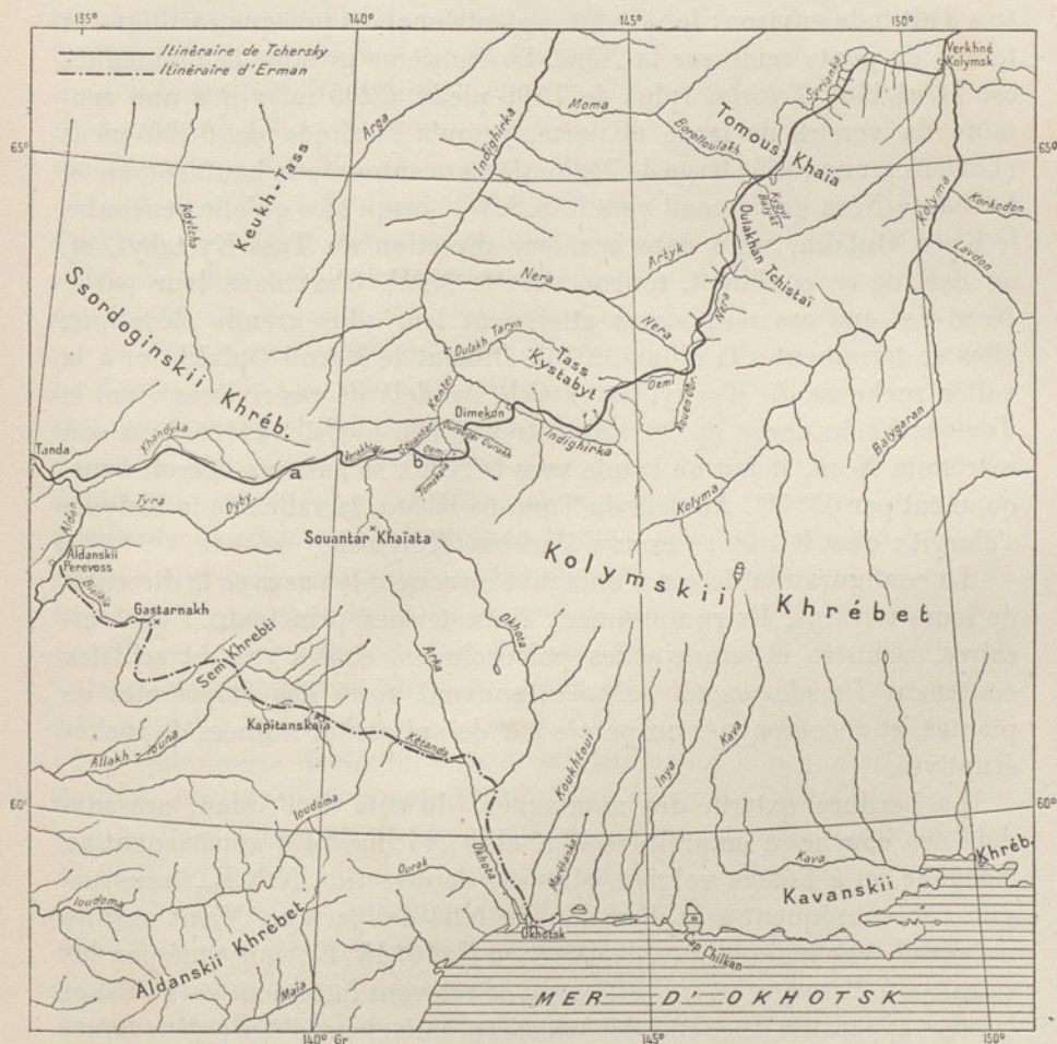
FIG. 242. — Carte de la région des sources de l'Indigirka (Sibérie orientale), d'après la pl. XVIII du tome III de l'édition allemande.
