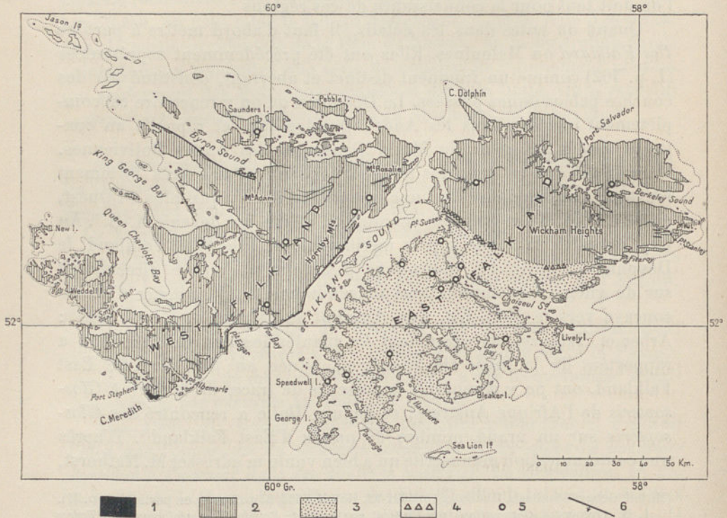
FIG. 306. — Carte géologique des Iles Falkland ou Malouines, d'après Thore G. Halle (Bull. Geol. Inst., University of Upsala, XI, 1910, pl. 10, 1912.)
