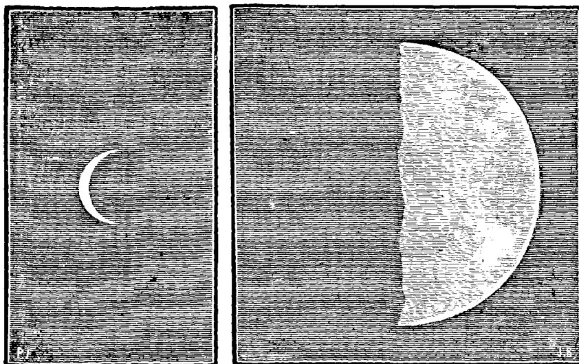
Fig. 113. — La Lune vue à l'œil nu.
