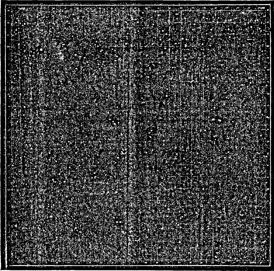
Fig. 234. — Une carte d'étoiles le long de l'écliptique.
