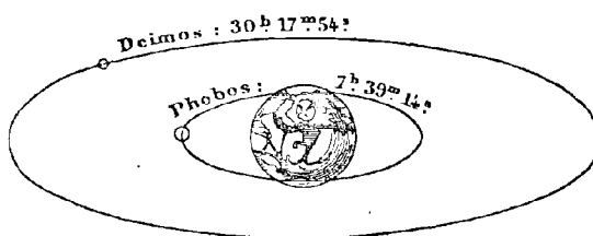
Fig. 74. — Le système de Mars.
