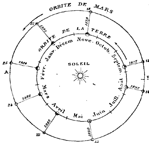
Fig. 40. — Cycle des oppositions de Mars.
