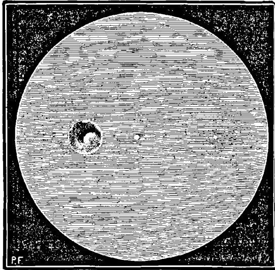
Fig. 73. — Mars et ses deux satellites.
