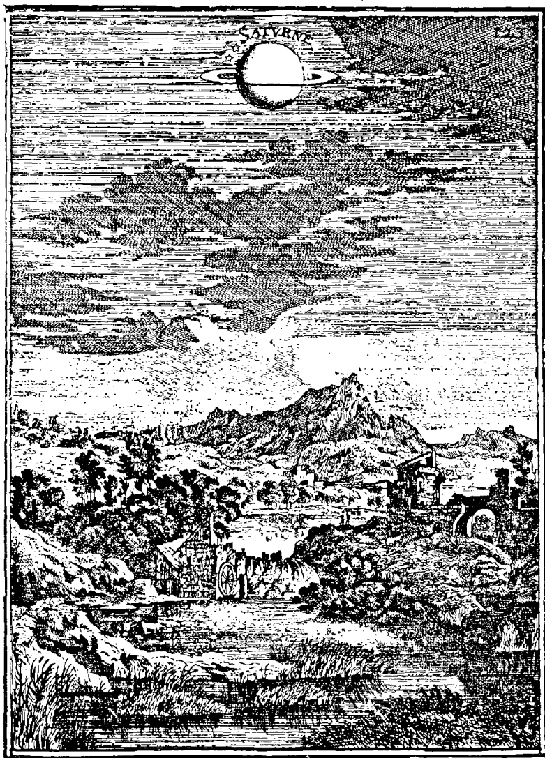
Fig. 292. — L'anneau de Saturne et les perspectives (Figure du XVII e siècle.)
