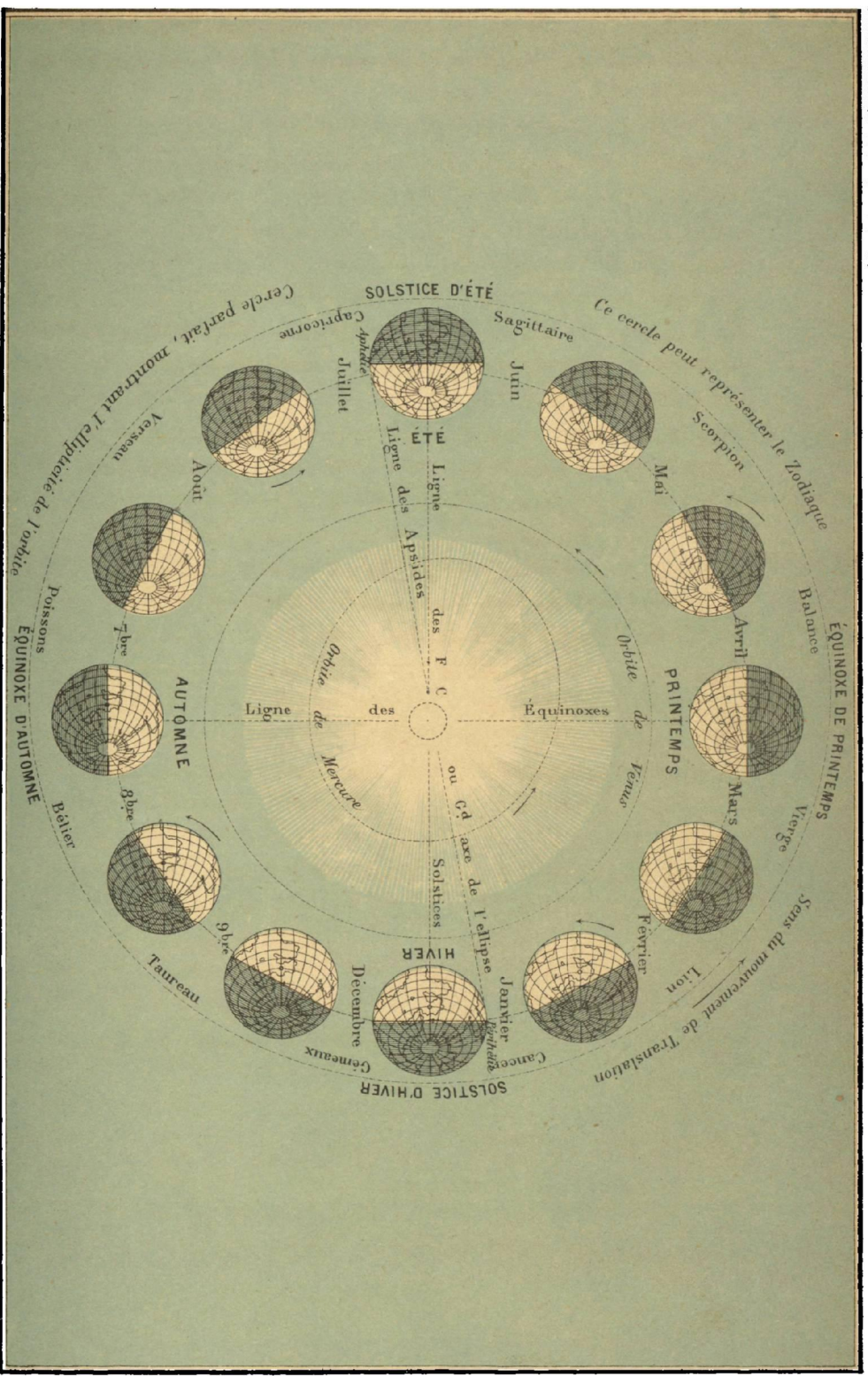
MOUVEMENT ANNUEL DE LA TERRE AUTOUR DU SOLEIL, ET PRODUCTION DES SAISONS.
