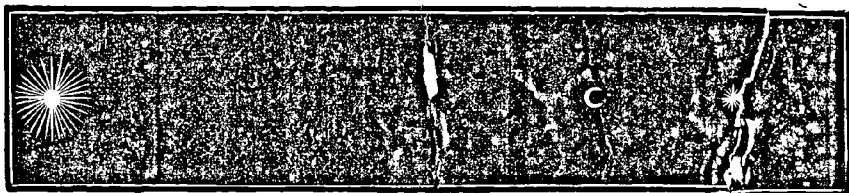
Fig. 112. — Le Soleil, la Lune et Vénus vus à l'œil nu, le 4 février 1883.
