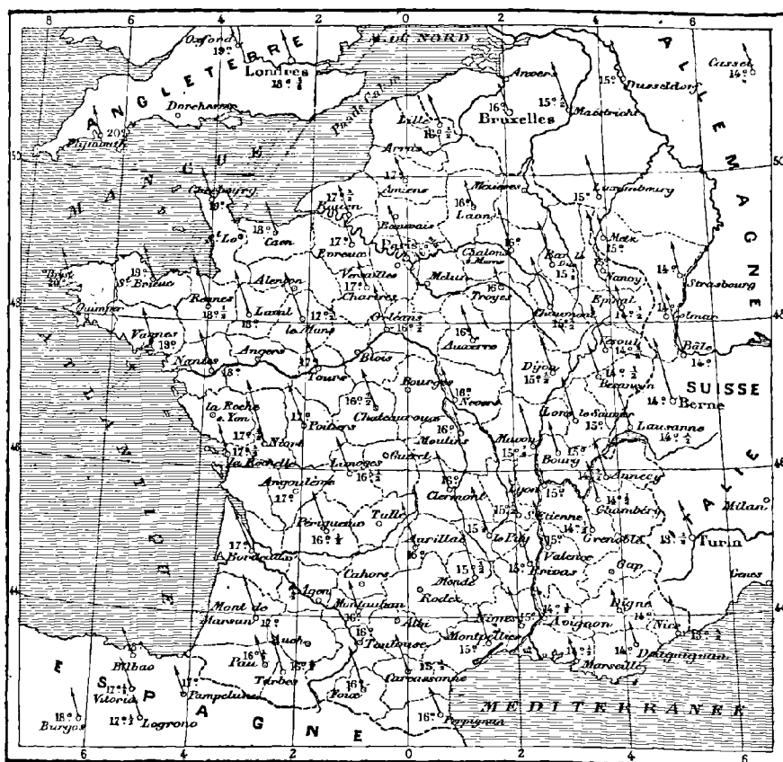
Fig. 189. — Déclinaison de l'aiguille aimantée.
