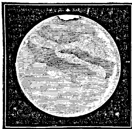
Fig 39. — Voile atmosphérique sur le contour intérieure de la planète.
