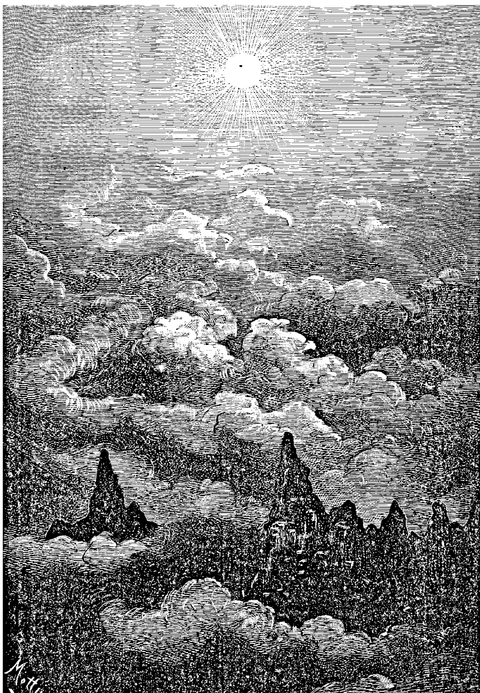
Vue de Jupiter, notre Terre n'est qu'un minuscule point noir devant le Soleil.
