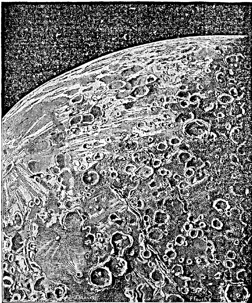
Fig. 204. — Région montagneuse au sud de la mer de la Fécondité.
