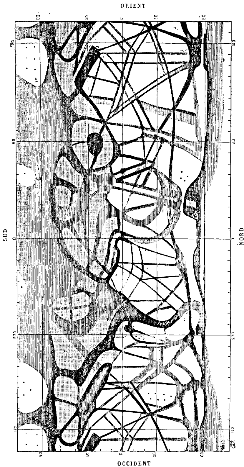
Fig. 30. -- Canaux énigmatiques observés sur la planète Mars. (Dessin de M. SCHIAPARELLI.) (Aux points signalés par de petits cercles 0000, on a vu des taches blanches comme de la neige.)
