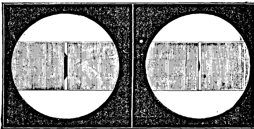
Fig. 135. — Expérience spectroscopique pendant le passage de Vénus devant le Soleil.
