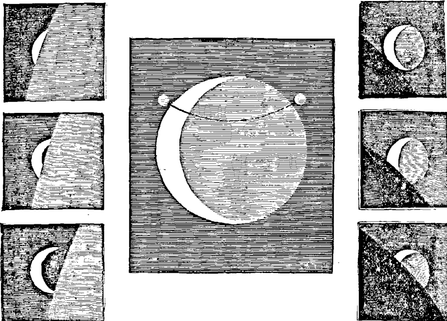
Fig. 108. — Occultation de Vénus par la Lune, le 14 octobre 1874.)
