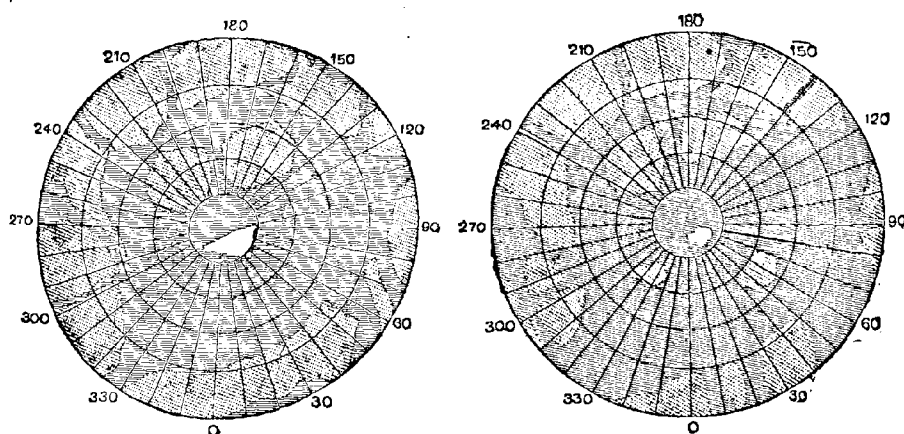
Fig. 54. — Neiges polaires de Mars après l'été : 1877 et 1879.
