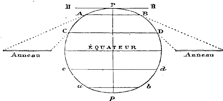
Fig. 303. — Coupe géométrique à travers Saturne et ses anneaux.
