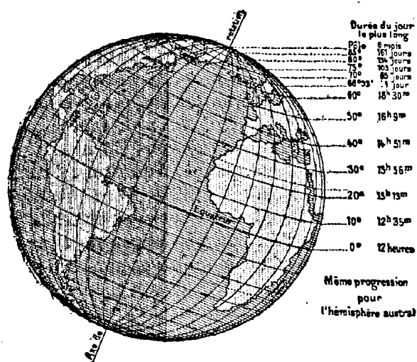
Fig. 181. — La Terre au solstice de juin : durée du jour selon les latitudes.
