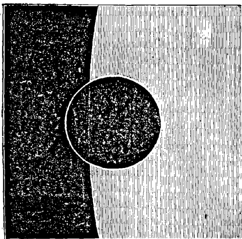
Fig. 137. — L'auréole atmosphérique de Vénus (Orgères, 6 décembre 1882).
