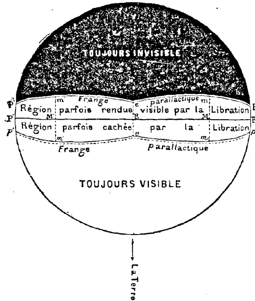
Fig. 198. — Étendue du globe lunaire que nous connaissons.
