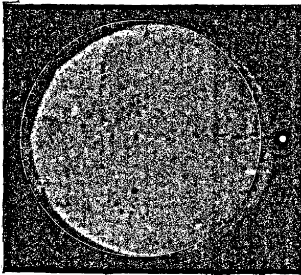
Fig. 322. — Grandeur comparée du Soleil vu de la Terre et vu de Neptune.
