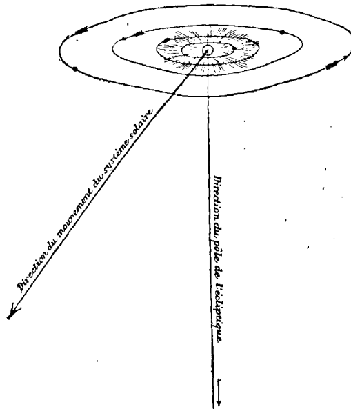
Fig. 184. — Chute du système solaire dans l'espace.
