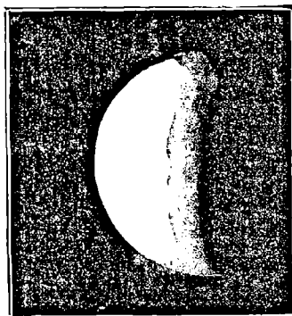
Fig. 164. Phase de Mercure. Troncature de la corne australe.
