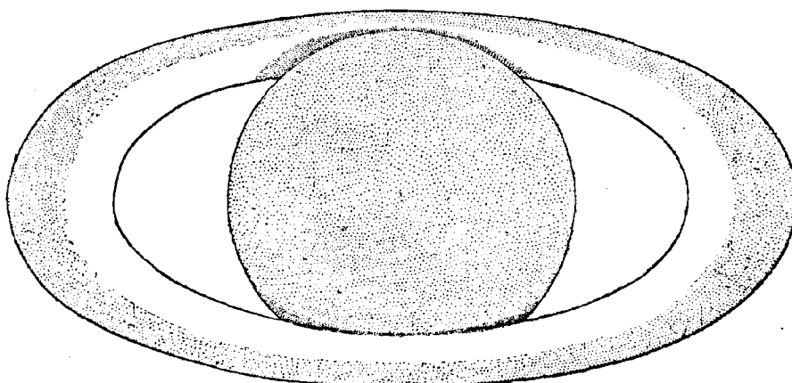
Fig. 289. — Premier dessin du double anneau de Saturne, CAMPANI, 1664.
