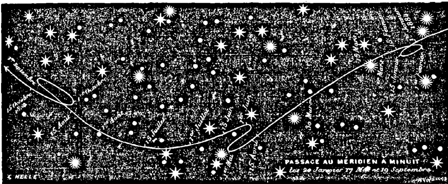
Fig. 176. — Marche de la planète Terre dans le ciel des habitants de Mercure.
