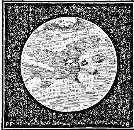
Fig. 28. — Aspect de Mars le 2 septembre 1877 (1 h 40 m du matin).
