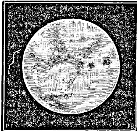
Fig. 29 — Aspect de Mars le 24 octobre 1879 (2 h du matin).
