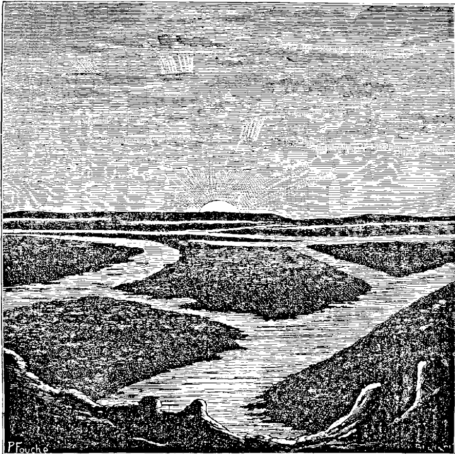
Fig. 31. — Le lever du soleil sur les canaux de Mars.
