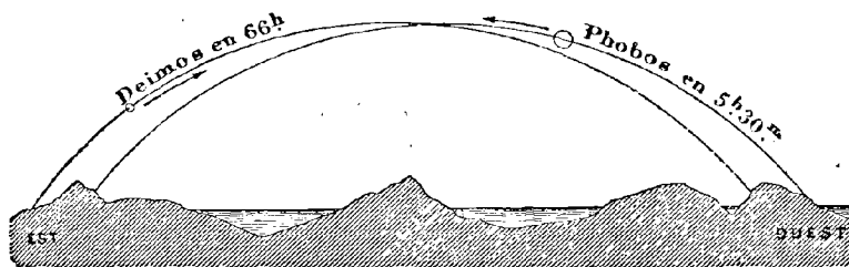
Fig. 70. — Marche des satellites de Mars dans le ciel de leur planète.
