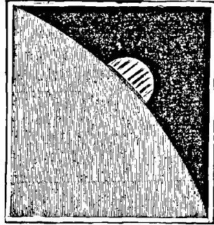
Fig. 247. — Occultation de Jupiter par la Lune, le 24 mai 1860.
