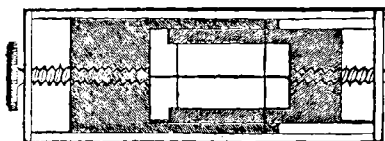
Fig. 145. — Mécanisme du micromètre.
