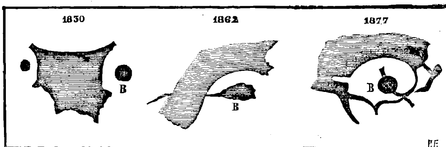
Fig. 25. — Variations produites dans les mers de Mars. La mer Terby en 1830, 1862 et 1877.
