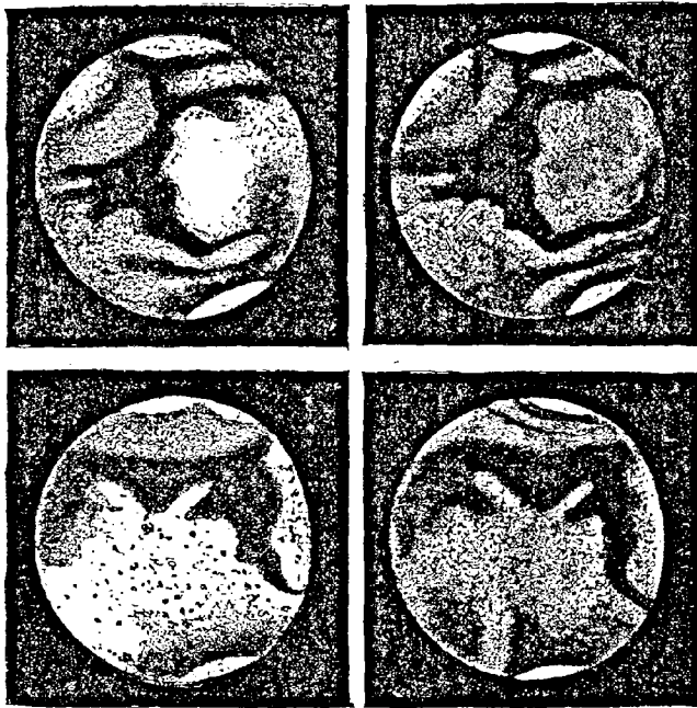
Fig. 13. — Aspects de Mars les 13, 14, 17 et 18 juin 1858.
