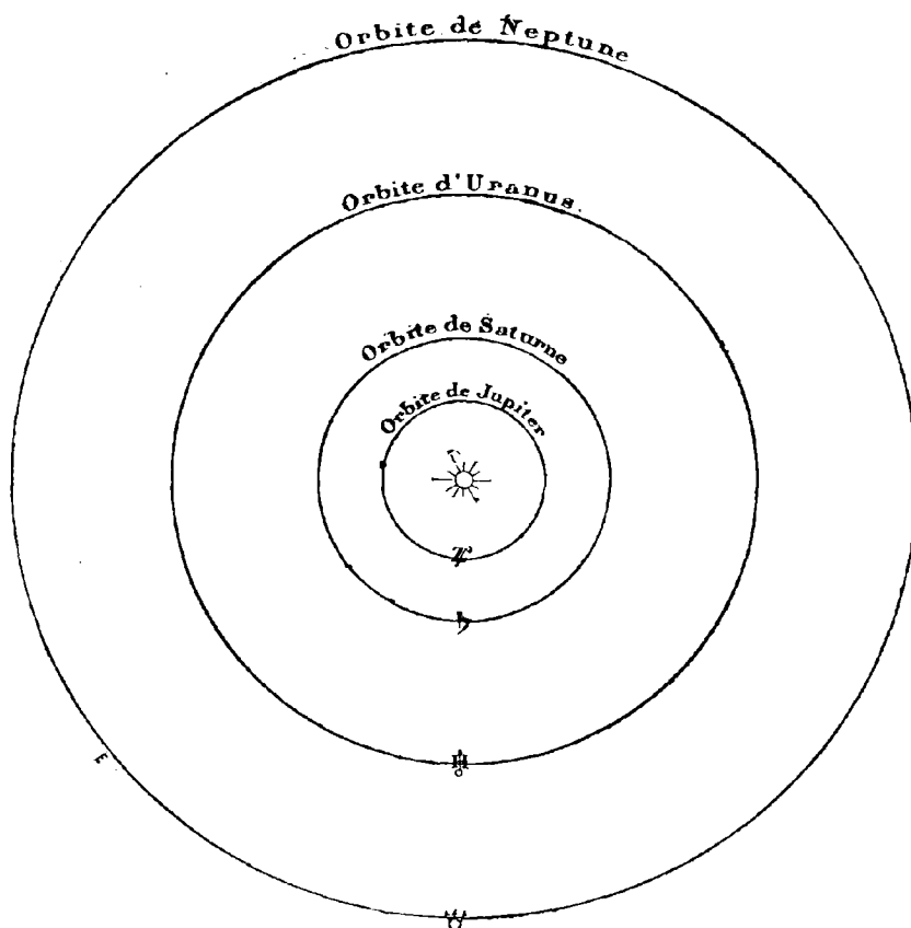
Fig. 320. — Les mondes principaux du système solaire.
