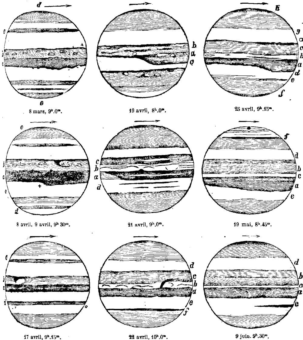
Fig. 249. — Vues télescopiques de Jupiter prises en 1874.
