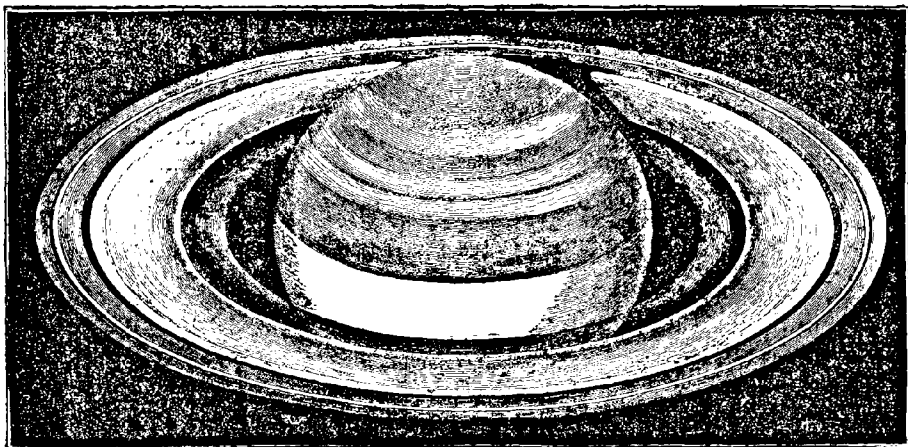
Fig. 284. — Saturne et ses anneaux.
