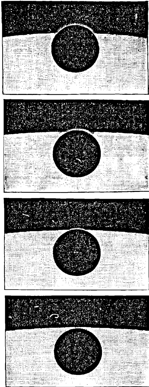
Fig. 133. — L'auréole atmosphérique de Vénus (Postdam, 6 décembre 1882).
