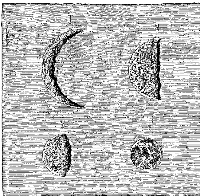
Fig. 117. — Inégalités observées sur la planète Vénus.
