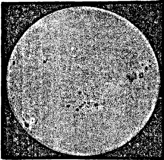
Fig. 106. — Aspect des taches solaires.
