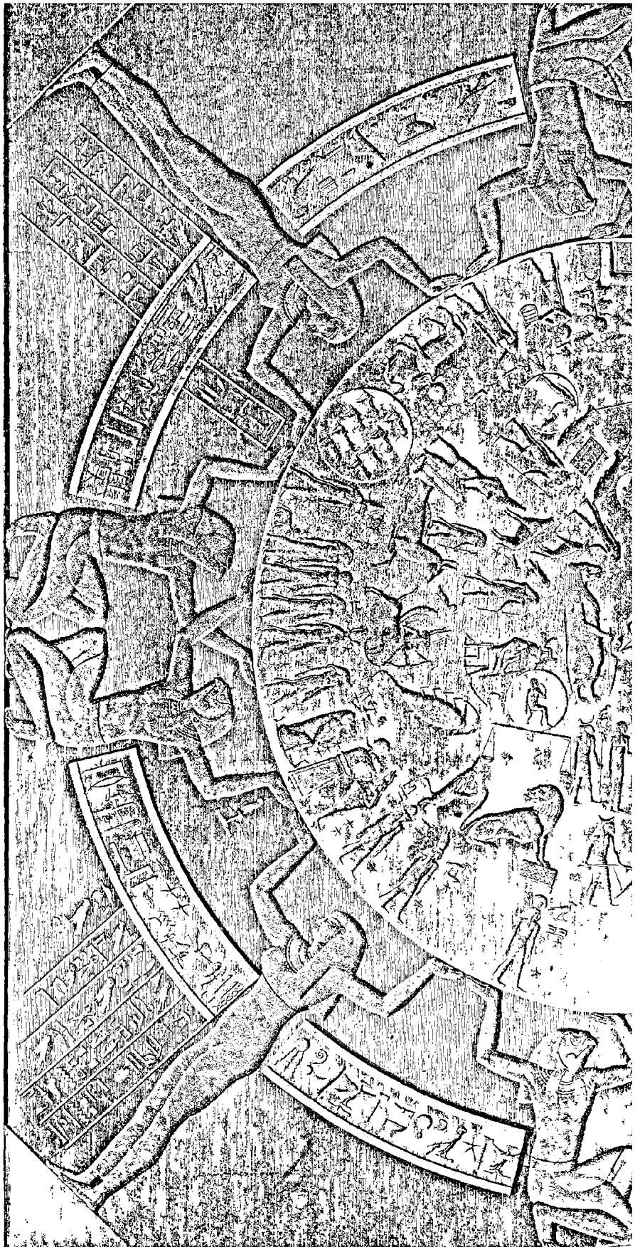
Fig. 239. — ZODIAQUE DE DENDÉRAH : Balance. — Scorpion. — Sagittaire. — Capricorne. — Verséau. — Poissons
