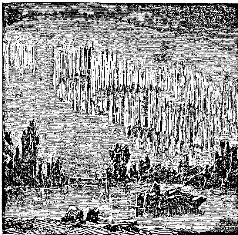
Fig. 190. — Une aurore boréale.
