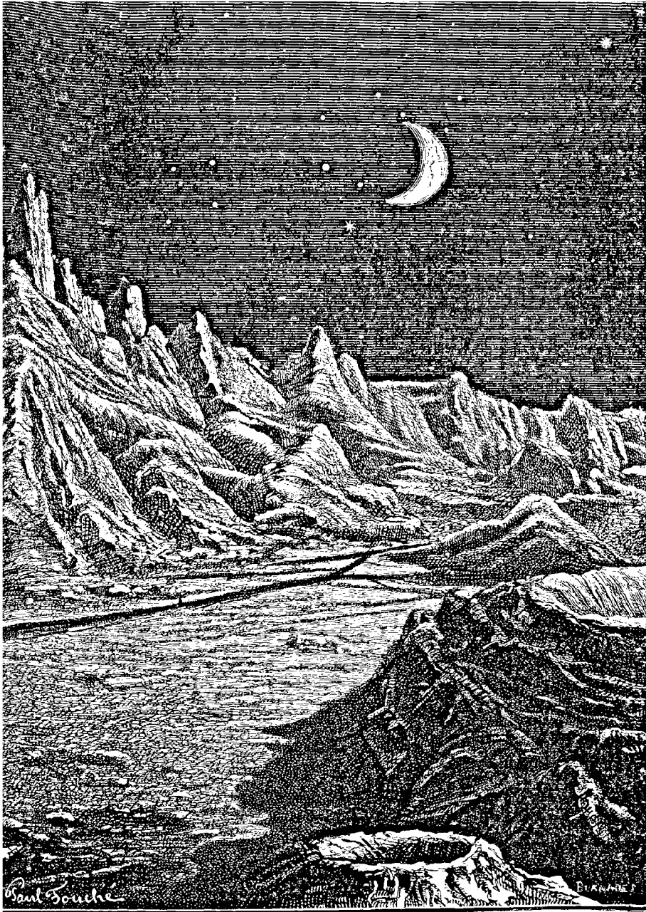
Phases de la Terre vue de la Lune.
