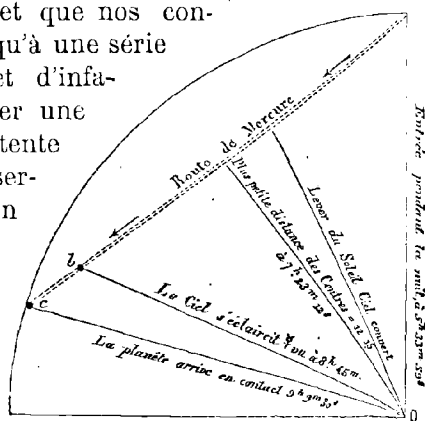
Fig. 134. — Quart nord-ouest du Soleil montrant la route suivie par Mercure devant le Soleil.
