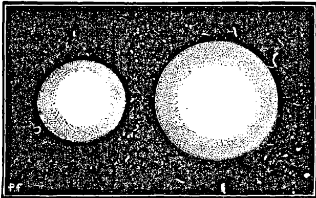
Fig. 51. — Grandeur comparée du Soleil vu de Mars et vu de la Terre.
