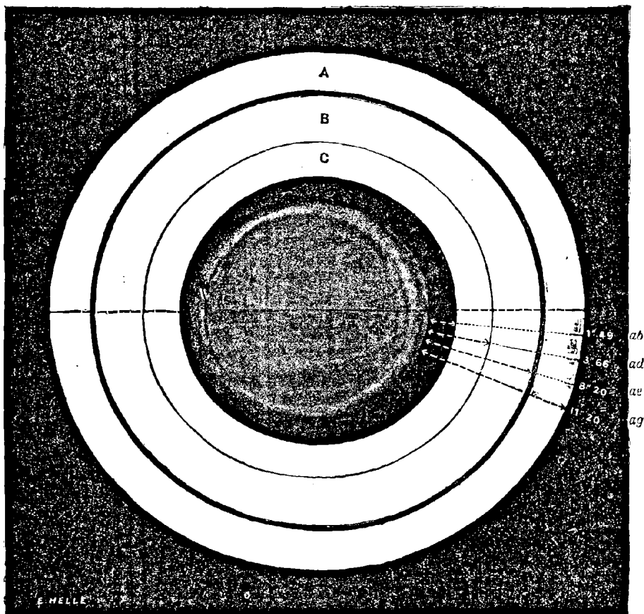
Fig. 295. — Le système de Saturne (mesures de M. Struve, 1832).
