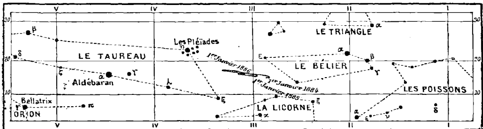
Fig 269. — Mouvement et positions des planètes Jupiter, Saturne, Uranus et Neptune pendant deux années (1884 et 1885).
