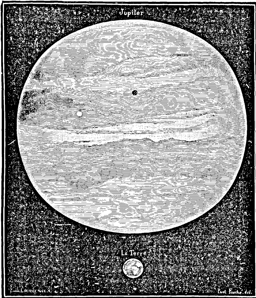
Fig. 240. — Grandeur comparée de Jupiter et de la Terre.
