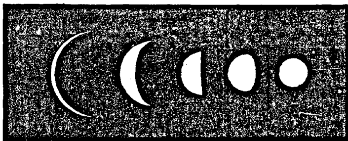
Fig. 163. — Les phases de Mercure.
