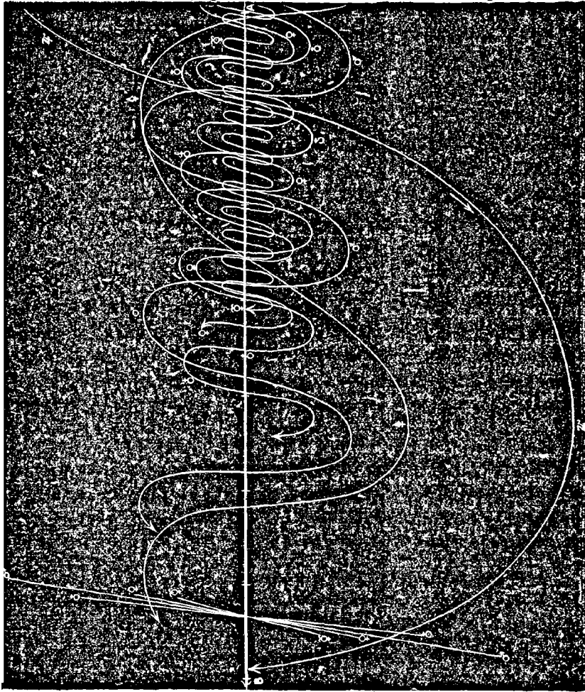
Fig. 183. — Hélices parcourues par Jupiter, Vesta, Mars, la Terre, Vénus et Mercure, dans leur mouvement annuel autour du Soleil.
