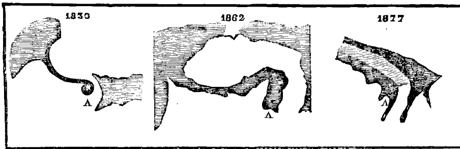
Fig. 24. — Variations probables dans les mers de Mars. Le golfe Kaiser et la Baie du Méridien en 1830, 1862 et 1877.
