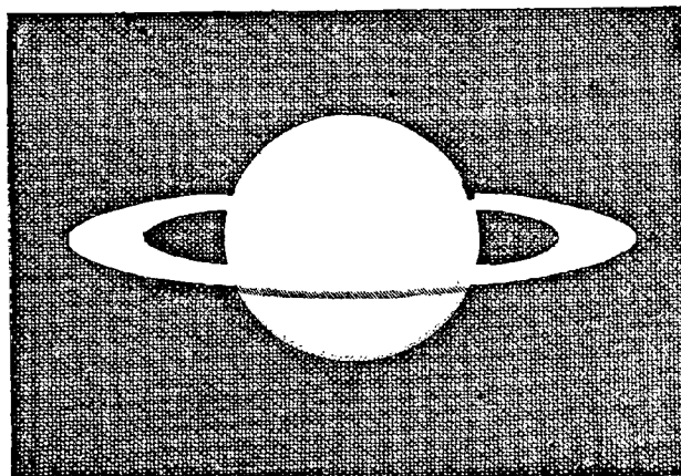
Fig. 287. — Premiers dessins de l'anneau de Saturne : HUYGENS 1657.
