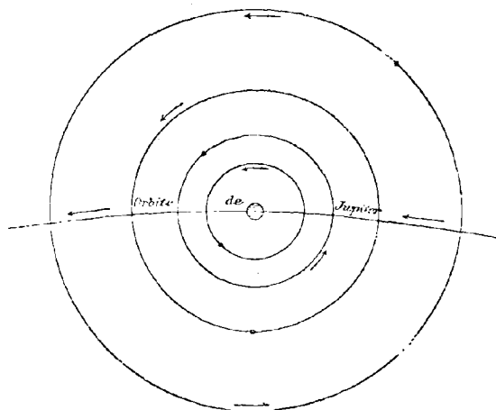
Fig. 264. — Le système de Jupiter.
