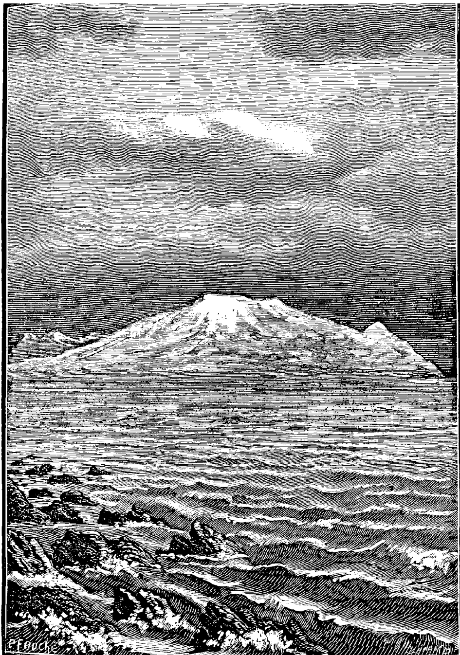
L'île neigeuse vue de l'océan Képler : météorologie martienne.
