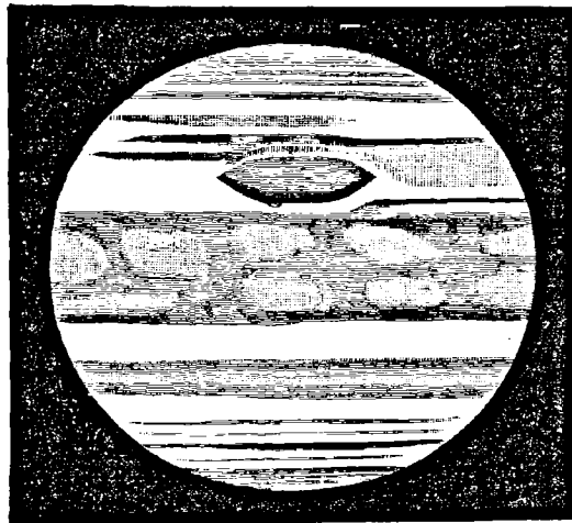
Fig. 251. — Aspect de Jupiter le 7 décembre 1881.
