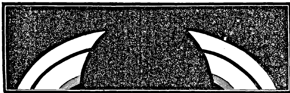
Fig. 307. — Les anneaux de Saturne et l'ombre de la planète
