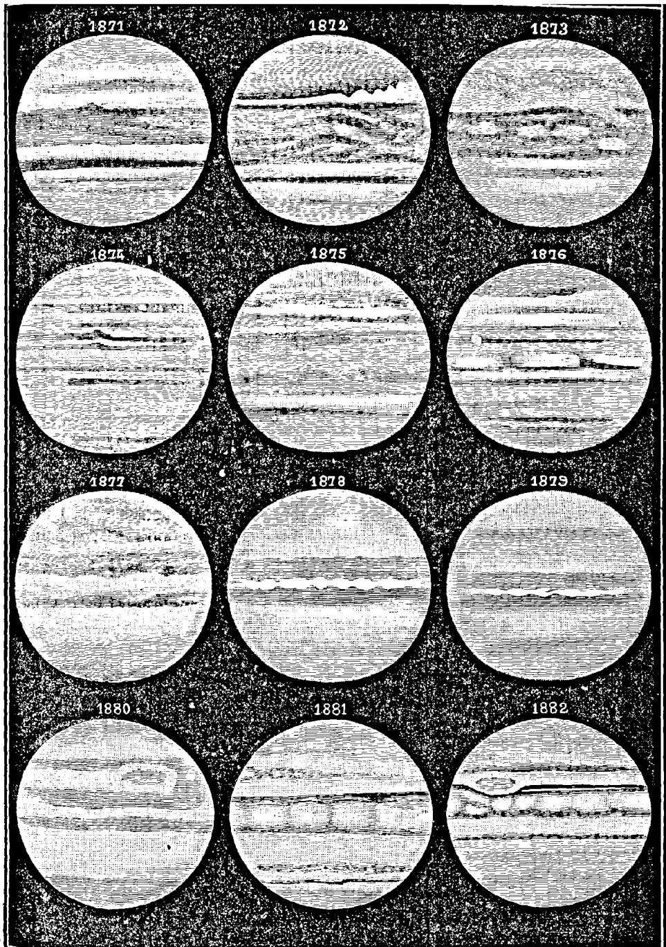
Fig. 254. — Aspect télescopique de Jupiter pendant douze ans.
