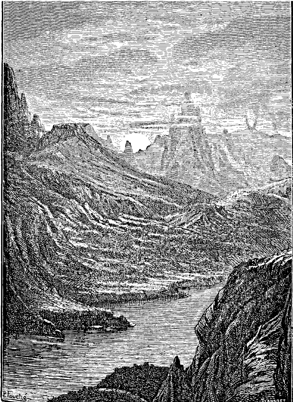
TERRES DU CIEL Les montagnes de Vénus, au lever du soleil.
