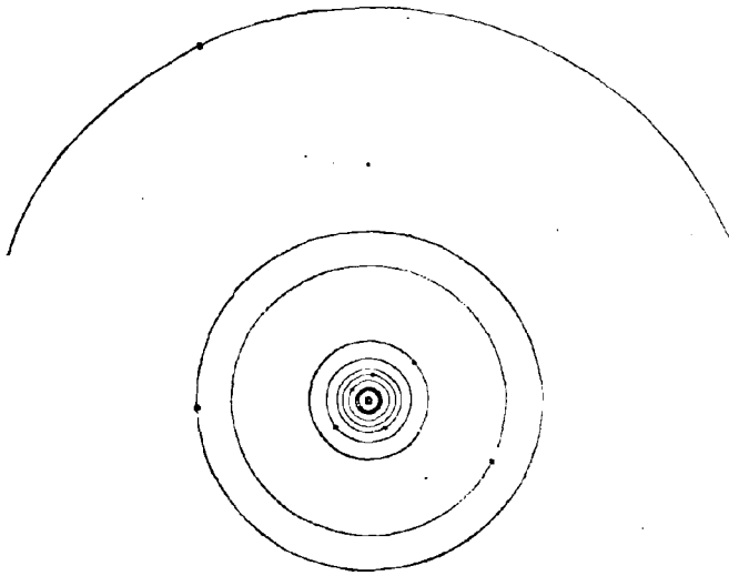
Fig. 300. — Le système de Saturne.
