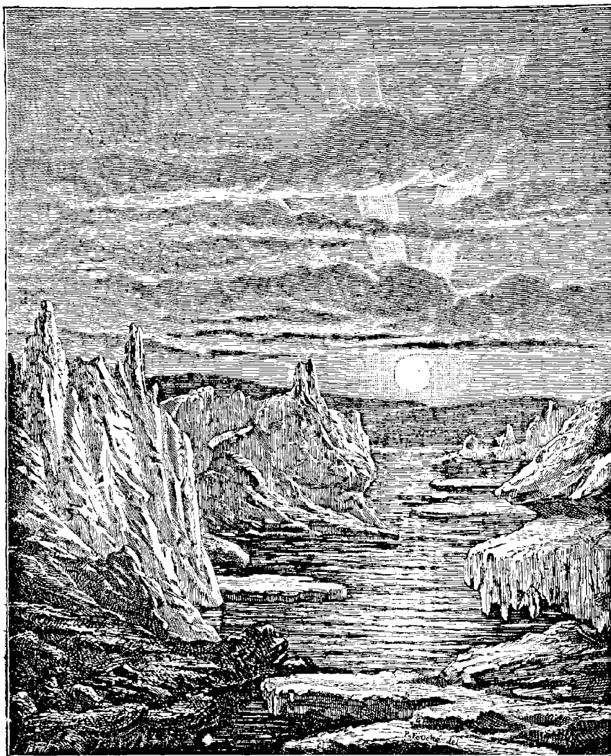
Fig. 53. — Le soleil de minuit sur la planète Mars.
