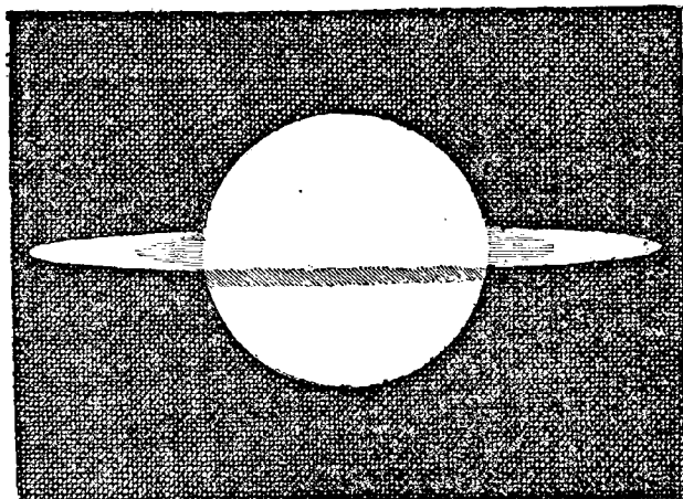
Fig. 286. — Premiers dessins de l'anneau de Saturne : HUYGENS 1636.
