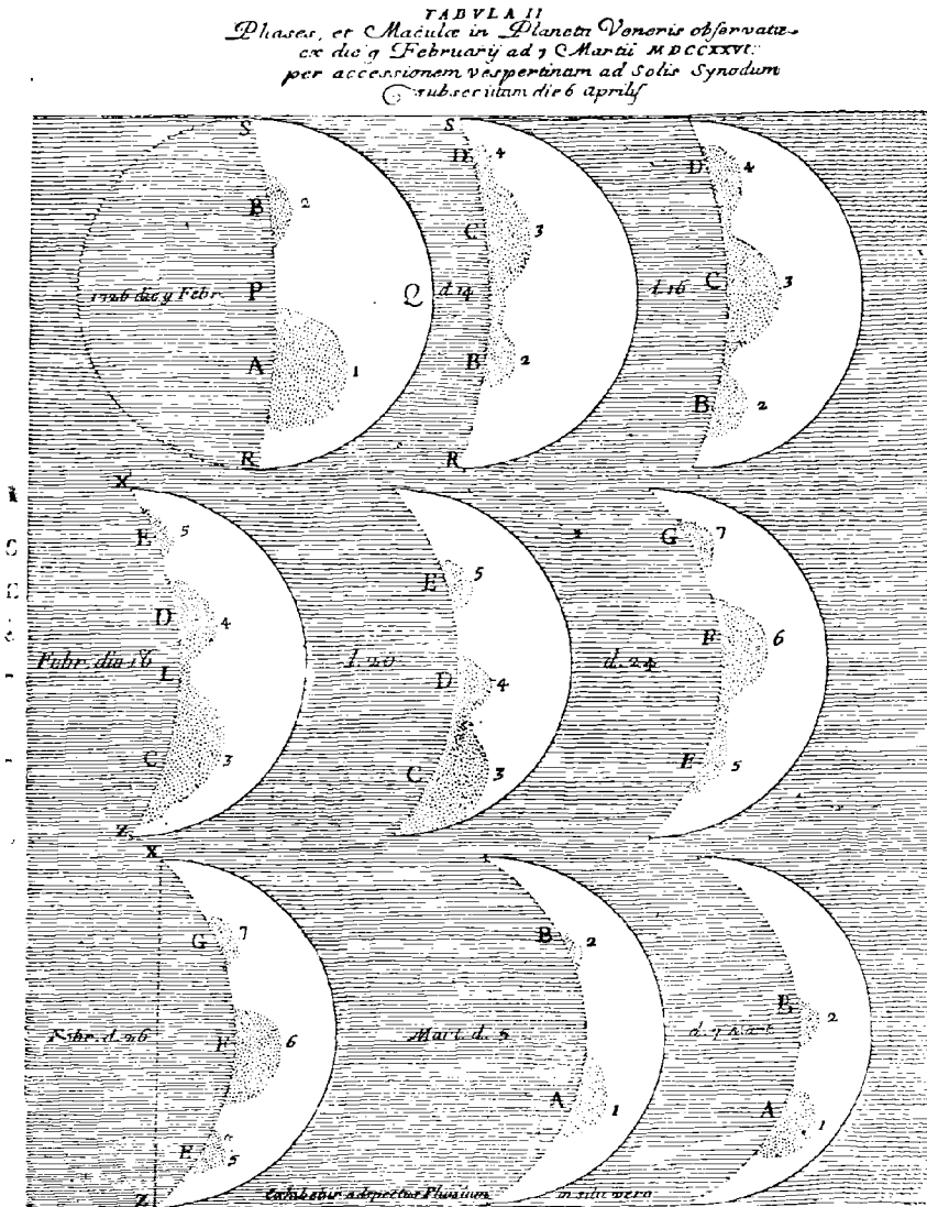
Fig. 121. — Dessins de la planète Vénus faits en 1726-1727, par Bianchini, à l'aide d'une lunette de 30 mètres.
