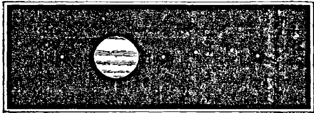
Fig. 262. — Jupiter et ses quatre satellites.
