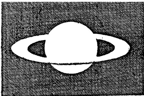
Fig. 188. — Premiers dessins de l'anneau de Saturne . HUYGENS 1659.
