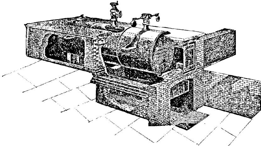
Fig. 43. — Chaudière Galloway multitubulaire.
