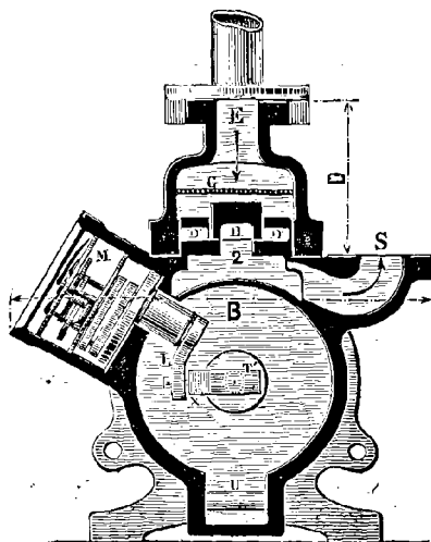
Fig. 497. — Compteur Samain.
