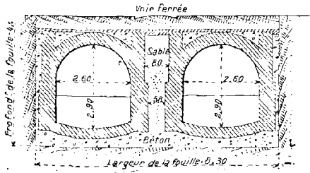
Fig. 41. — Coupe, type n° 3.
