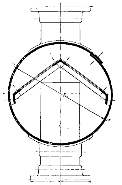
Fig. 90. — Collecteur de vapeur. Coupe transversale.
