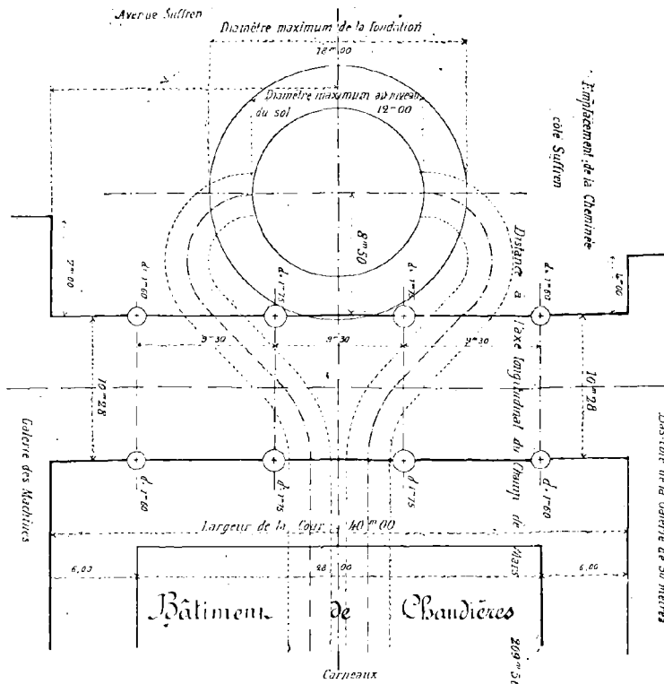
Fig. 17. — Disposition des carreaux à la base de la cheminée Sulfren.
