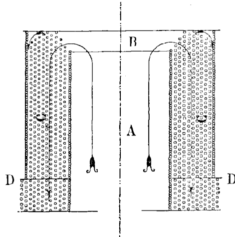
Fig. 406. — Chaudière Du Temple-Guyot.
