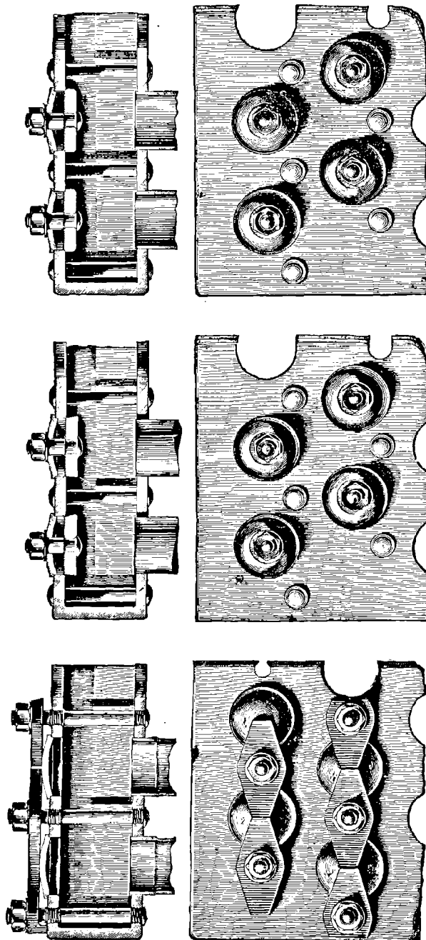
Fig. 80. — Générateur Steinmüller. — Fermeture des chambres à eau.
