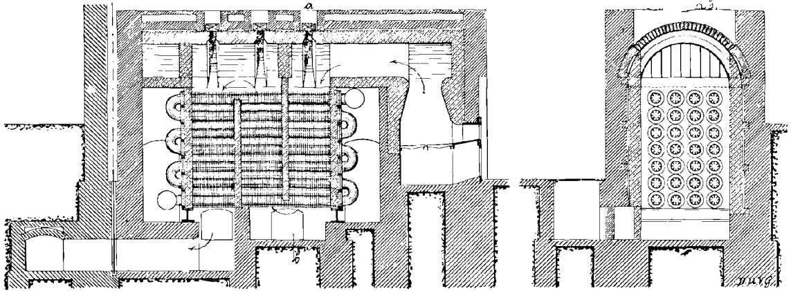
Fig. 148. — Surchauffeur Schwærer.
