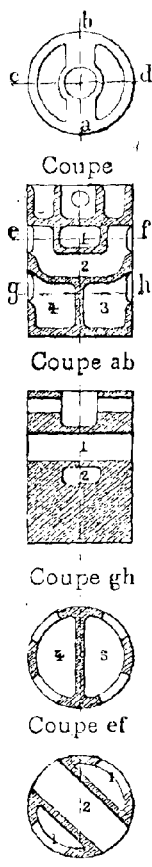
Fig. 195. Détails des pistons
