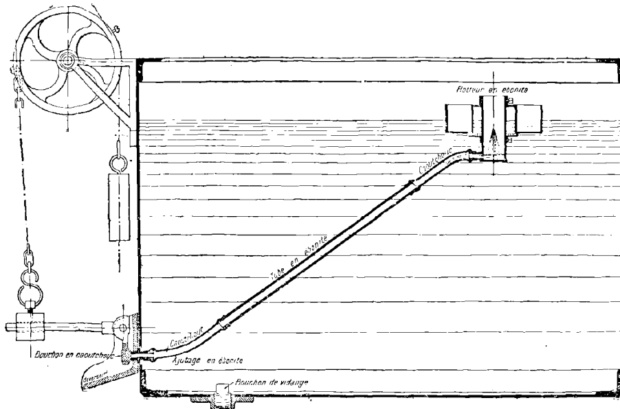
Fig. 185. — Réservoir à réactifs.
