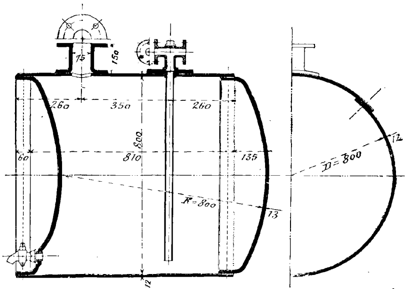
Fig. 87. — Bouteille de purge.
