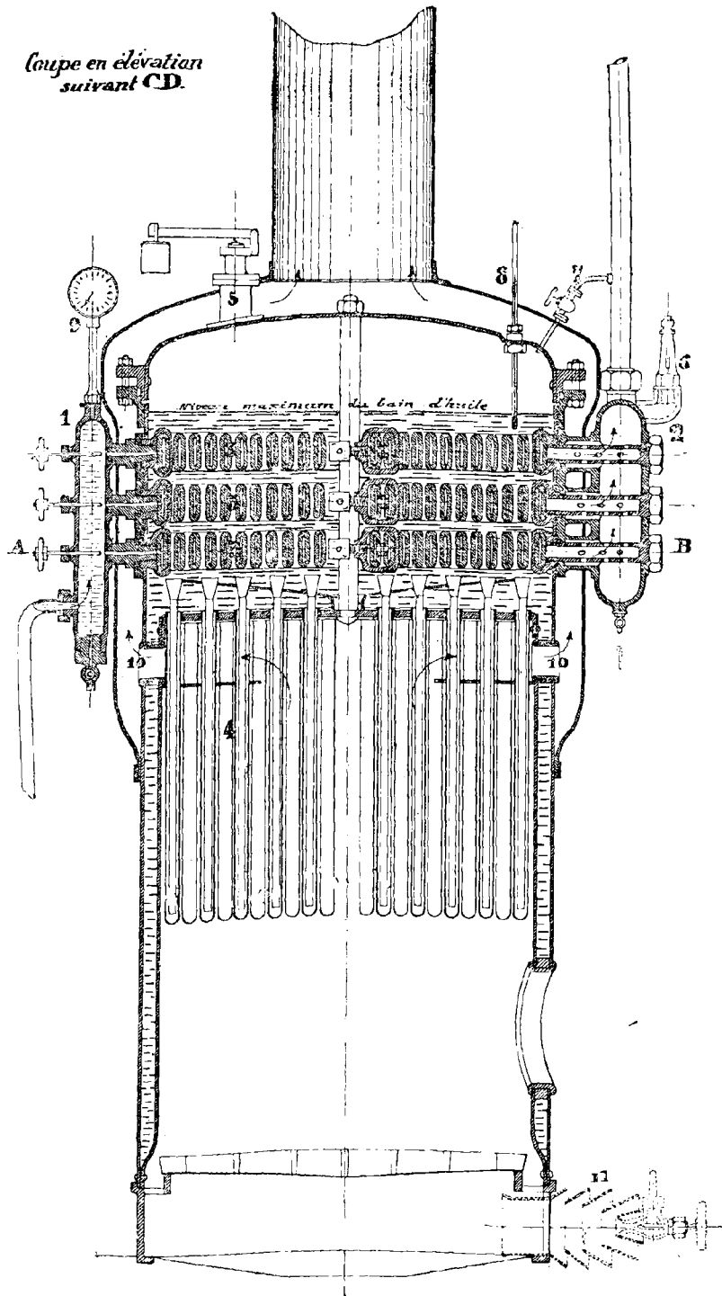
Fig. 148.
