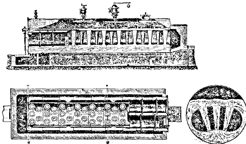
Fig. 36. — Chaudière Galloway (type normal).
