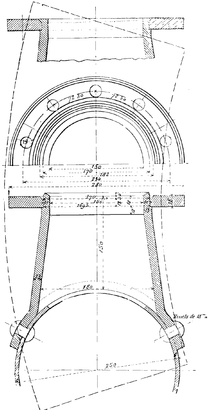
Fig. 84. — Tubulure de tuyau de 0 m ,250.
