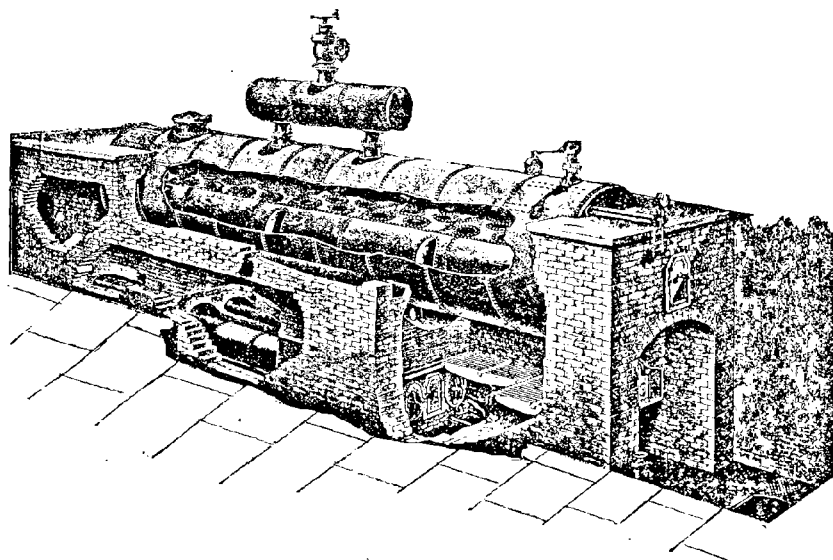
Fig. 39. — Chaudière Galloway avec foyer extérieur.
