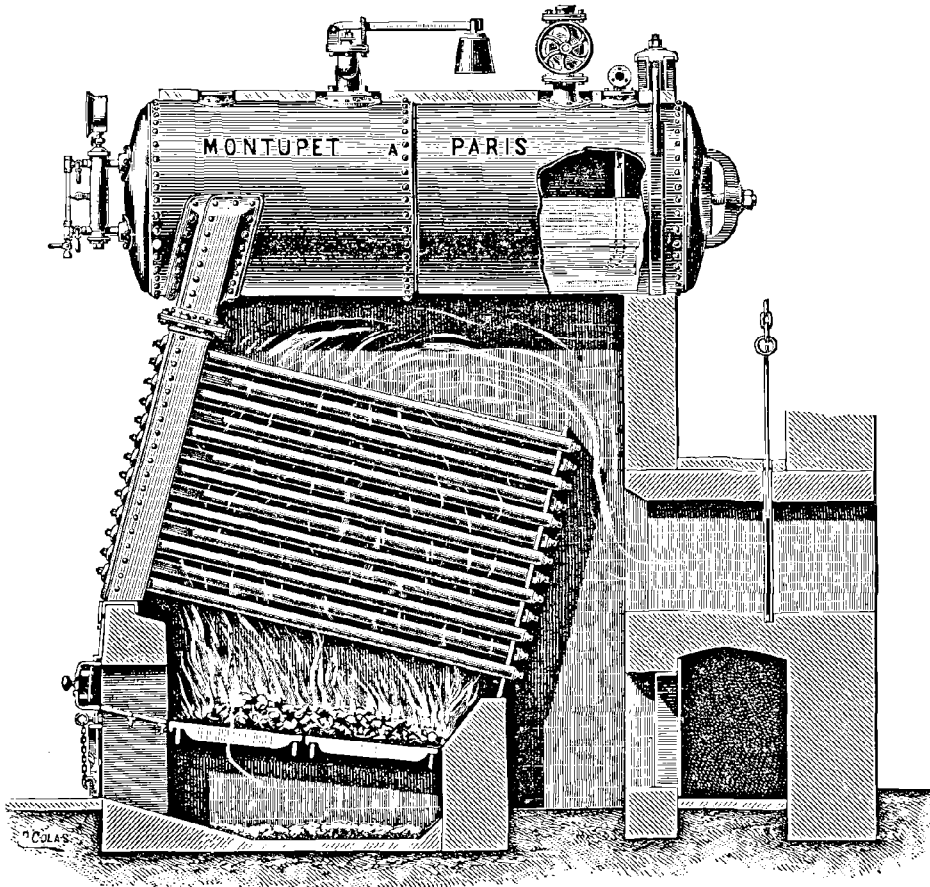
Fig. 51. — Type industriel, variante N° 3.
