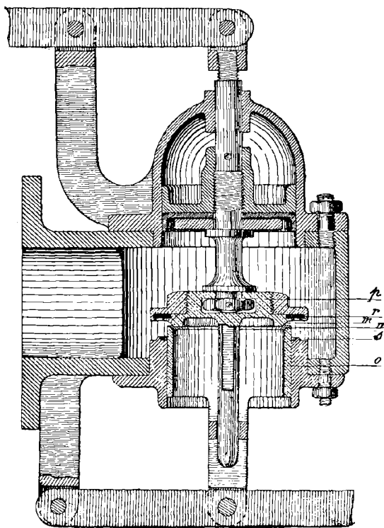
Fig. 192. — Soupape équilibrée.
