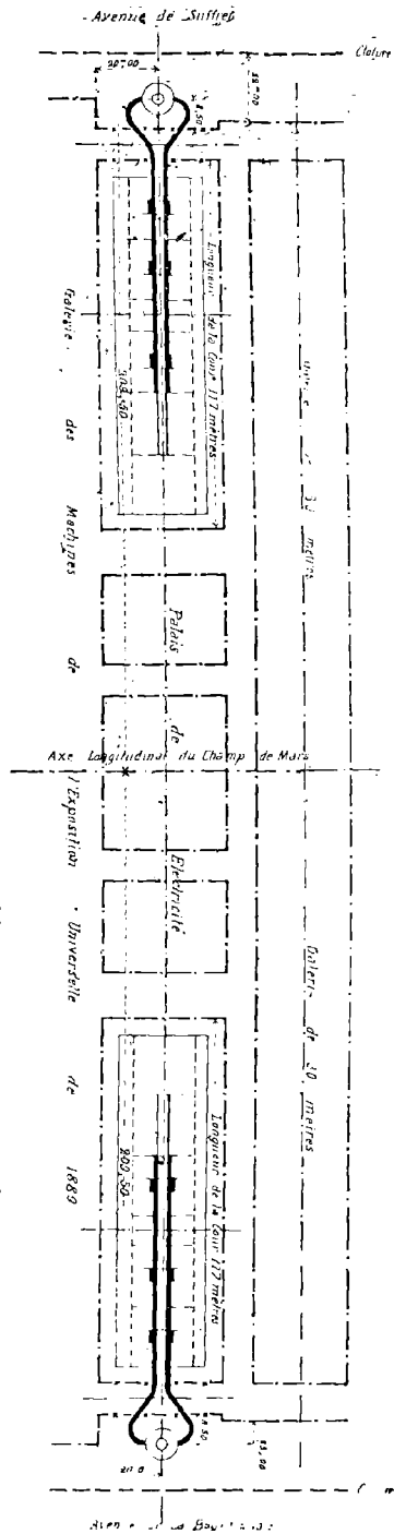
Fig. 1. — Disposition d'ensemble des carreaux de fumée aux Usines Suffren et La Bourdonnais.
