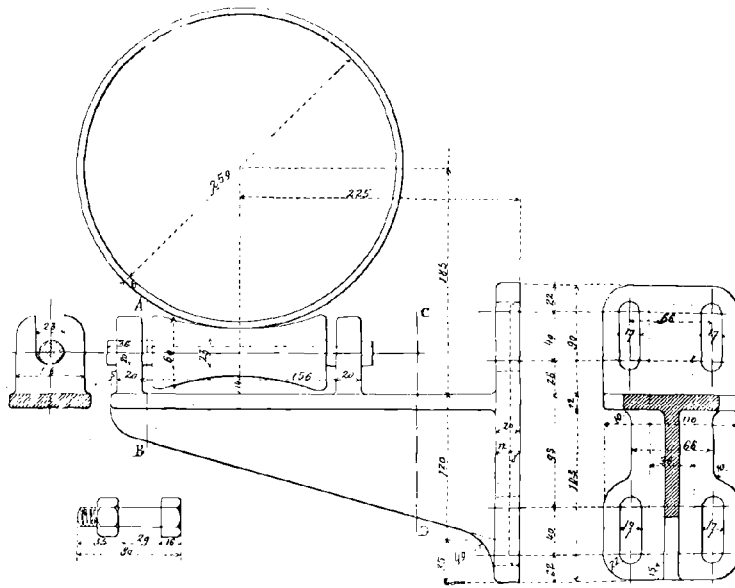
Fig. 83. — Support à une branche pour tuyau de 0 m ,250.
