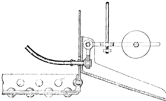
Fig. 187. — Flotteur-régulateur (Détails).
