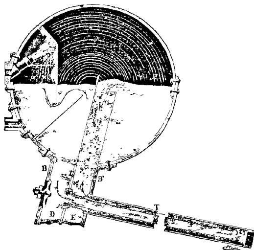
Fig. 47. — Chaudière Montupet.
