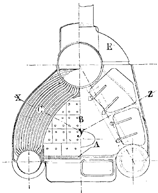
Fig. 105. — Chaudière Du Temple-Guyot.
