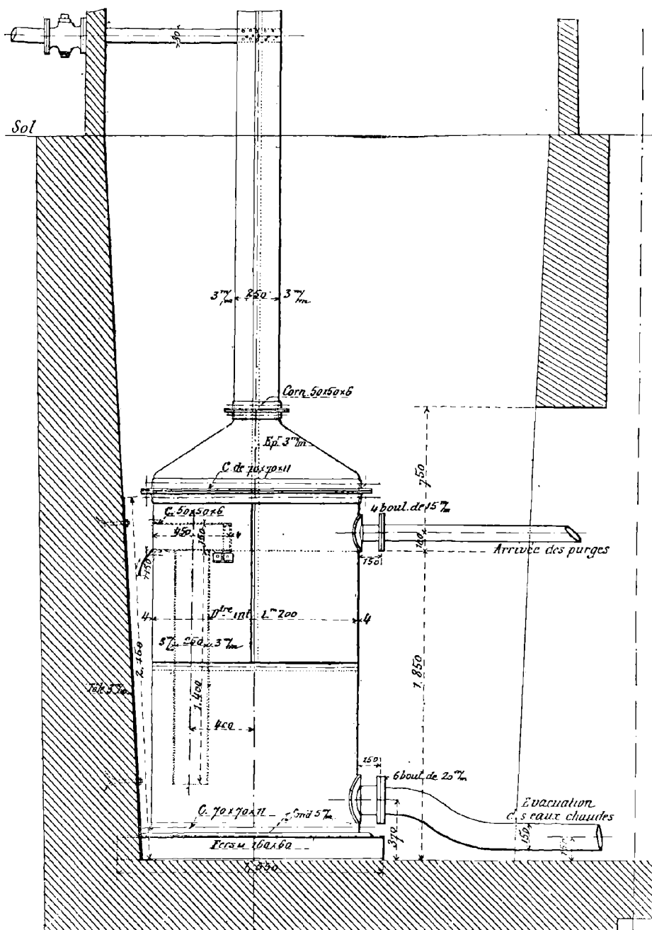
Fig. 99. — Vase d'expansion des purges.
