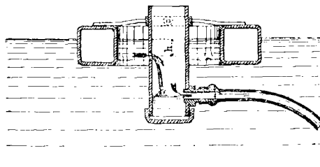
Fig. 186. — Flotteur-régulateur (détails).
