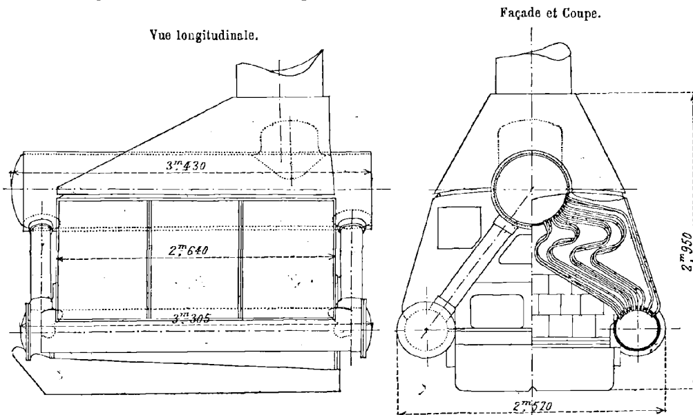
Fig. 103. — Chaudière Du Temple.
