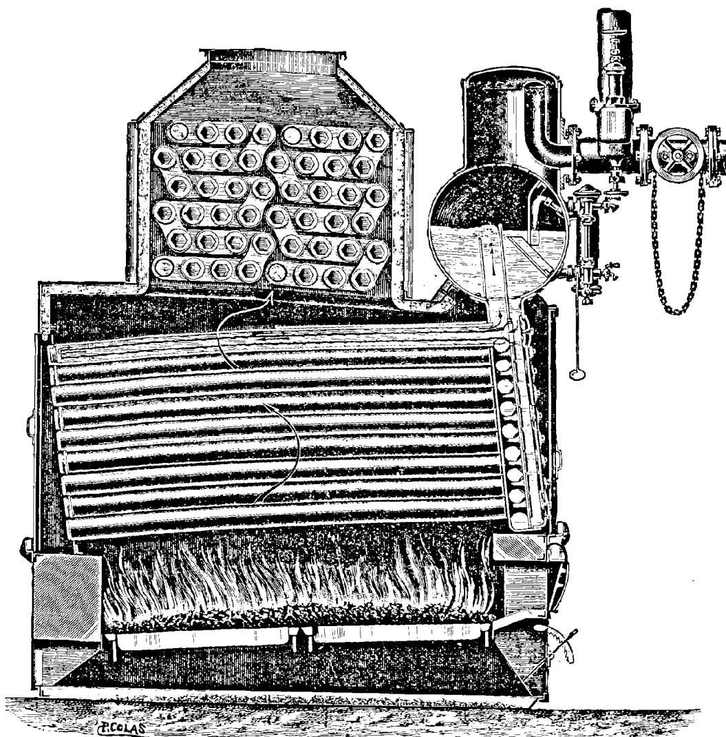
Fig. 52. — Chaudière Montupet, type Marine.
