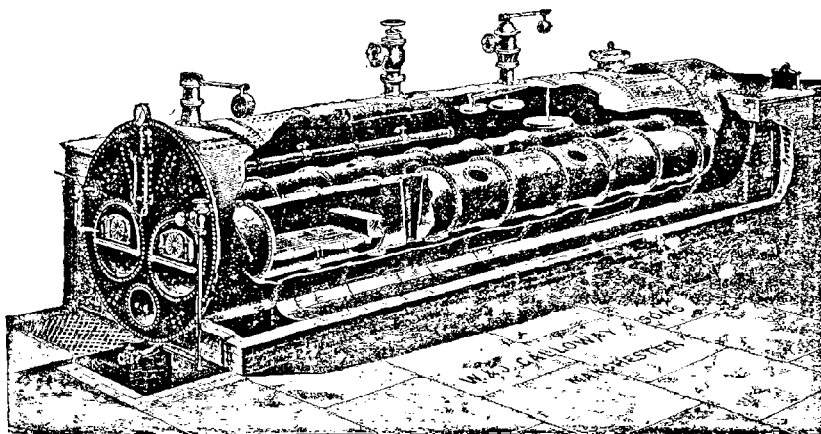
Fig. 44. — Chaudière à deux carneaux « Lancashire ».
