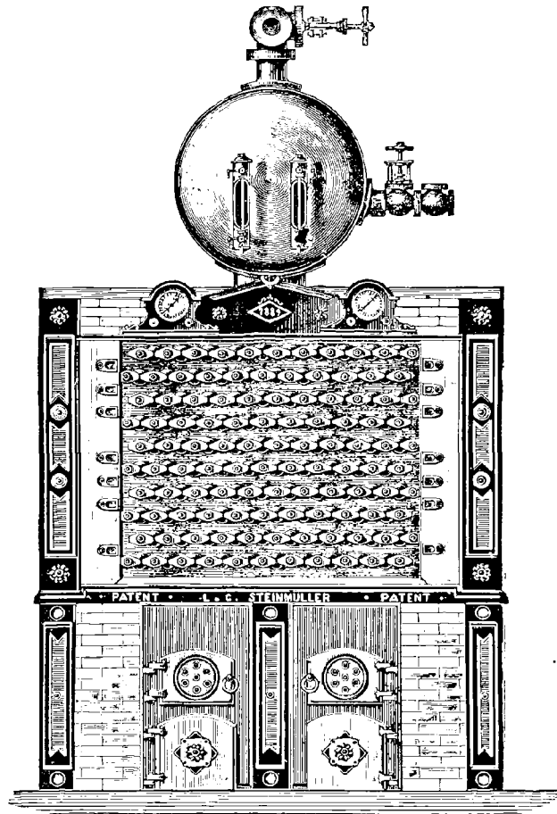
Fig. 82. — Vue de face d'un générateur Steinmüller.
