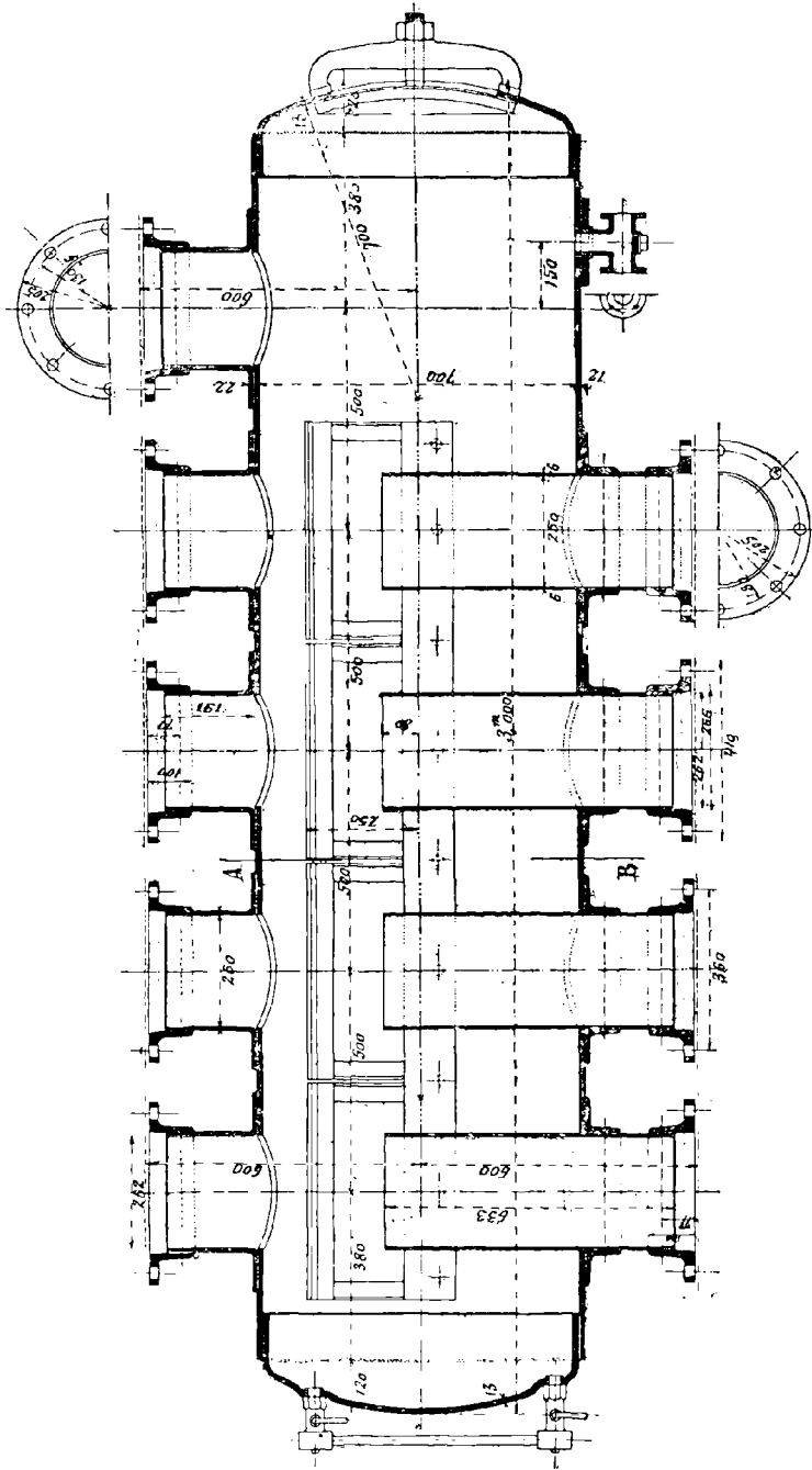
Fig. 89. — Collecteurs de vapeur. — Coupe longitudinale.
