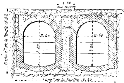
Fig. 42. — Coupe, type n° 4.
