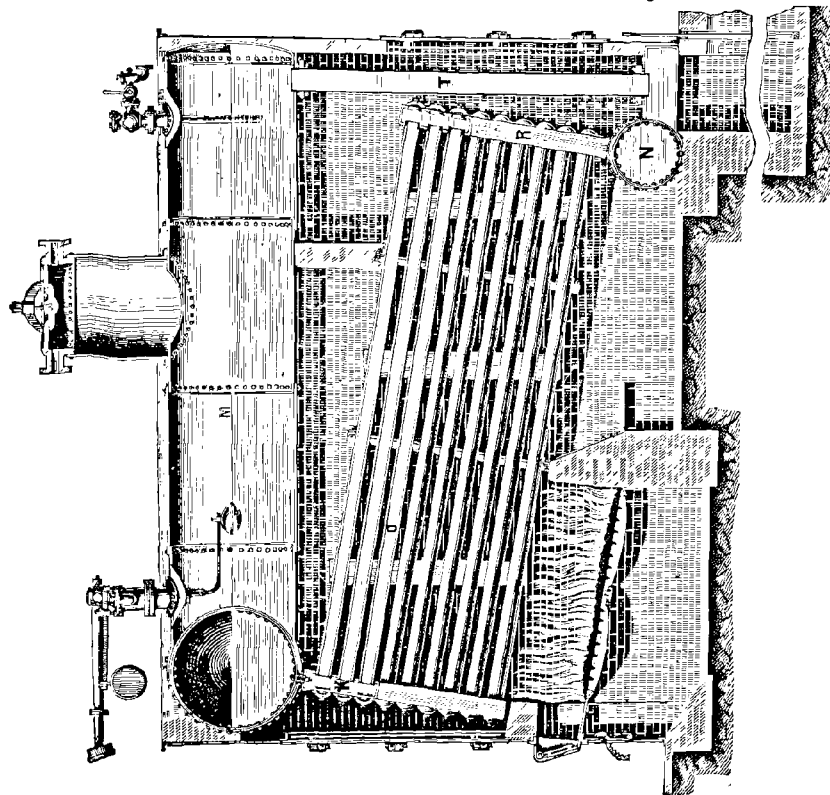
Fig. 69. — Coupe longitudinale.
