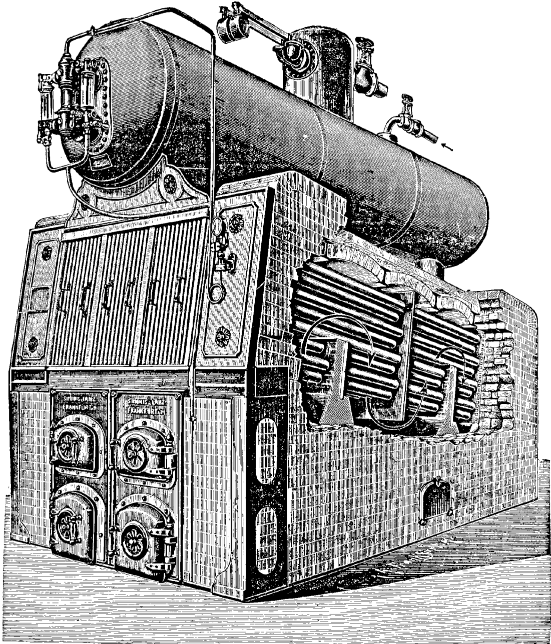
Fig. 77. — Chaudière Simonis et Lanz.
