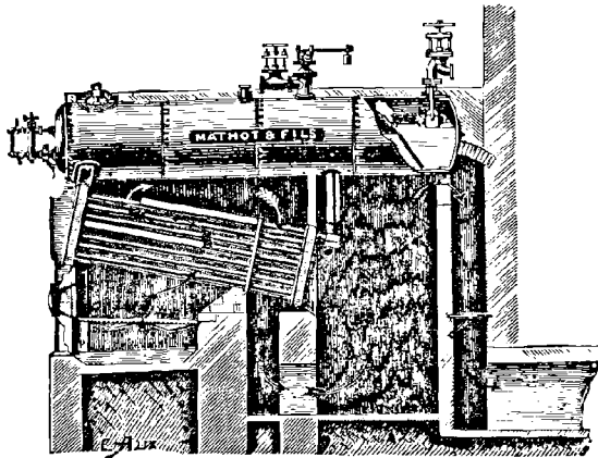
Fig. 45. — Générateur Mathot.
