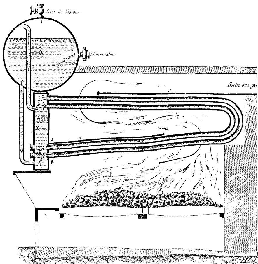
Fig. 74. — Schéma de la chaudière Solignac.
