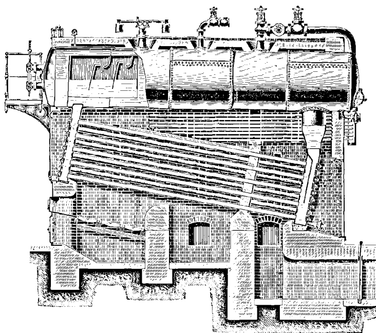
Fig. 65. — Chaudière multitubulaire Petry-Dereux.
