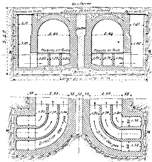
Fig. 14 et 15. — Branchements avec deux groupes de chaudières.
