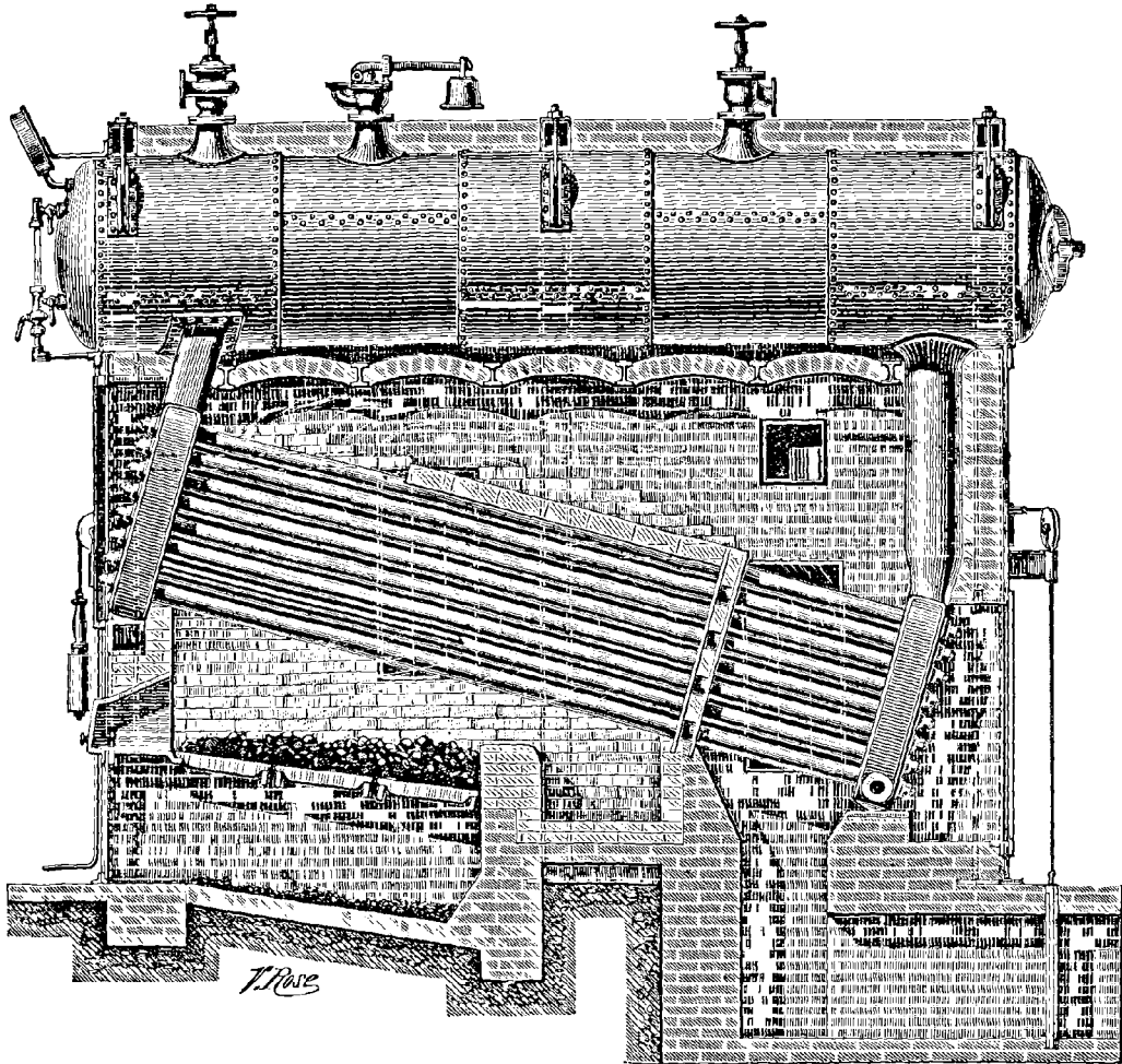
Fig. 139. — Chaudière multitubulaire, système Jacques Piedbœuf.
