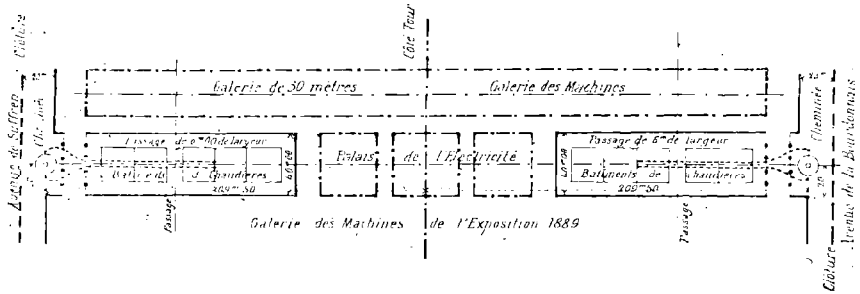
Fig. 16. — Plan d'ensemble pour l'emplacement des cheminées.
