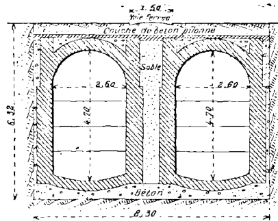
Fig. 43. — Coupe, type n° 5.
