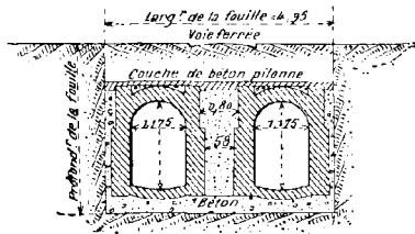
Fig. 9. — Coupe, type n° 1.
