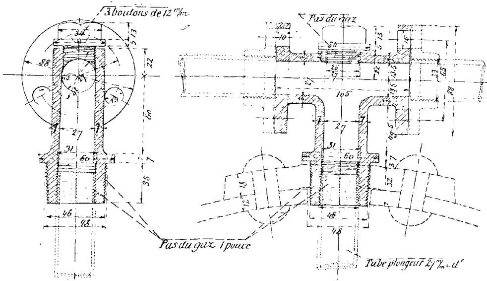
Fig. 88. — Détails de la bouteille de purge.
