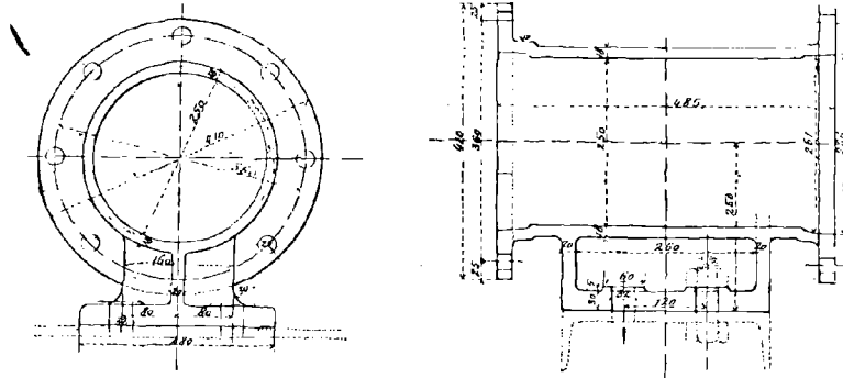
Fig. 91. — Mauchon point fixe.
