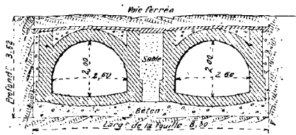
Fig. 10. — Coupe, type n° 2 bis.
