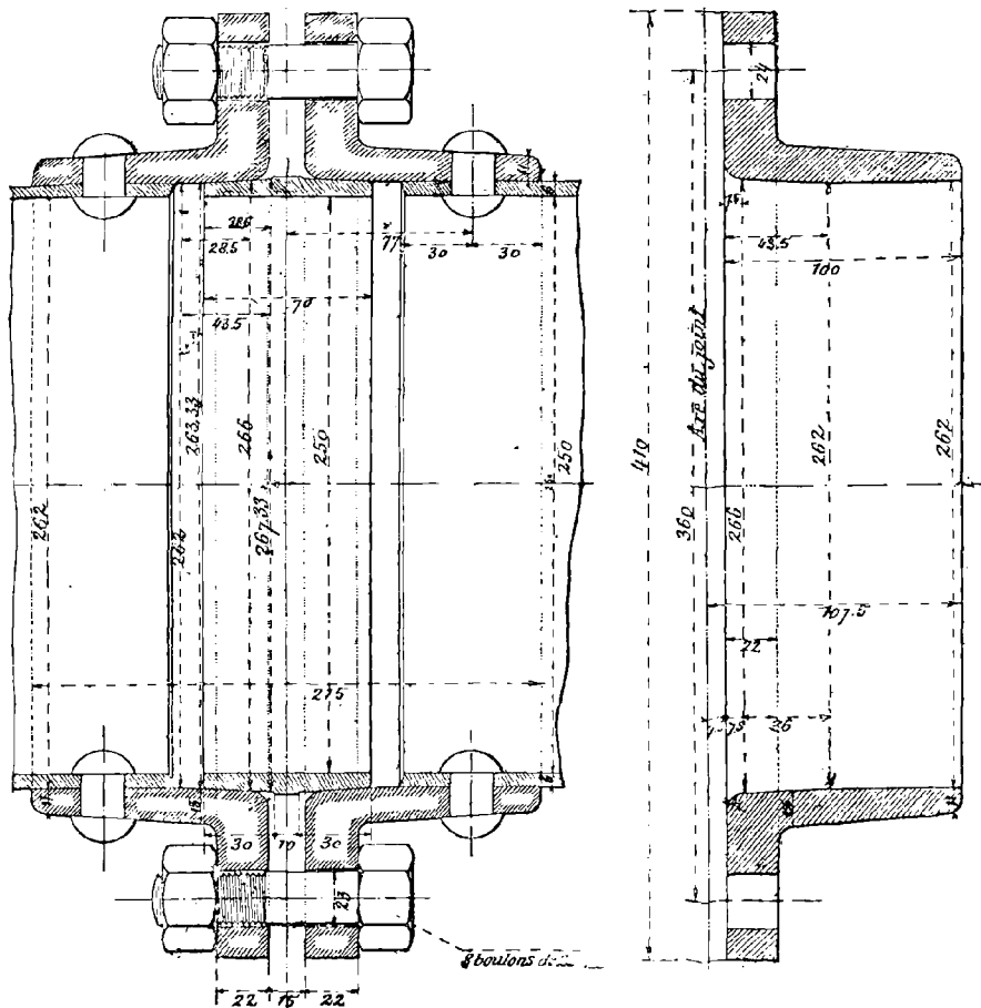
Fig. 83. — Joint biconique pour tuyaux de 0 m ,250.
