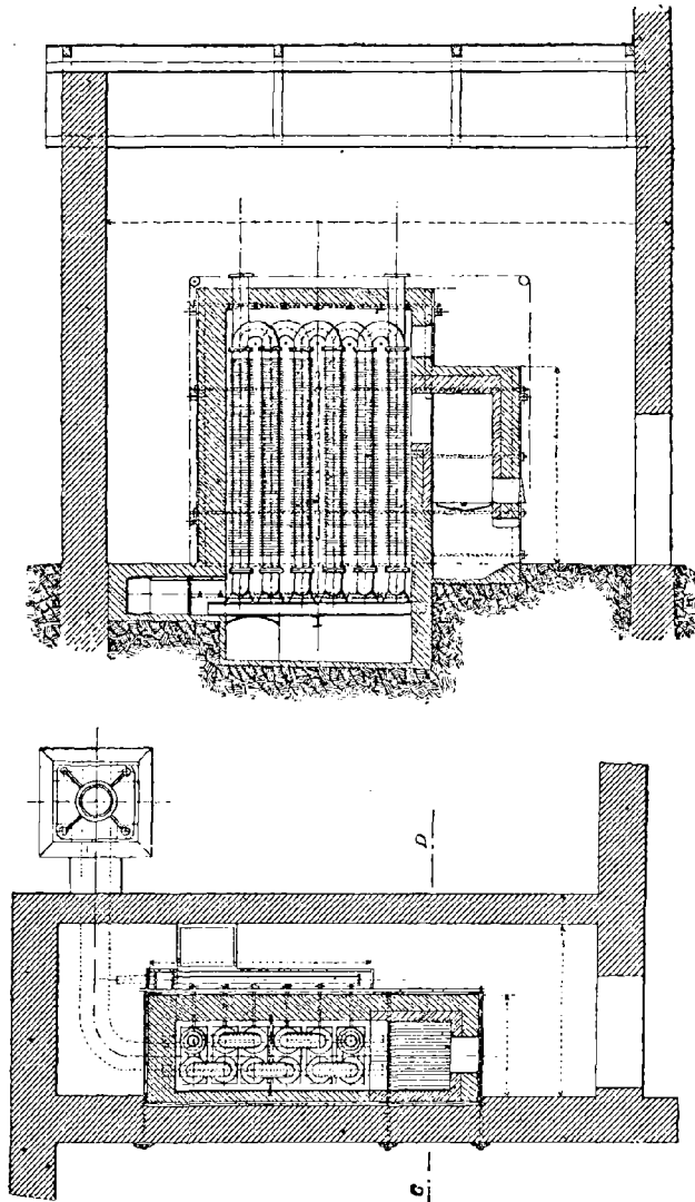
Fig. 147. — Surchauffeur Schwærer.
