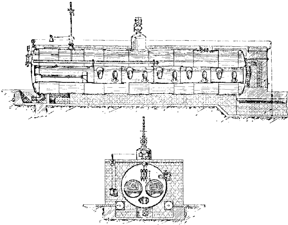
Fig. 133 et 136. — Chaudière Piedbœuf.
