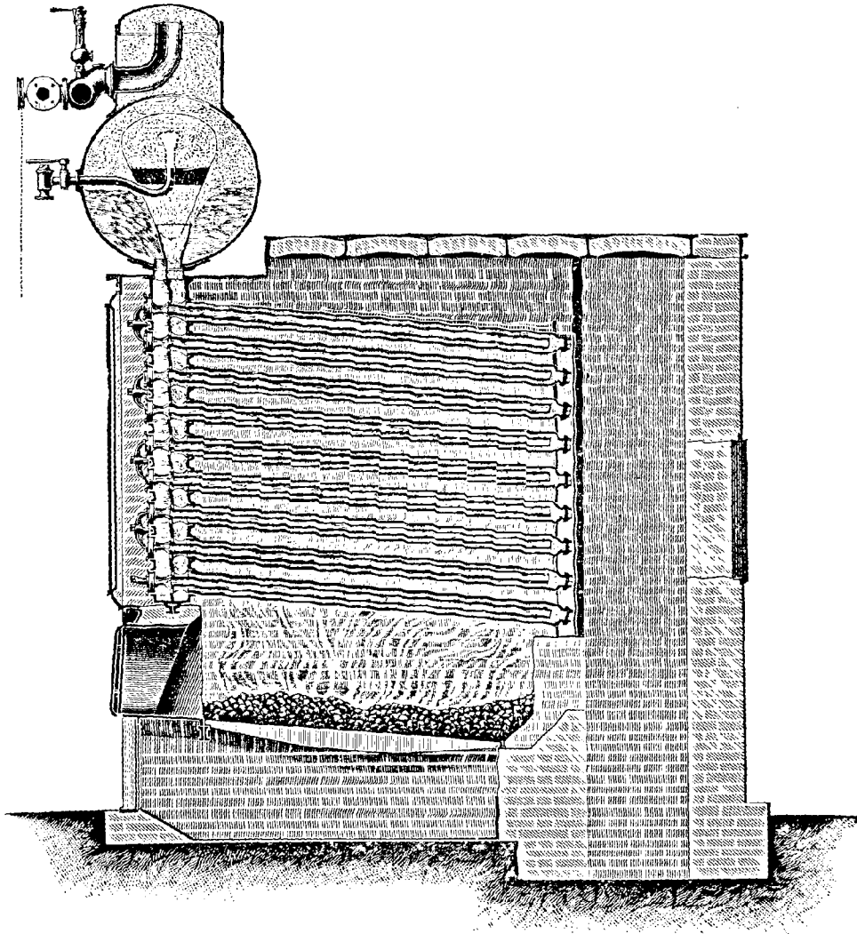
Fig. 58. — Générateur Nielsusse.
